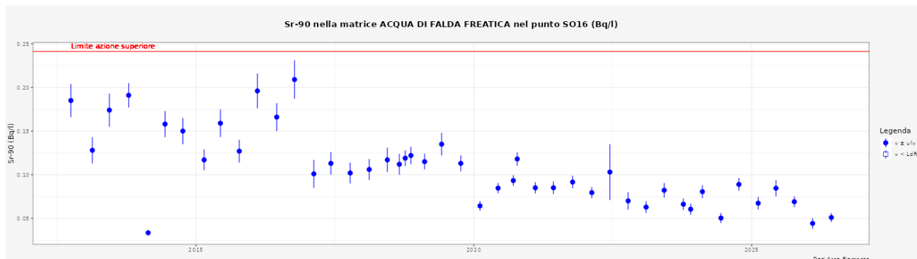
Figura 5.10. Andamento della concentrazione di Sr-90 nell'acqua di falda superficiale campionata nel punto A09 (Bq/l) – La linea rossa rappresenta il limite di azione pertinente.
