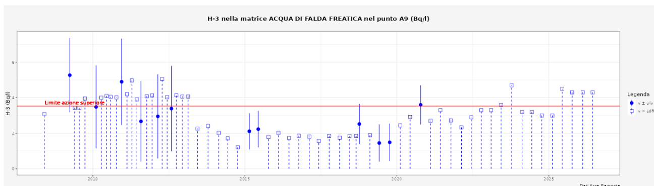
Figura 5.14. Andamento della concentrazione di H-3 nell'acqua di falda superficiale campionata nel punto A09 (Bq/l) – La linea rossa rappresenta il limite di azione pertinente.
