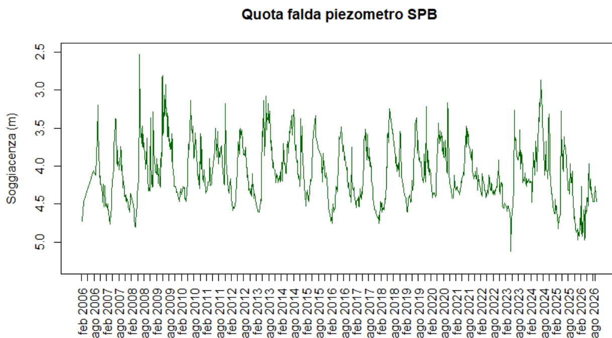
Figura 5.5. Andamento della soggiacenza della falda superficiale nel pozzo SPB espressa in metri rispetto al piano di campagna (Fonte: SO.G.I.N.).
