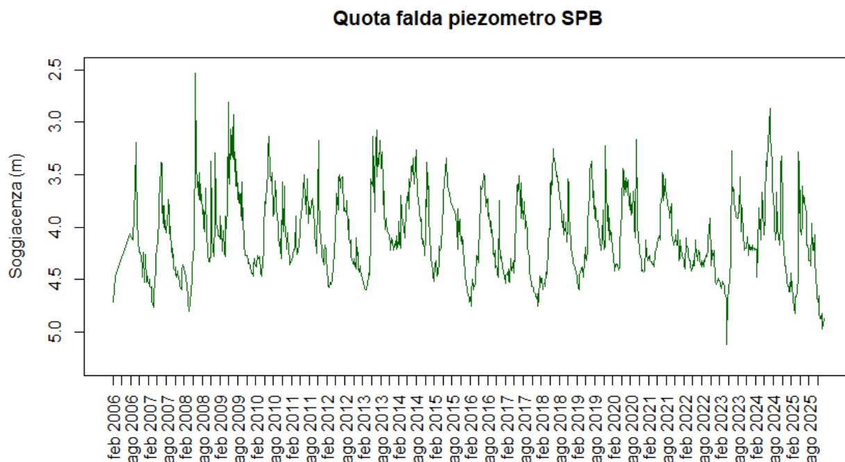
Figura 5.5. Andamento della soggiacenza della falda superficiale nel punto SPB (m.p.c.) (dati SO.G.I.N.).
