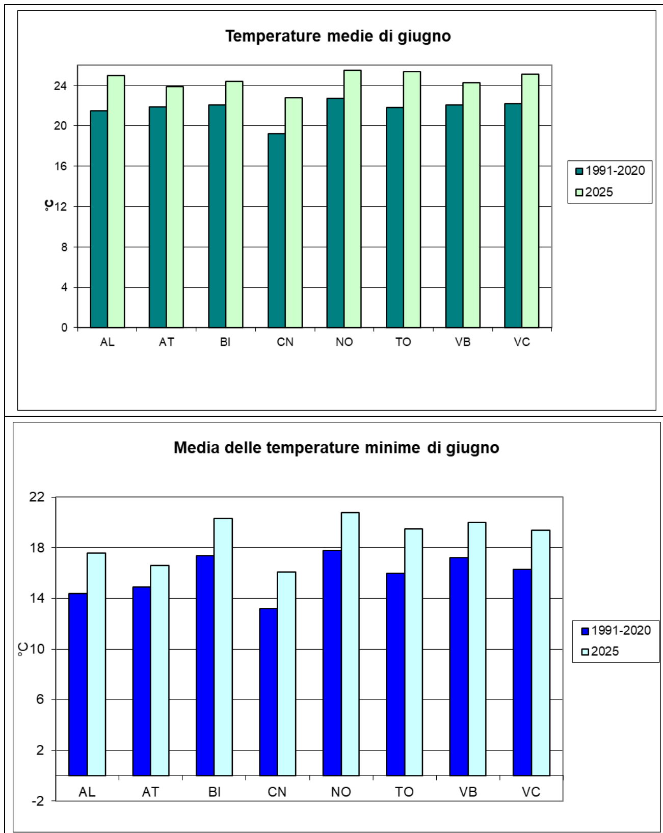
Figura 11 - Andamento della temperatura massima, media e minima mensile nei capoluoghi di provincia a giugno 2025 rispetto alla climatologia del periodo 1991-2020. Periodo di riferimento 2000-2020 per Biella, Novara e Verbania, fonte Arpa Piemonte.
