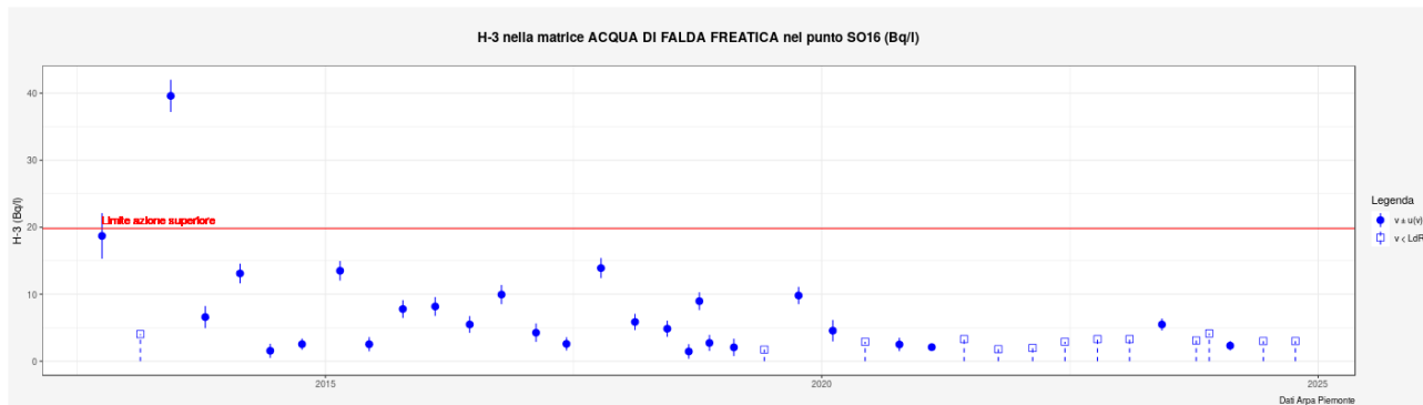
Figura 5.12. Andamento della concentrazione di attività di H-3 nell'acqua di falda superficiale campionata nel punto SO16 (Bq/l) – La linea rossa rappresenta il limite di azione pertinente.
