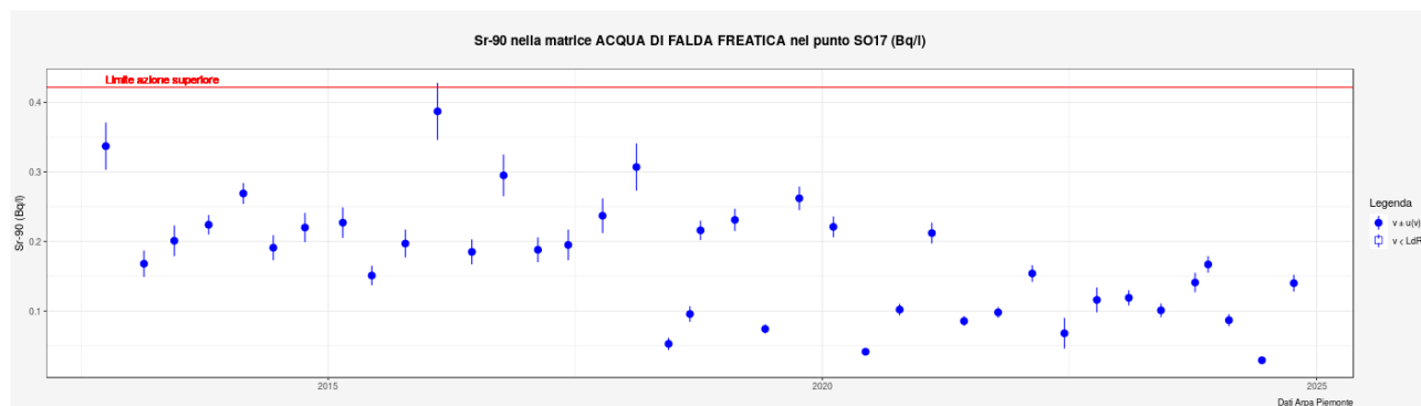
Figura 5.8. Andamento della concentrazione di attività di Sr-90 nell'acqua di falda superficiale campionata nel punto SO17 (Bq/l) – La linea rossa rappresenta il limite di azione pertinente.
