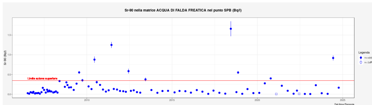
Figura 5.4. Andamento della concentrazione di attività di Sr-90 nell'acqua di falda superficiale campionata nel punto SPB (Bq/l) – La linea rossa rappresenta il limite di azione pertinente.
