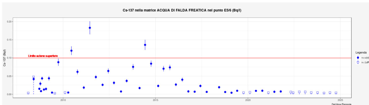
Figura 5.6. Andamento della concentrazione di attività di Cs-137 nell'acqua di falda superficiale campionata nel punto E5/6 (Bq/l) – La linea rossa rappresenta il limite di azione pertinente.
