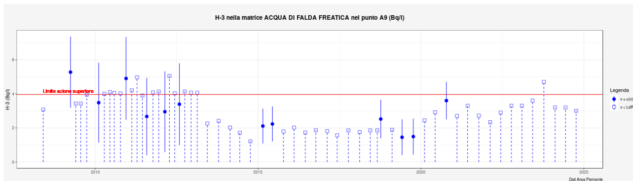
Figura 5.14. Andamento della concentrazione di attività di H-3 nell'acqua di falda superficiale campionata nel punto A9 (Bq/l) – La linea rossa rappresenta il limite di azione pertinente.
