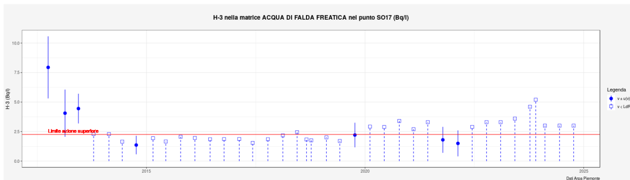
Figura 5.13. Andamento della concentrazione di attività di H-3 nell'acqua di falda superficiale campionata nel punto SO17 (Bq/l) – La linea rossa rappresenta il limite di azione pertinente.
