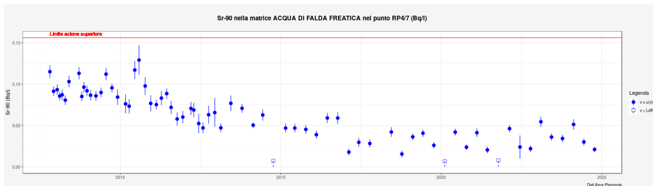
Figura 5.2. Andamento della concentrazione di attività di Sr-90 nell'acqua di falda superficiale campionata nel punto RP4/7 (Bq/l) – La linea rossa rappresenta il limite di azione pertinente.
