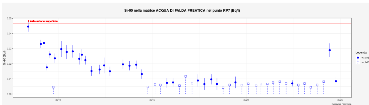
Figura 5.3. Andamento della concentrazione di attività di Sr-90 nell'acqua di falda superficiale campionata nel punto RP7 (Bq/l) – La linea rossa rappresenta il limite di azione pertinente.
