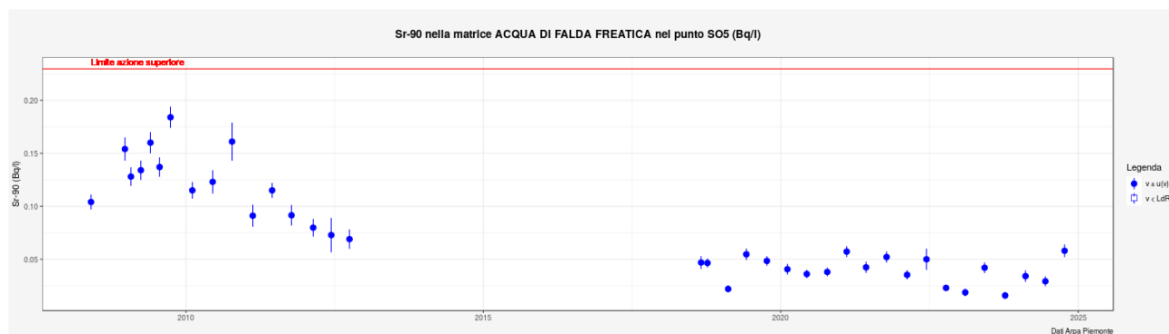
Figura 5.11. Andamento della concentrazione di attività di Sr-90 nell'acqua di falda superficiale campionata nel punto SO5 (Bq/l) – La linea rossa rappresenta il limite di azione pertinente.
