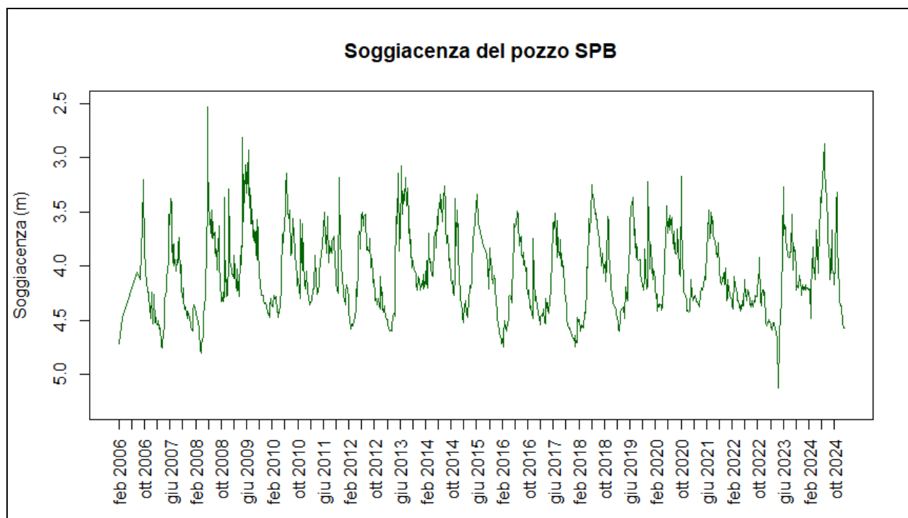
Figura 5.5. Andamento della soggiacenza della falda superficiale nel punto SPB (m.p.c.) (dati SO.G.I.N.).
