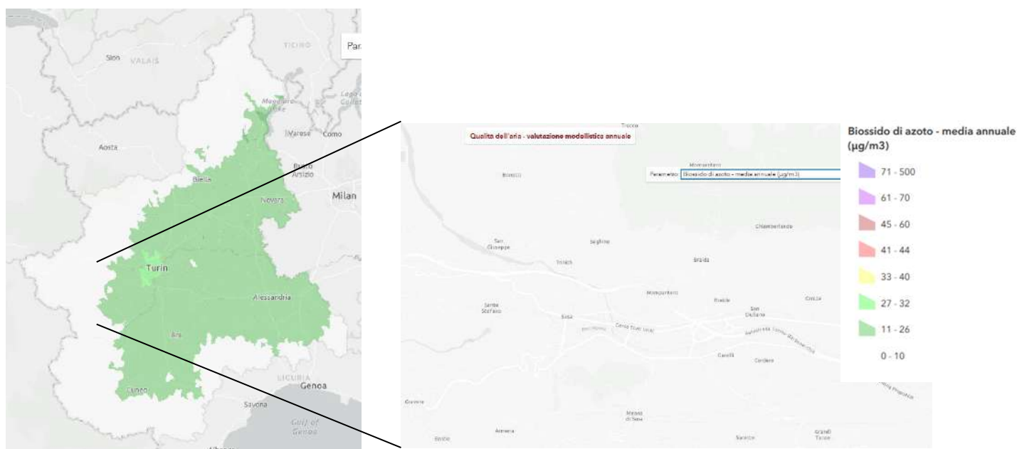
Figura 9: NO 2 - media annuale (µg/m 3 )
