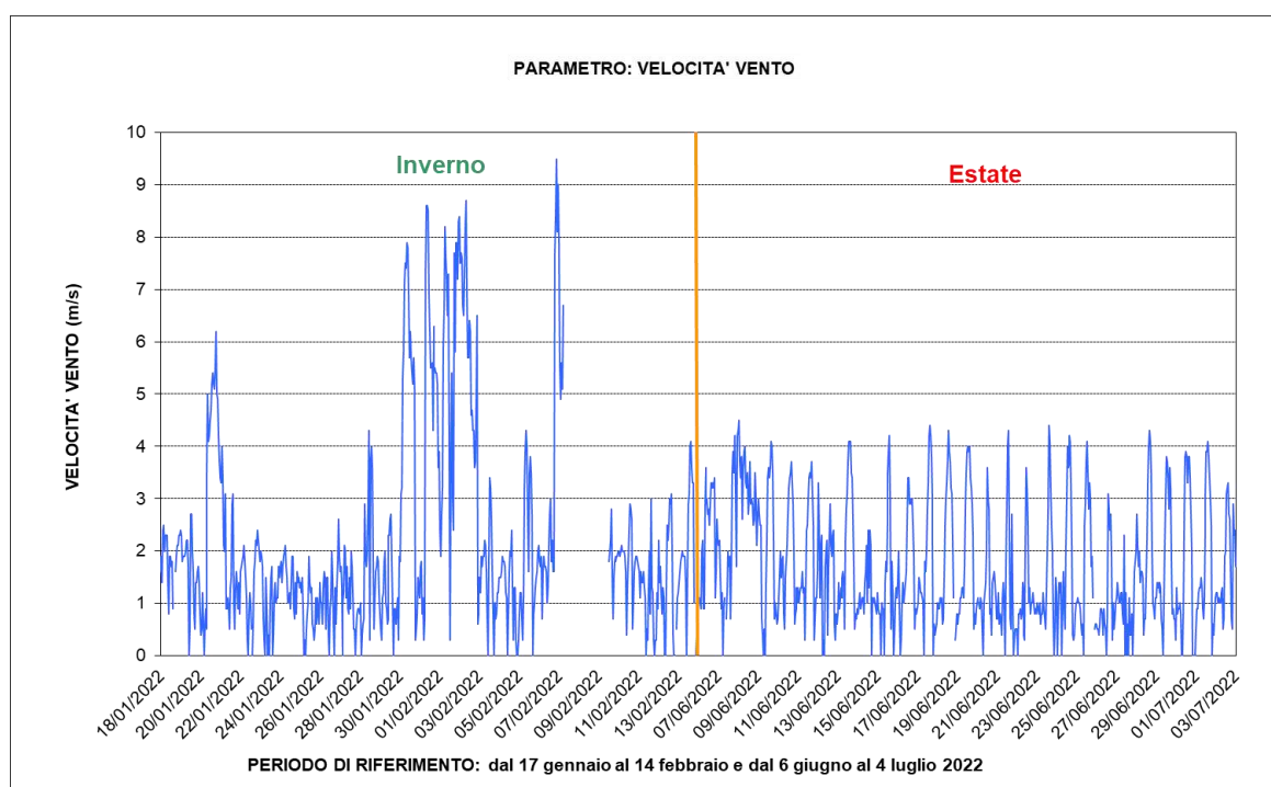
Figura 14: Velocità Vento
