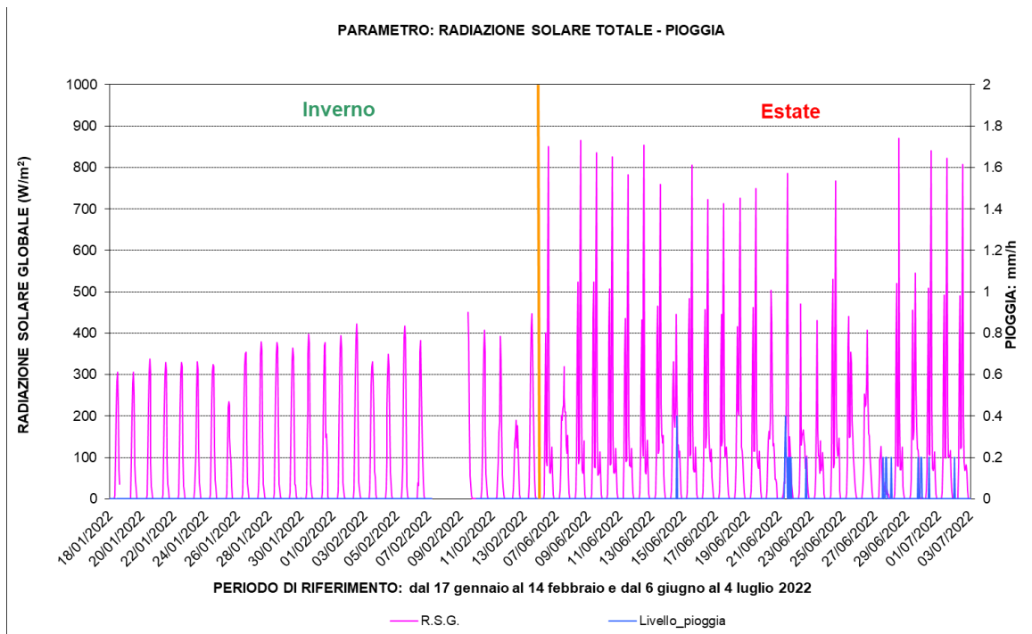
Figura 18: pioggia
