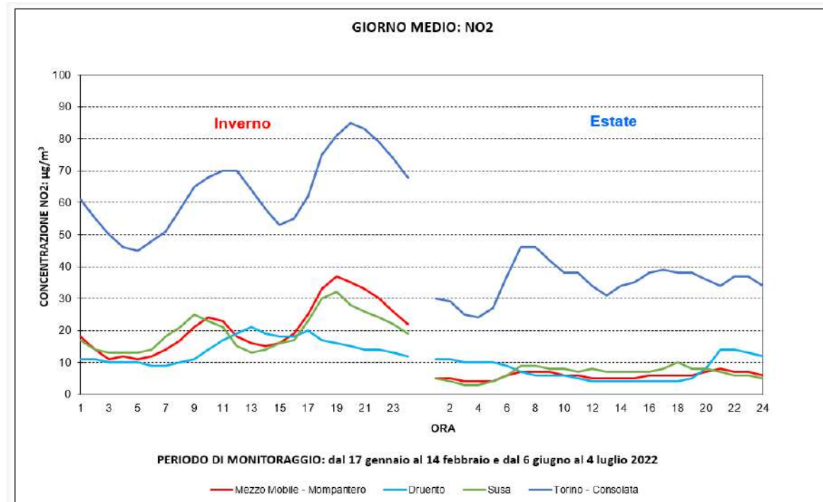
Figura 22: \text{NO}_2 - andamento del giorno medio
