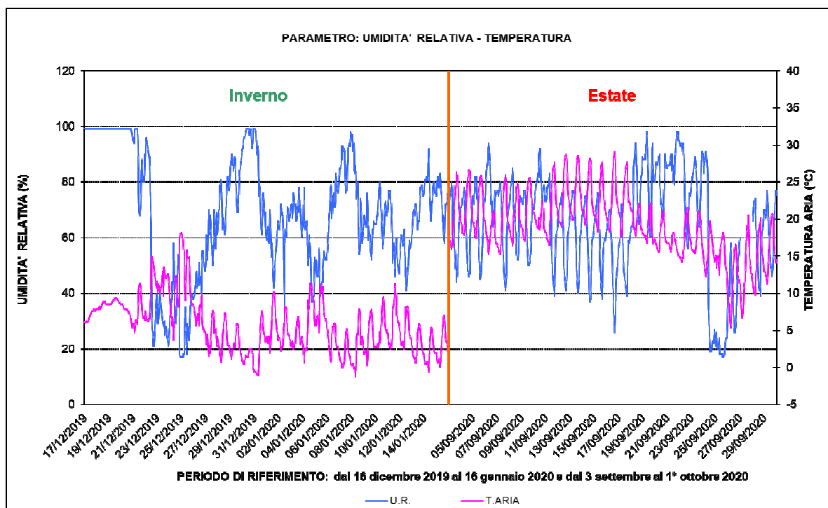
Figura 7: Umidità Relativa - Temperatura aria
