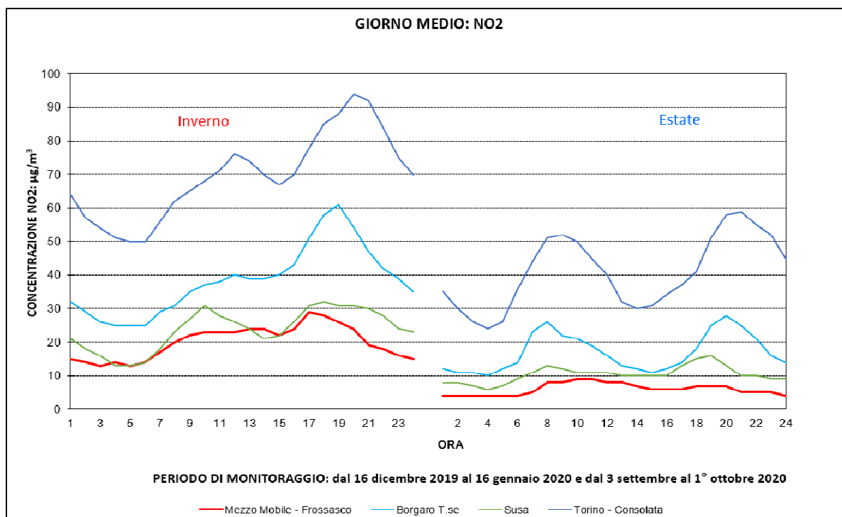
Figura 13: \text{NO}_2 - andamento del giorno medio
