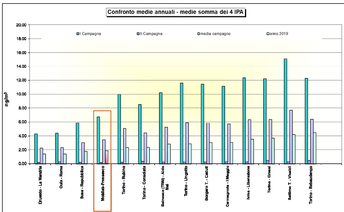
Figura 40: somma dei quattro IPA confronto della media delle campagne di monitoraggio con media anno 2019 nella Città Metropolitana di Torino
