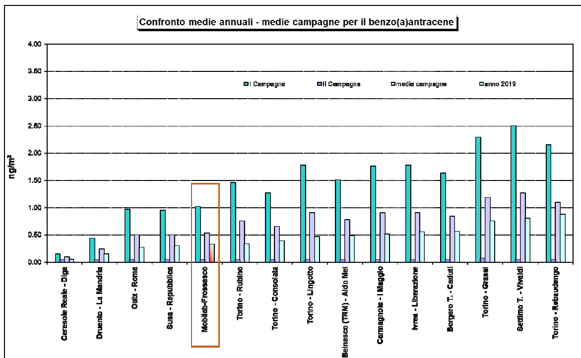
Figura 36: Benzo(a)antracene confronto della media delle campagne di monitoraggio con media anno 2019 nella Città Metropolitana di Torino
