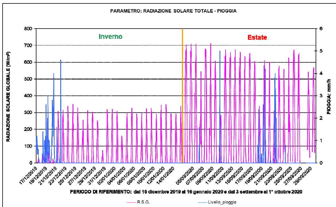
Figura 8: Radiazione Solare Globale e pioggia
