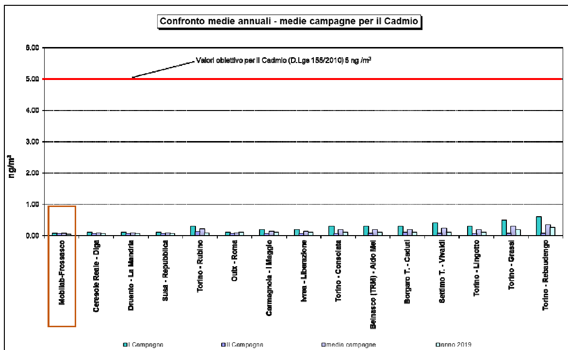
Figura 42: Cadmio confronto della media delle campagne di monitoraggio con media anno 2019 nella Città Metropolitana di Torino
