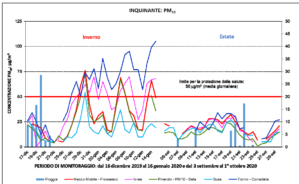
Figura 23: Particolato sospeso PM_{10} - confronto con il limite giornaliero per la protezione della salute e con i dati di alcune stazioni della rete fissa
