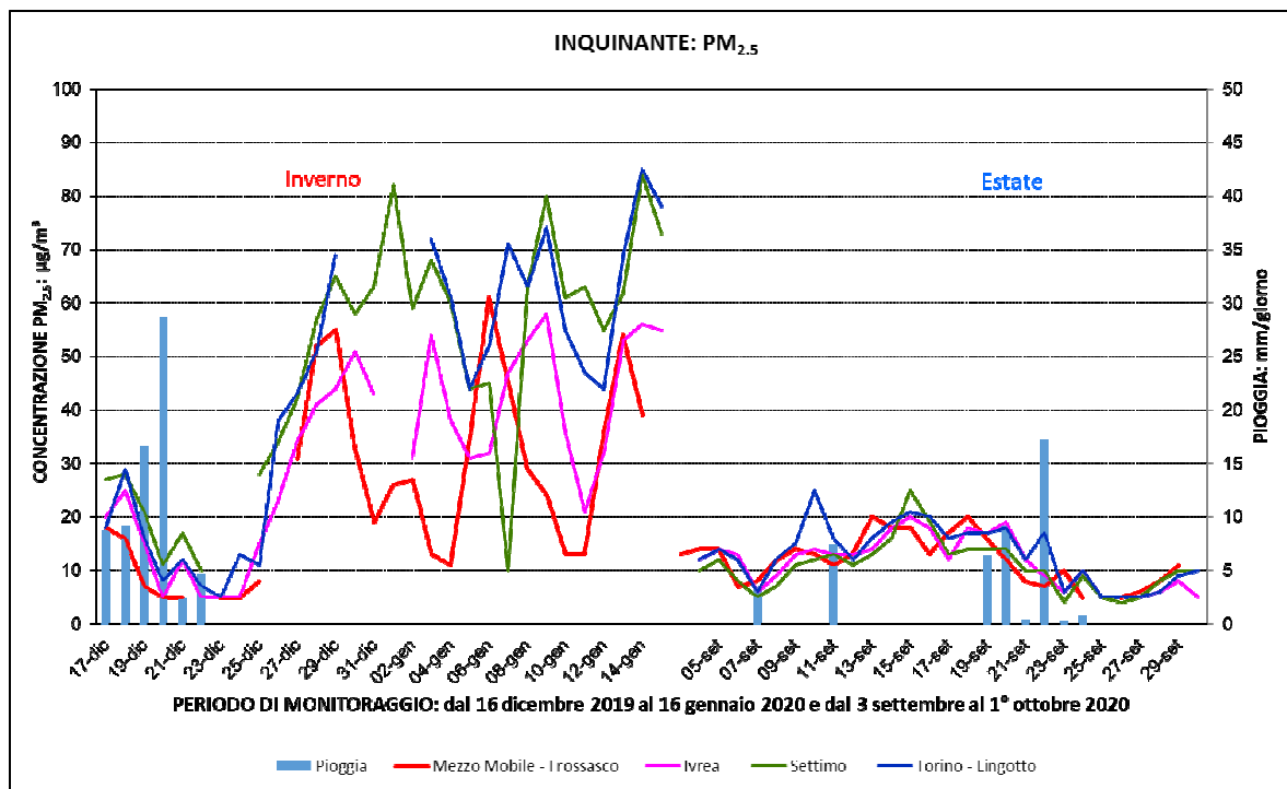
Figura 24: Particolato sospeso PM_{2.5} - confronto con i dati di alcune stazioni della rete fissa
