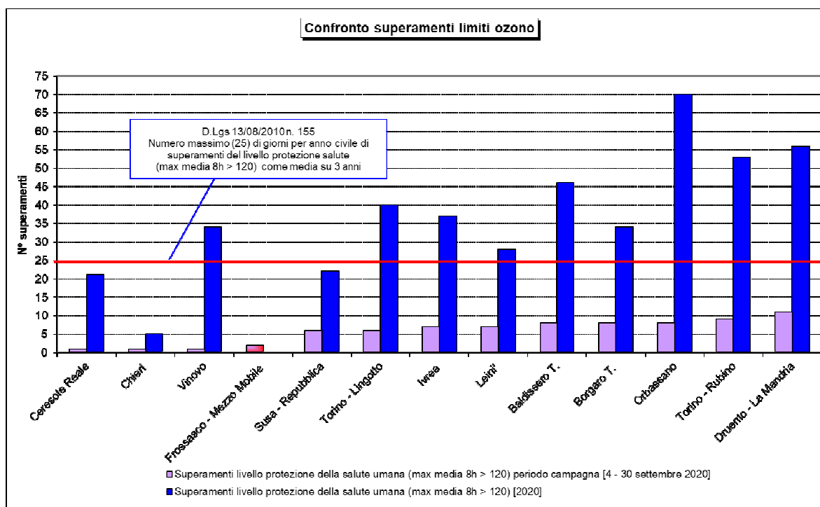
Figura 34: confronto superamenti livelli protezione della salute umana – periodo 2 a campagna 2020
