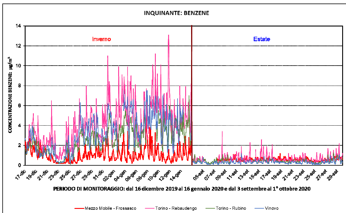
Figura 20: Benzene - andamento orario e confronto con i dati delle stazioni di Torino – Rebaudengo, Torino – Rubino T. e Vinovo
