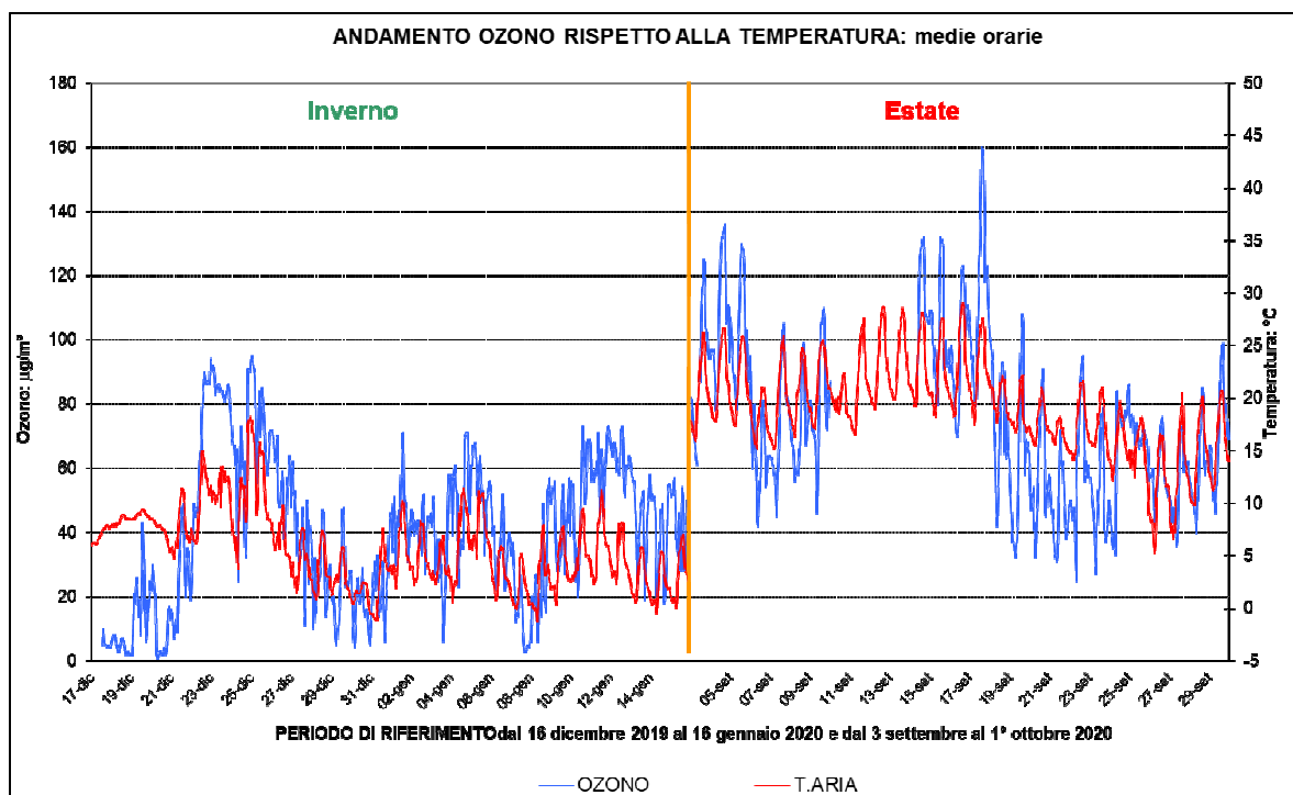
Figura 32: O_3 - andamento della concentrazione oraria e confronto con temperatura
