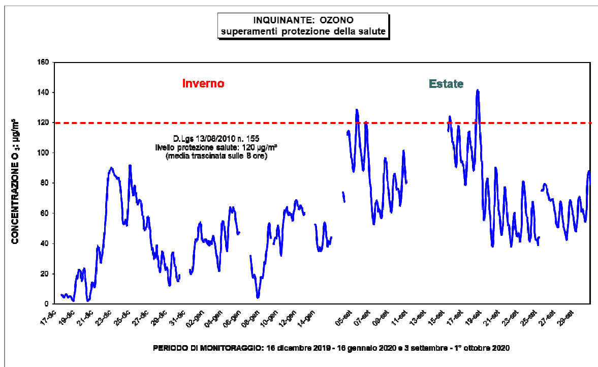
Figura 29: O_3 - superamenti protezione della salute umana
