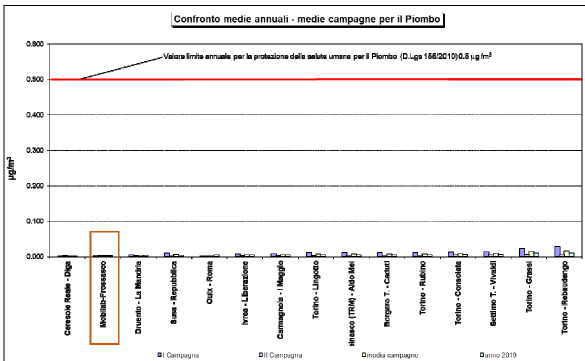
Figura 44: Piombo confronto della media delle campagne di monitoraggio con media anno 2019 nella Città Metropolitana di Torino
