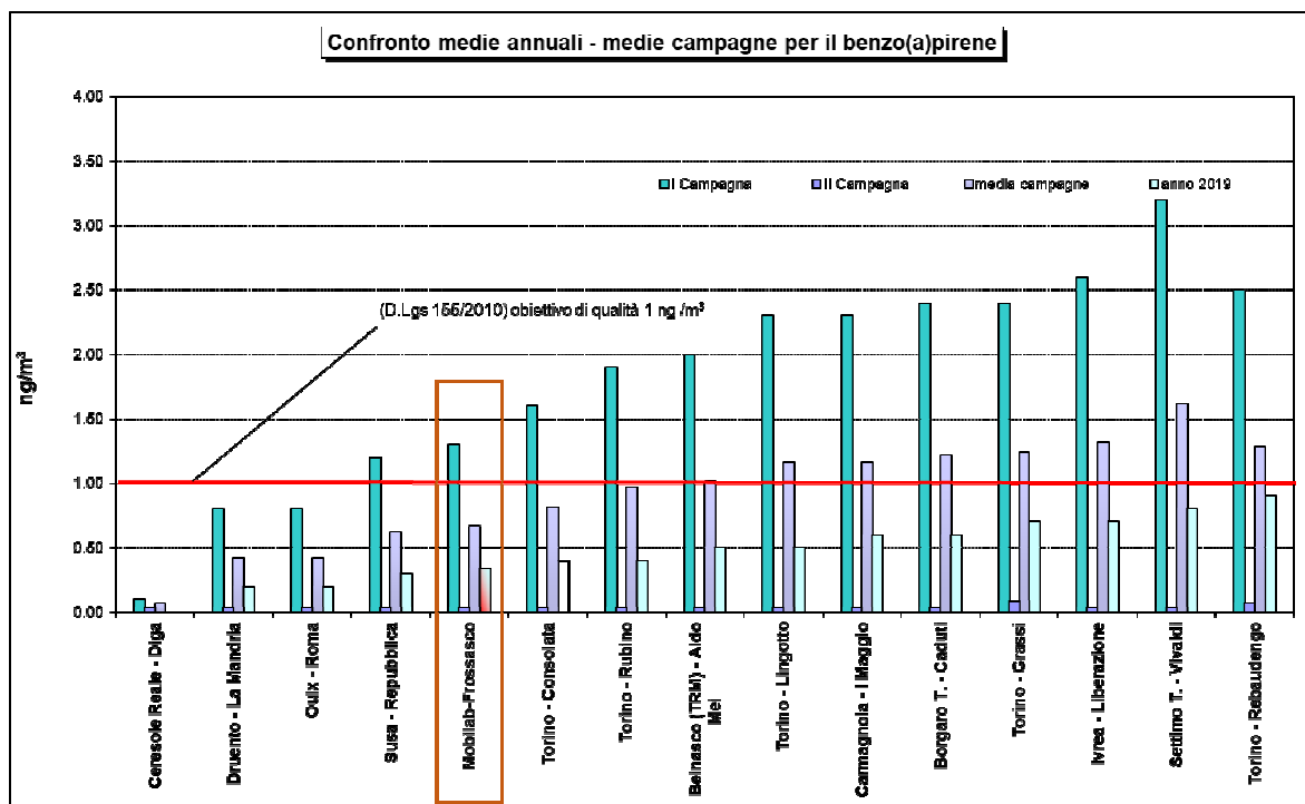
Figura 38: Benzo(a)pirene confronto della media delle campagne di monitoraggio con media anno 2019 nella Città Metropolitana di Torino
