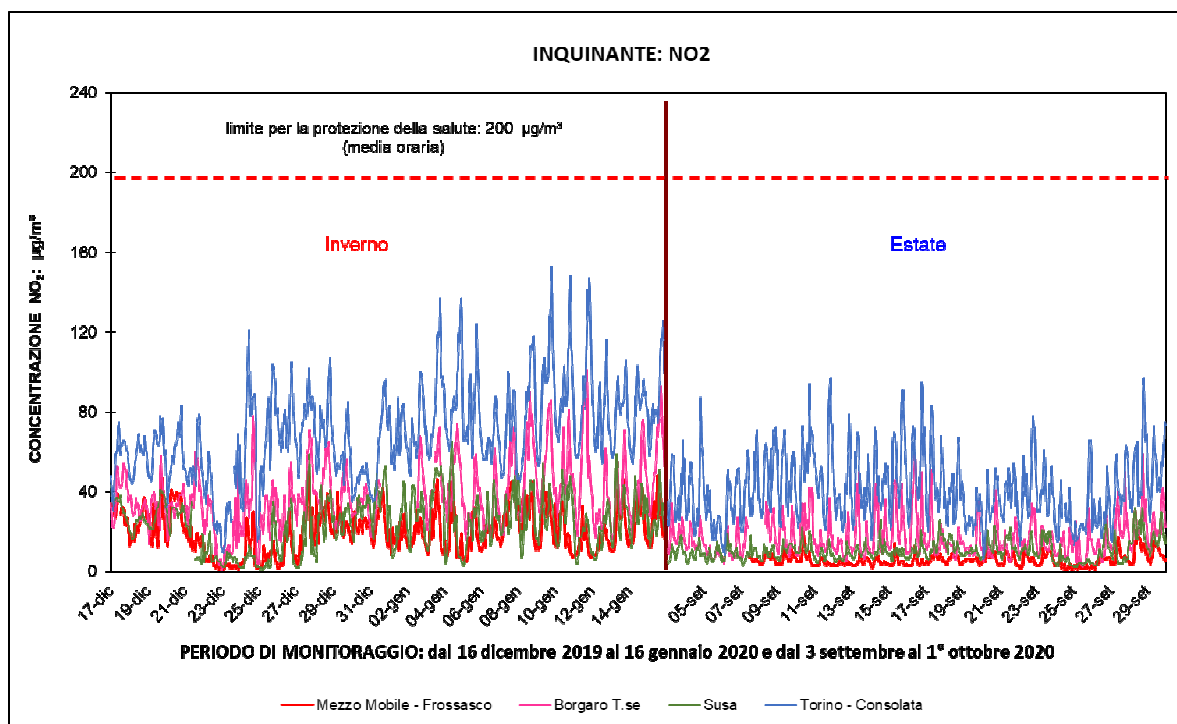
Figura 12: \text{NO}_2 - confronto con i limiti di legge e con i dati delle stazioni fisse di Borgaro, Susa e Torino-Consolata
