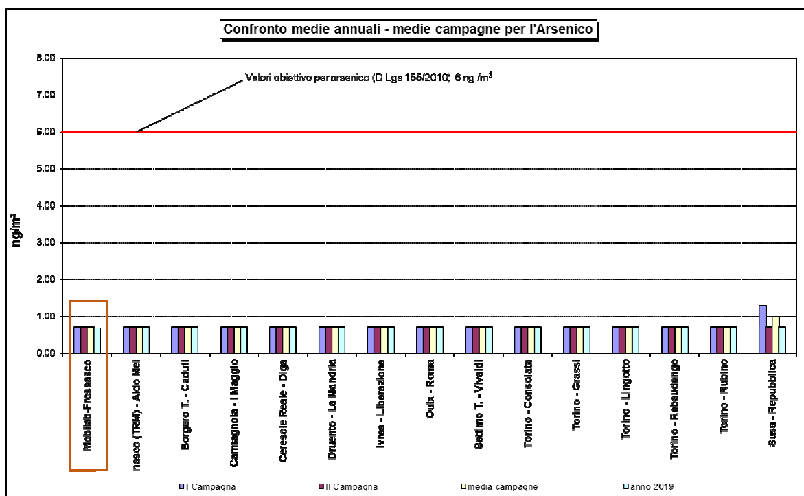
Figura 41: Arsenico confronto della media delle campagne di monitoraggio con media anno 2019 nella Città Metropolitana di Torino
