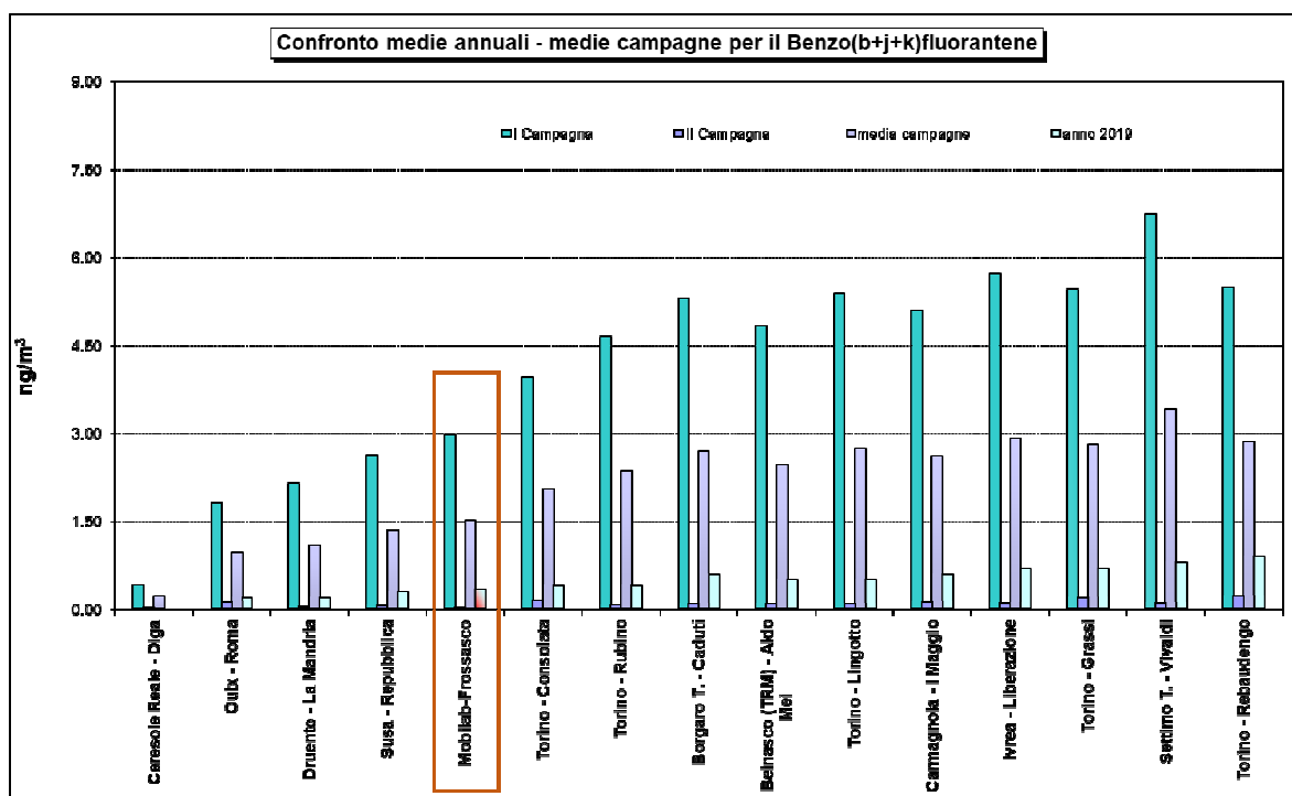
Figura 37: Benzo(b+j+k)fluorantene confronto della media delle campagne di monitoraggio con media anno 2019 nella Città Metropolitana di Torino
