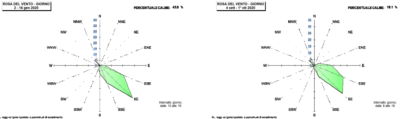
Figura 4: Distribuzione dati di vento in funzione della direzione e della classe di velocità – diurna
