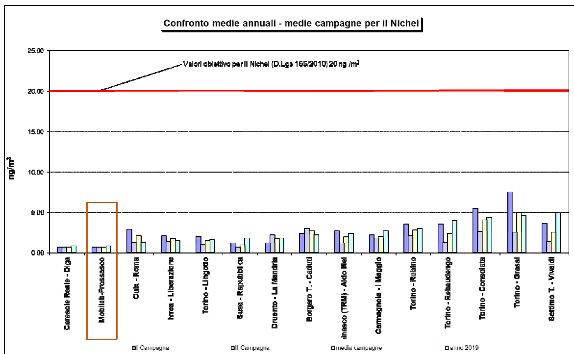
Figura 43: Nichel confronto della media delle campagne di monitoraggio con media anno 2019 nella Città Metropolitana di Torino
