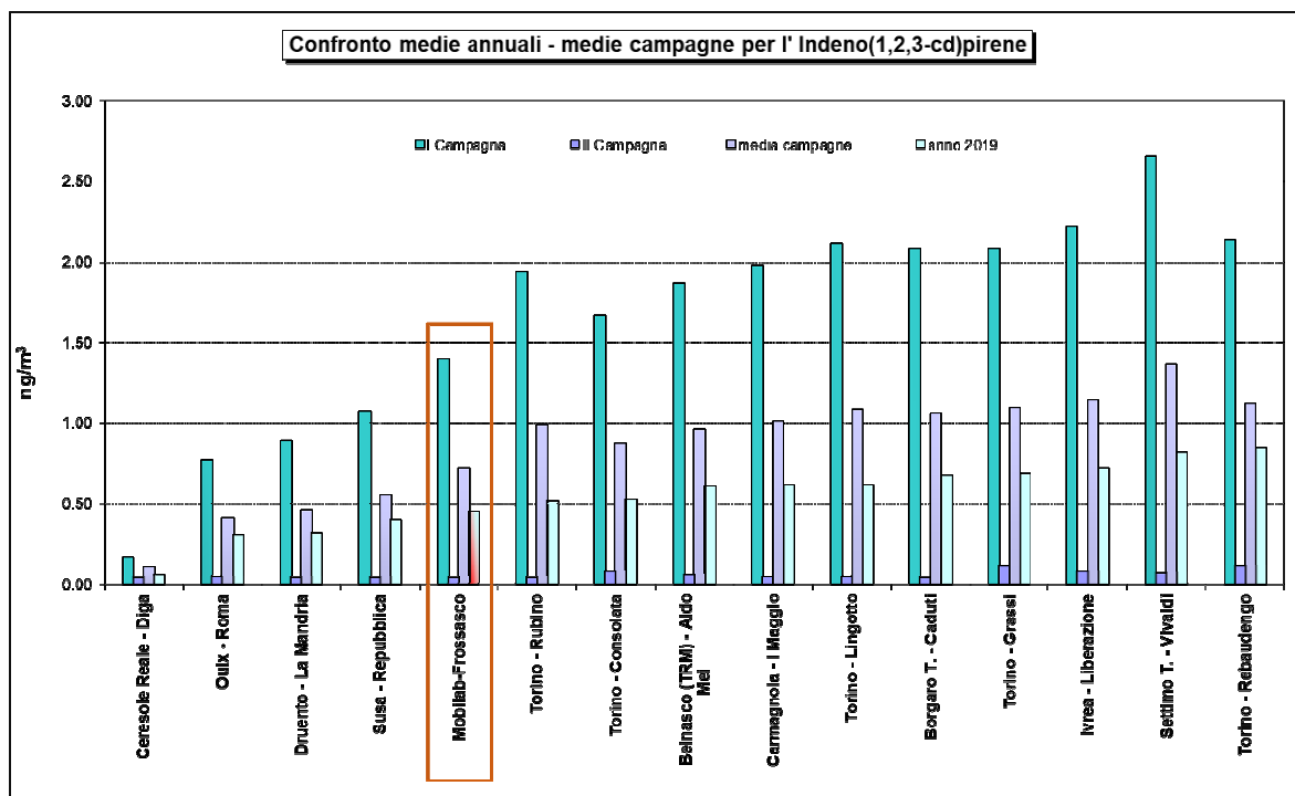
Figura 39: Indeno(1, 2, 3-cd)pirene confronto della media delle campagne di monitoraggio con media anno 2019 nella Città Metropolitana di Torino
