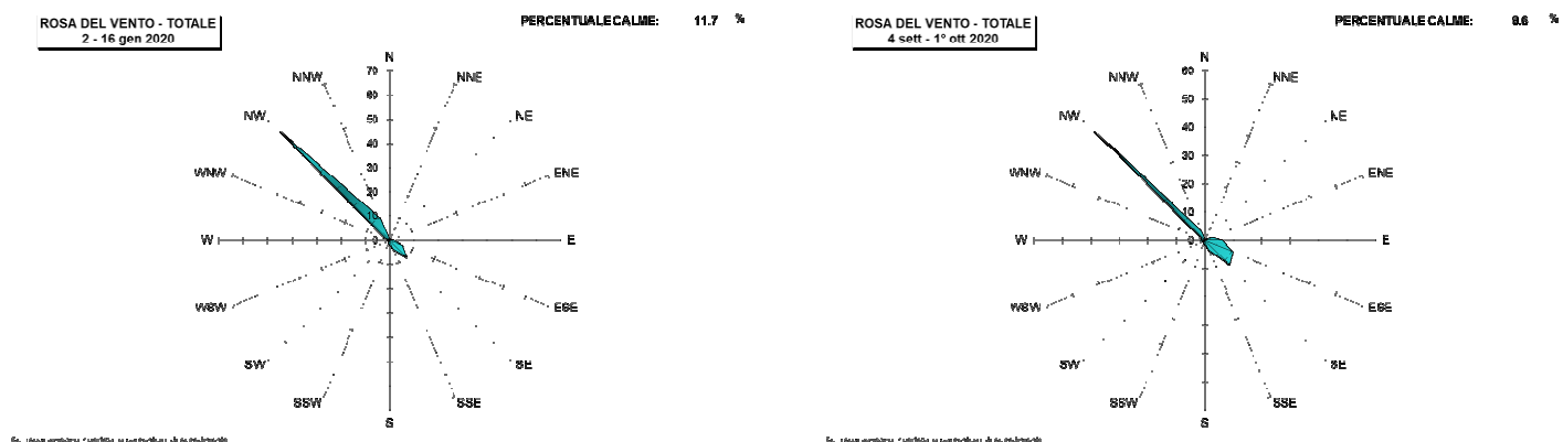
Figura 3: Distribuzione dati di vento in funzione della direzione e della classe di velocità – totale
