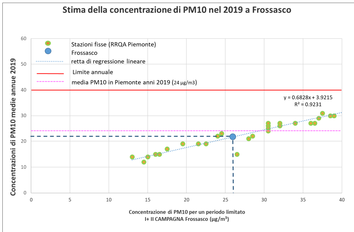
Figura 26: Particolato sospeso PM_{10} - stima della concentrazione annuale a Frossasco
