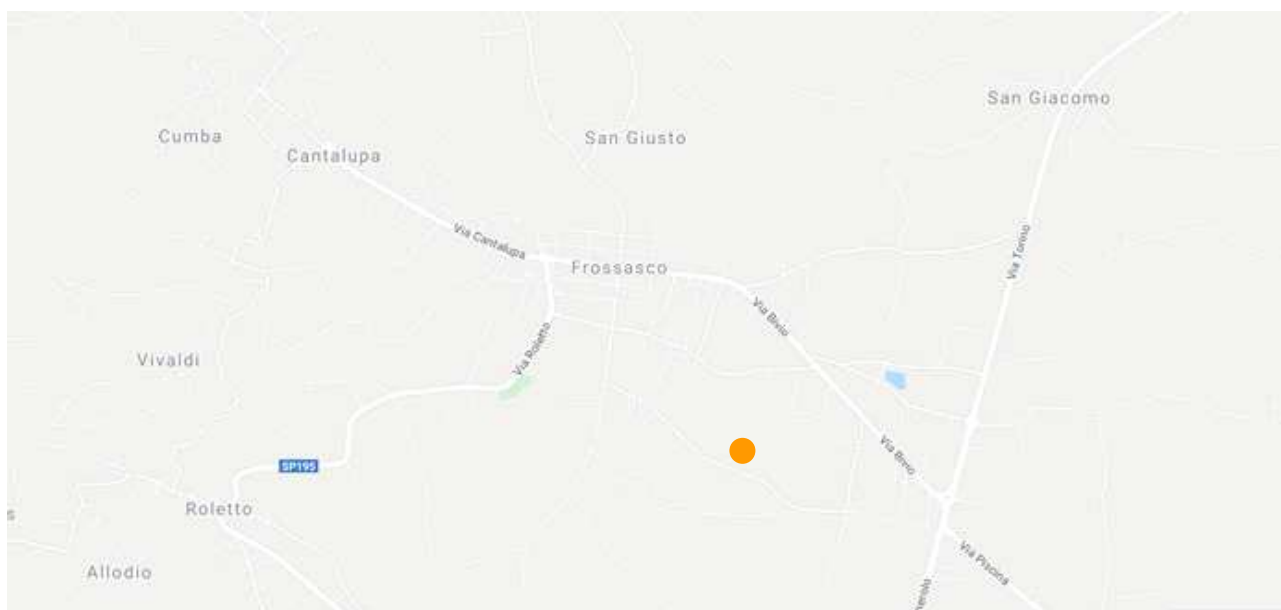
Figura 1: Ubicazione del Laboratorio Mobile per il monitoraggio della qualità dell'aria nel comune di Frossasco.
