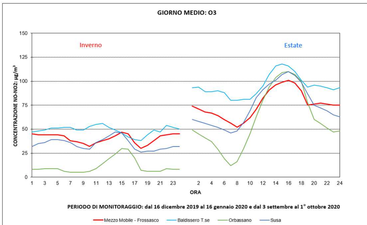
Figura 30: Ozono giorno medio
