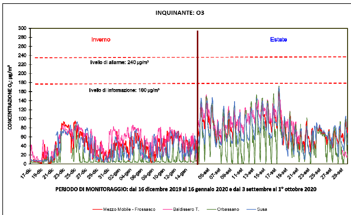
Figura 28: O_3 - confronto con i limiti di legge
