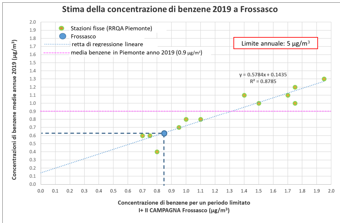
Figura 22: Benzene - stima della concentrazione annuale a Frossasco
