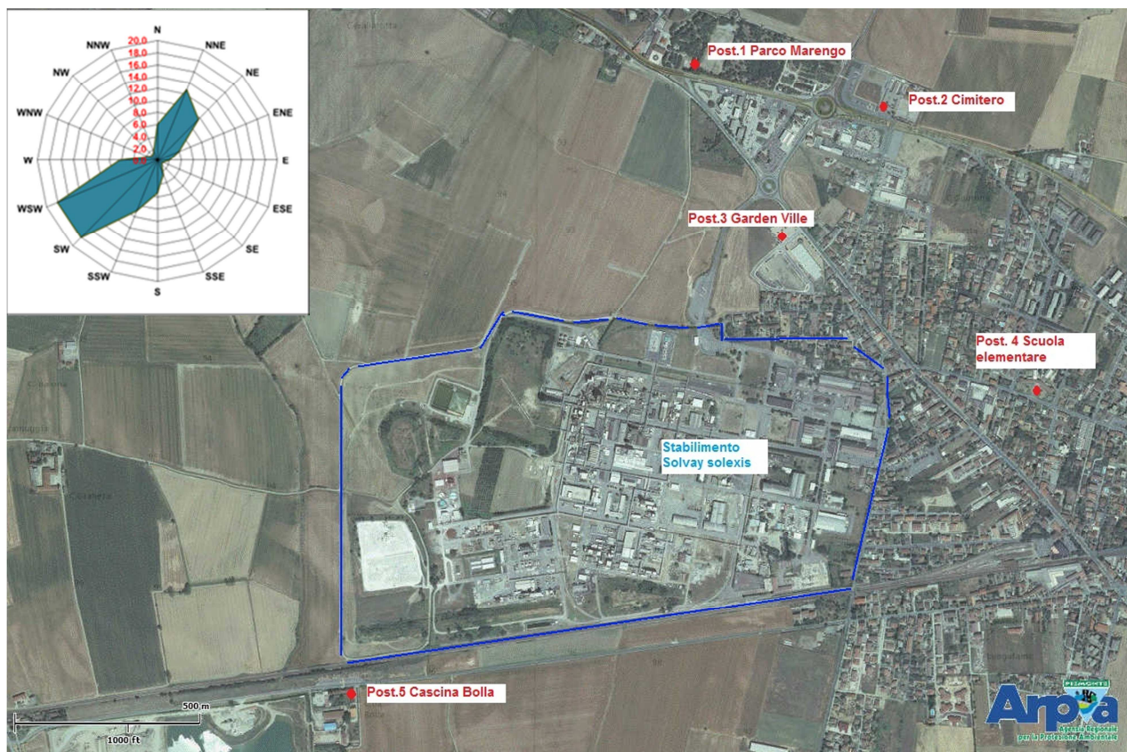
Punti di campionamento di HCl e HF effettuati dal 2010 al 2012 a Spinetta M.go e direzioni prevalenti del vento registrate dalla stazione meteo regionale di Alessandria Lobbì.
