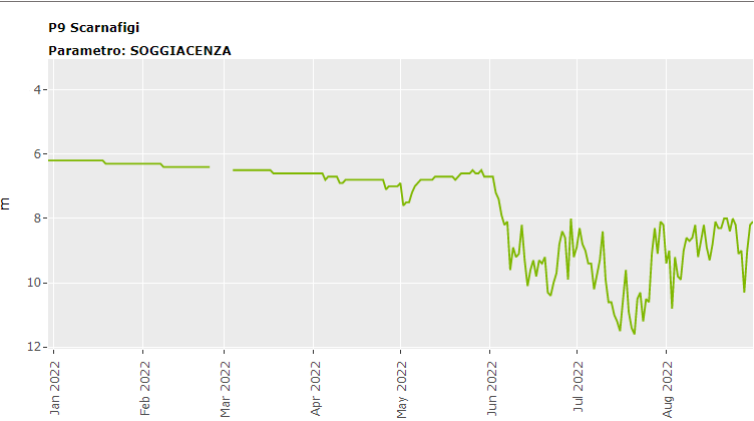
Grafico della soggiacenza dell'anno 2022 aggiornato al 31/08
