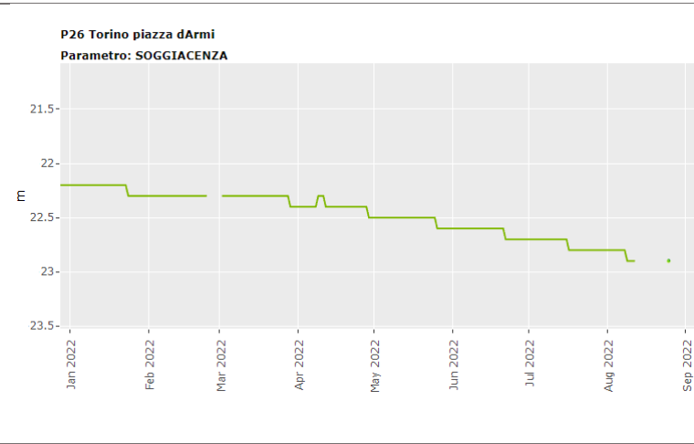
Grafico della soggiacenza dell'anno 2022 aggiornato al 26/08
