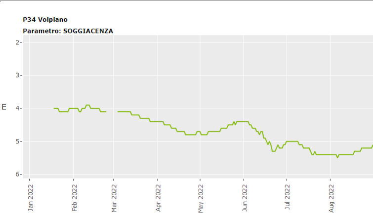
Grafico della soggiacenza dell'anno 2022 aggiornato al 31/08
