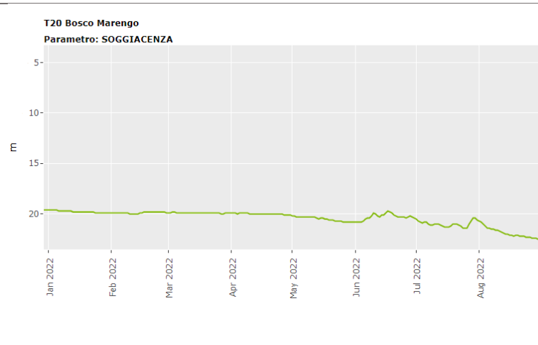
Grafico della soggiacenza dell'anno 2022 aggiornato al 31/08
