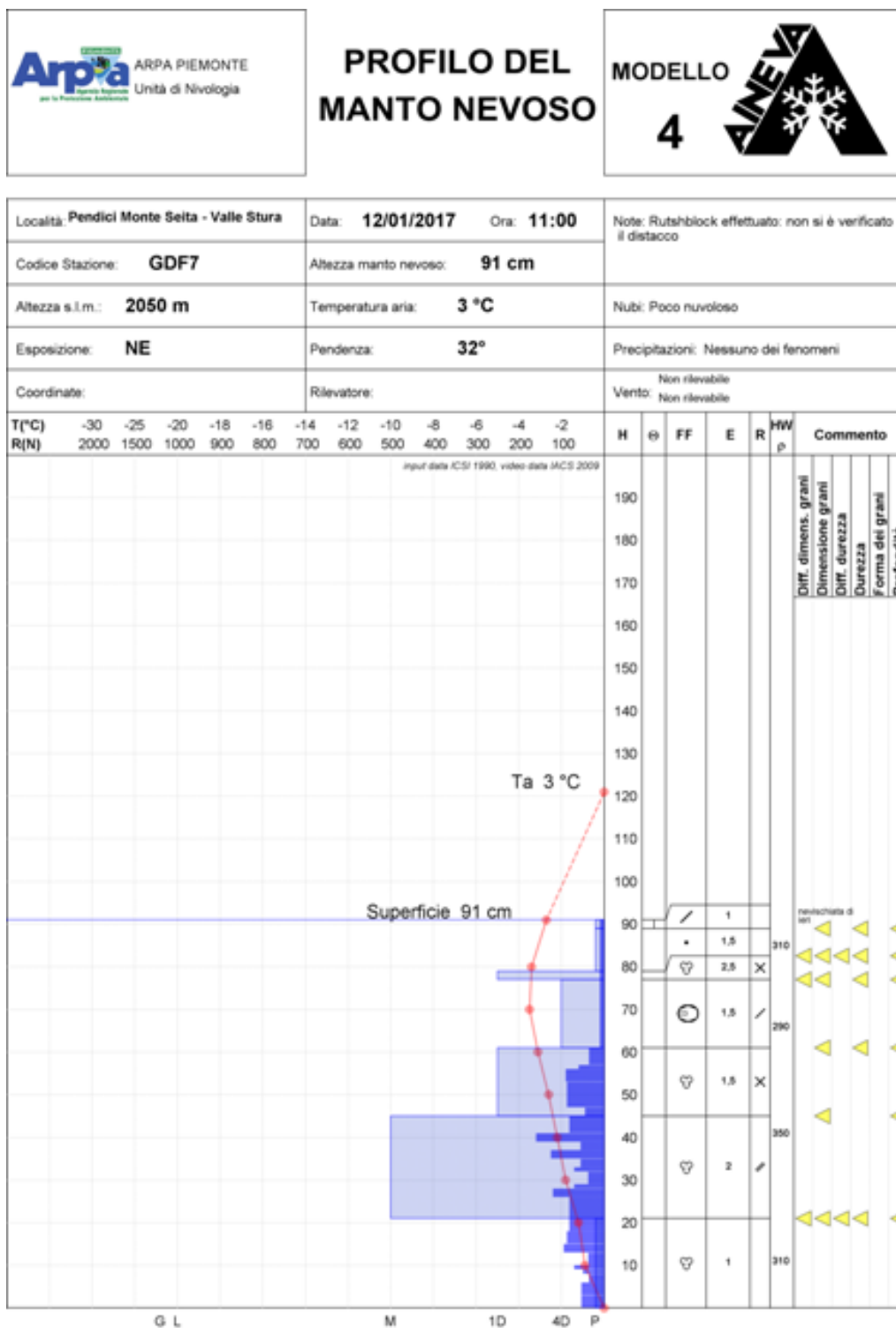
Figura 4.19: Profilo nivologico effettuato il giorno dopo l'incidente nei pressi della zona di distacco.
