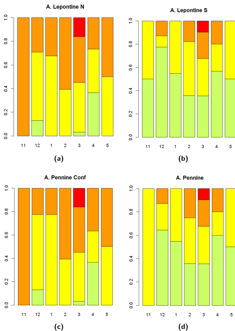
Figura 3.13: Distribuzione mensile dei gradi di pericolo valanghe emessi per i settori settentrionali 3.13b A.Leontine Sud, 3.13d A.Pennine, 3.13a A.Leontine Nord, 3.13c A. Pennine di Confine.
