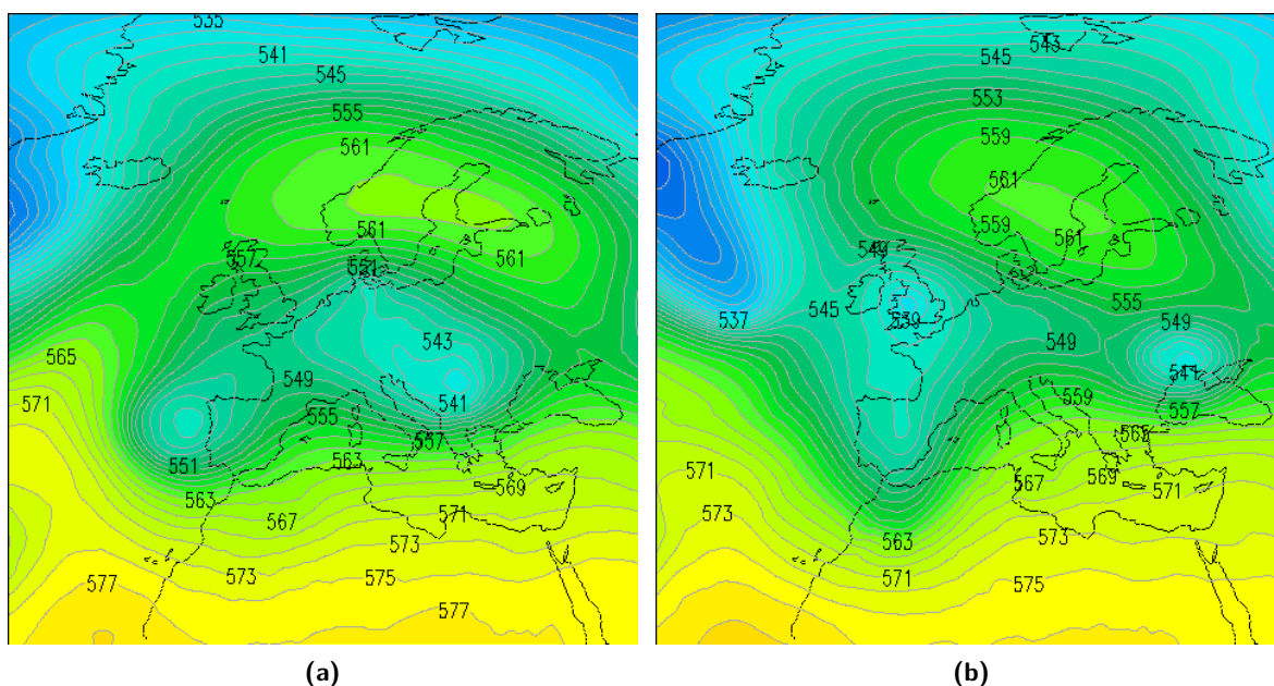
Figura 2.2: Analisi dell'altezza di geopotenziale a 500 hPa (dam) alle ore 12 UTC del 12 ottobre 2016 (2.2a) e del 13 ottobre 2016 (2.2b) che evidenziano la vasta circolazione depressionaria avente il minimo sull'Inghilterra ed estesa fino alla penisola iberica.
