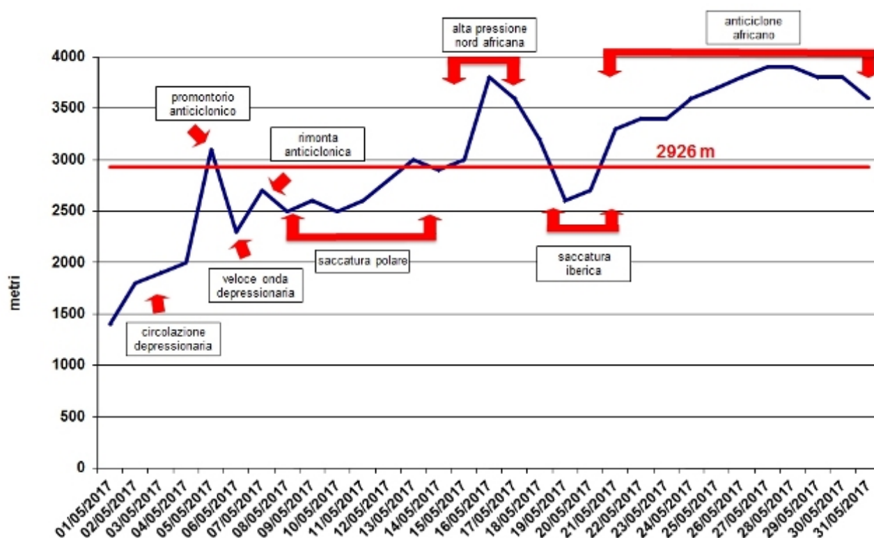
Figura 2.51: Andamento dello zero termico nel mese di maggio 2017 (in blu) e valore climatologico 1999-2015 (in rosso).
