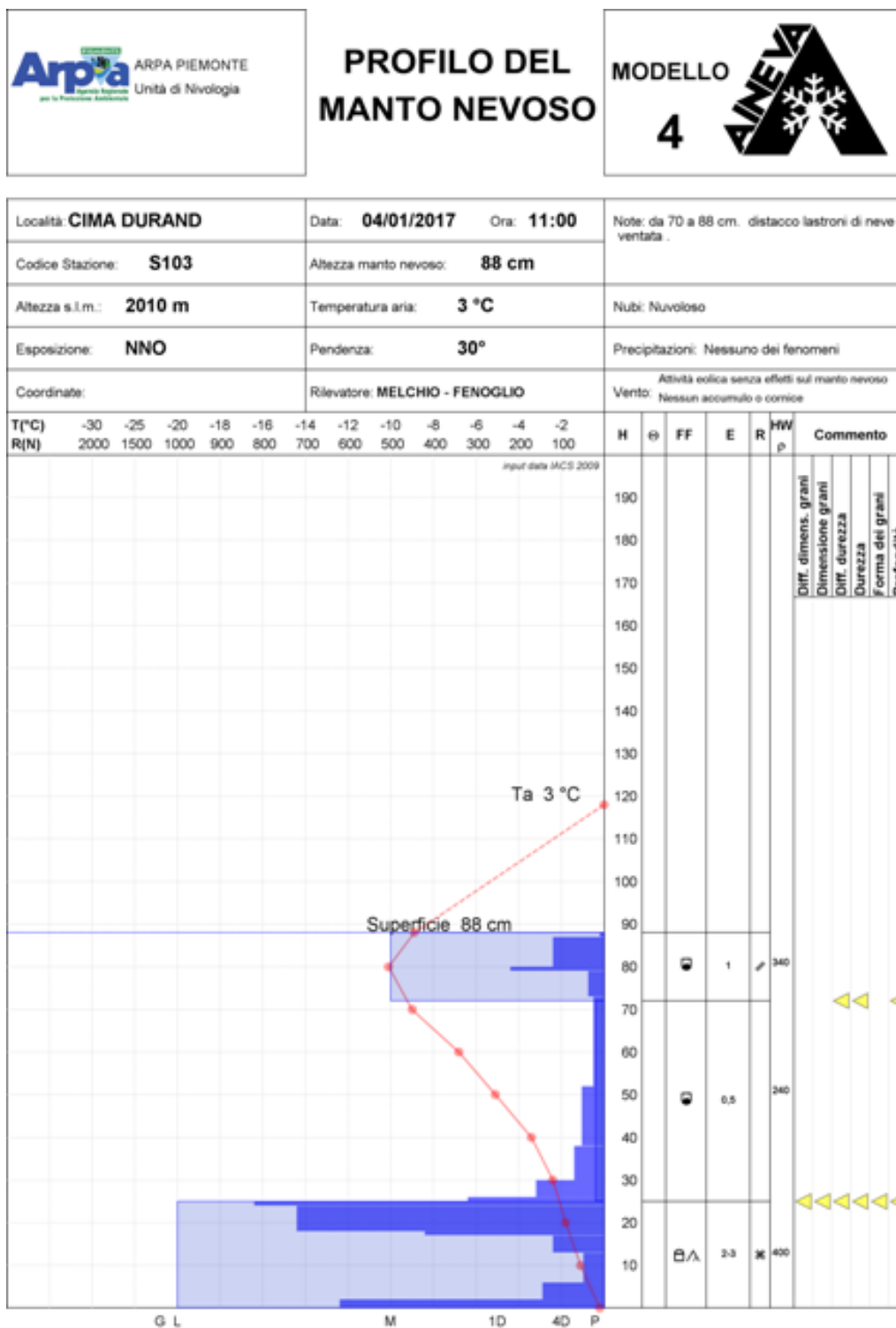
Figura 4.16: Profilo nivologico effettuato una settimana dopo l'incidente.
