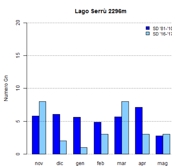
Giorni Nevosi mensili
