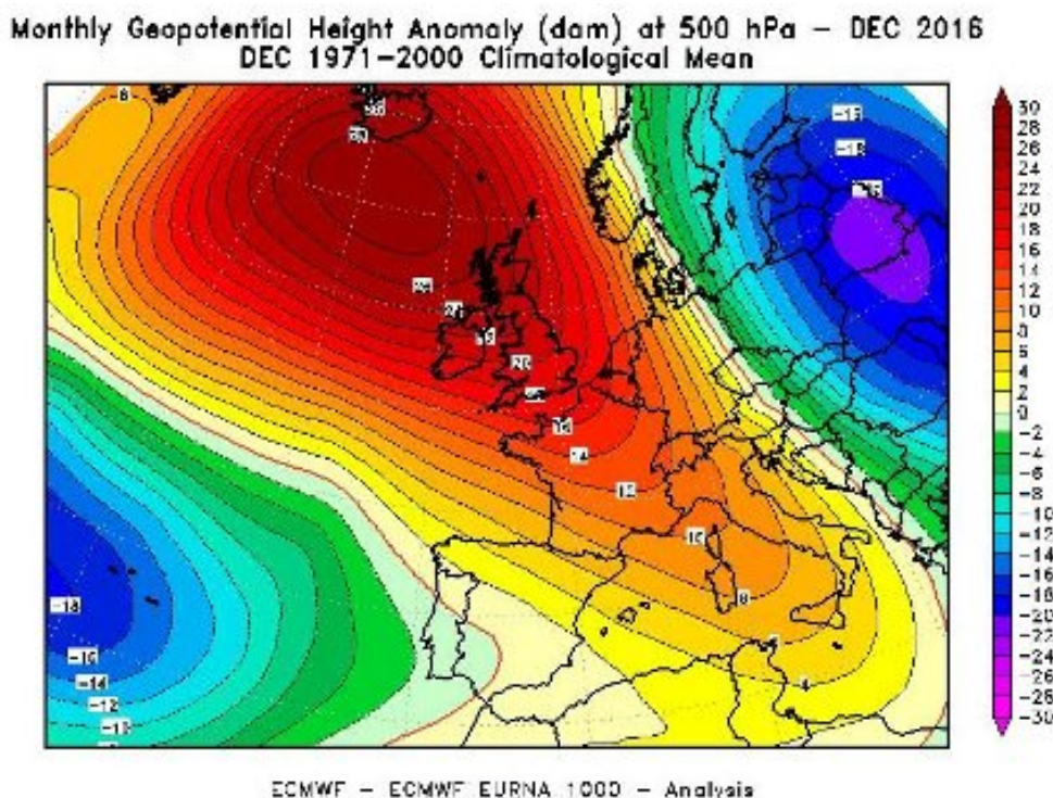
Figura 2.11: Anomalia dell'altezza di geopotenziale a 500 hPa del mese di dicembre 2016 rispetto alla climatologia del periodo 1971-2000. Elaborazione Arpa Piemonte su dati ECMWF.
