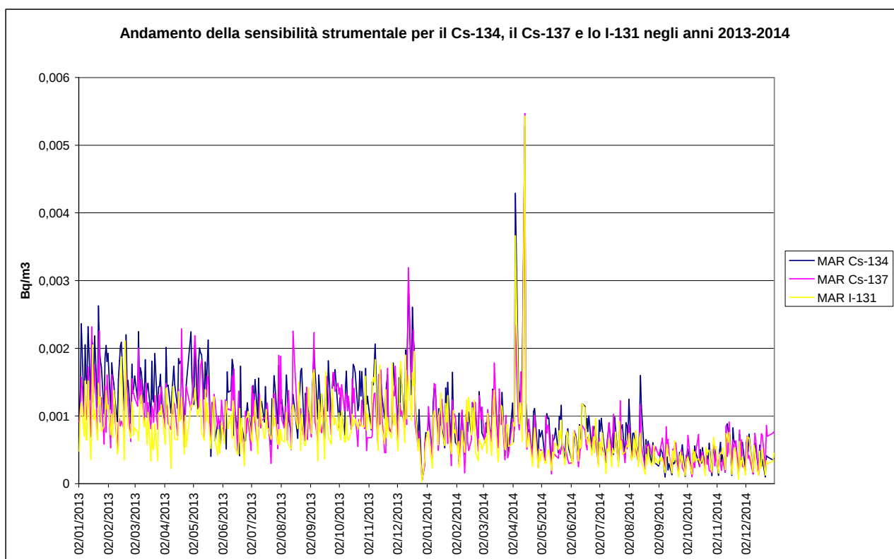
Figura 4: Andamento della sensibilità strumentale in spettrometria gamma per i filtri giornalieri del particolato atmosferico analizzati nel 2013 e 2014 per i radionuclidi artificiali di maggior interesse. Si nota come nei periodi in cui il volume di aria aspirato era inferiore la sensibilità peggiori, dando origine sul grafico a valori dell'ordine di 0,005 Bq/m 3 . Si tratta comunque, anche nel caso più sfavorevole, di sensibilità molto elevate: circa 1000 volte inferiori ai valori di radioattività che vennero misurati in aria in Italia durante l'incidente di Chernobyl.
