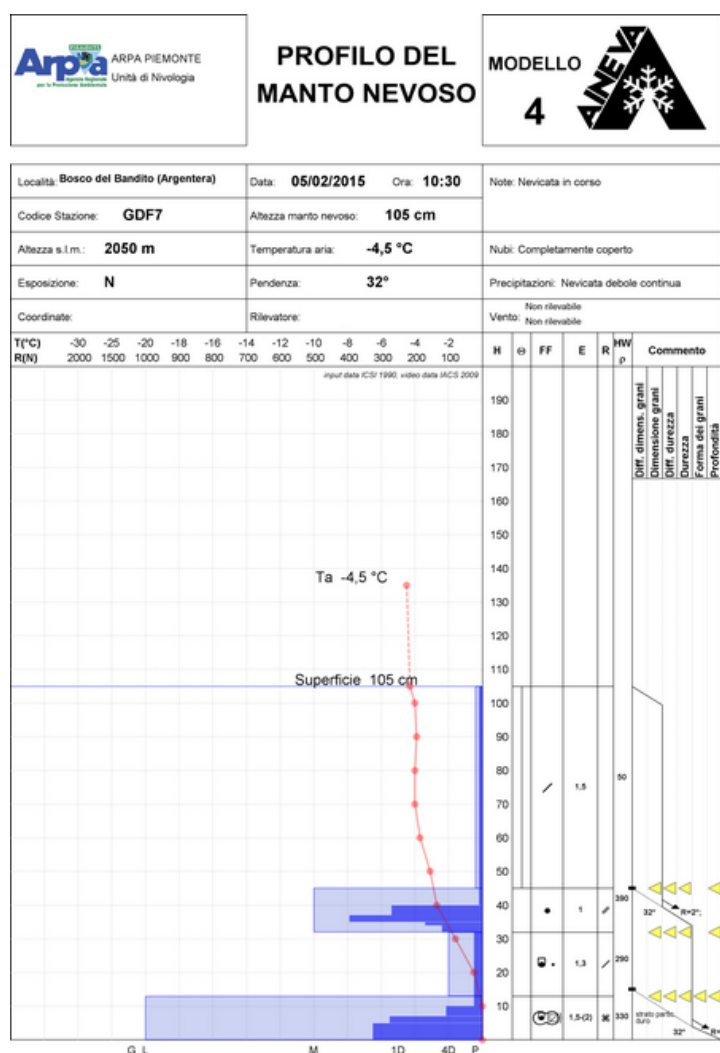
Figura 4.32: profilo del manto nevoso effettuato 2 giorni prima dell'incidente, non lontano dalla zona di distacco.
