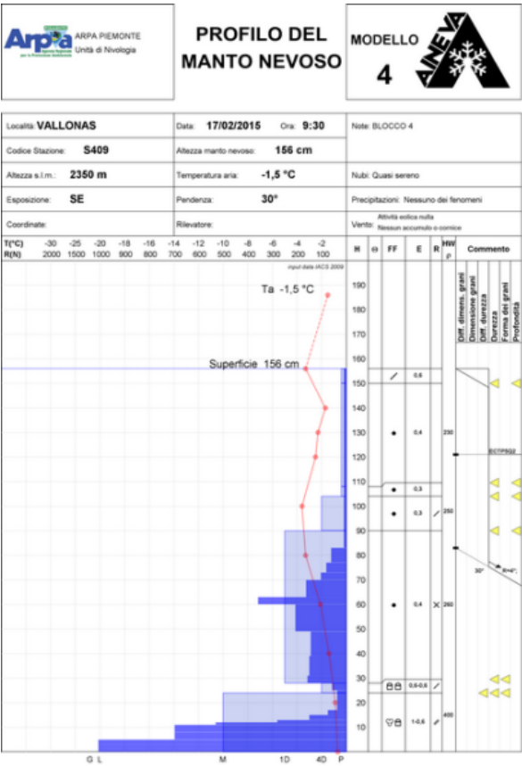
Figura 4.38: profilo del manto nevoso effettuato lo stesso giorno dell'incidente nel Comune di Sestriere.
