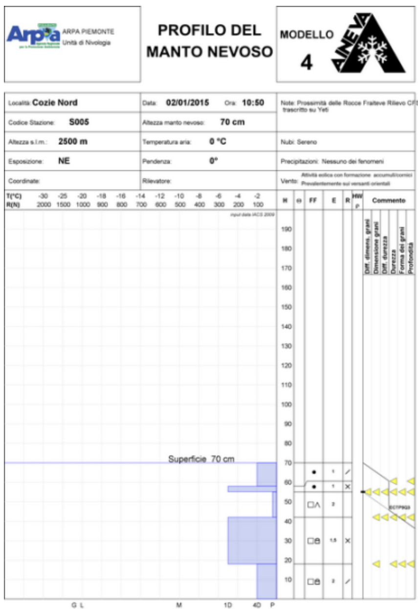
Figura 4.59: profilo nivologico speditivo realizzato il 02 gennaio.
