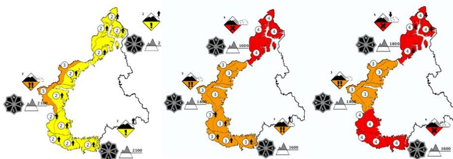
Figura 4.12: evoluzione del grado di pericolo: la prima mappa si riferisce alla tendenza espressa venerdì 13 per la domenica, mentre le altre due mappe si riferiscono al grado di pericolo espresso nel bollettino di lunedì 16 e martedì 17.
