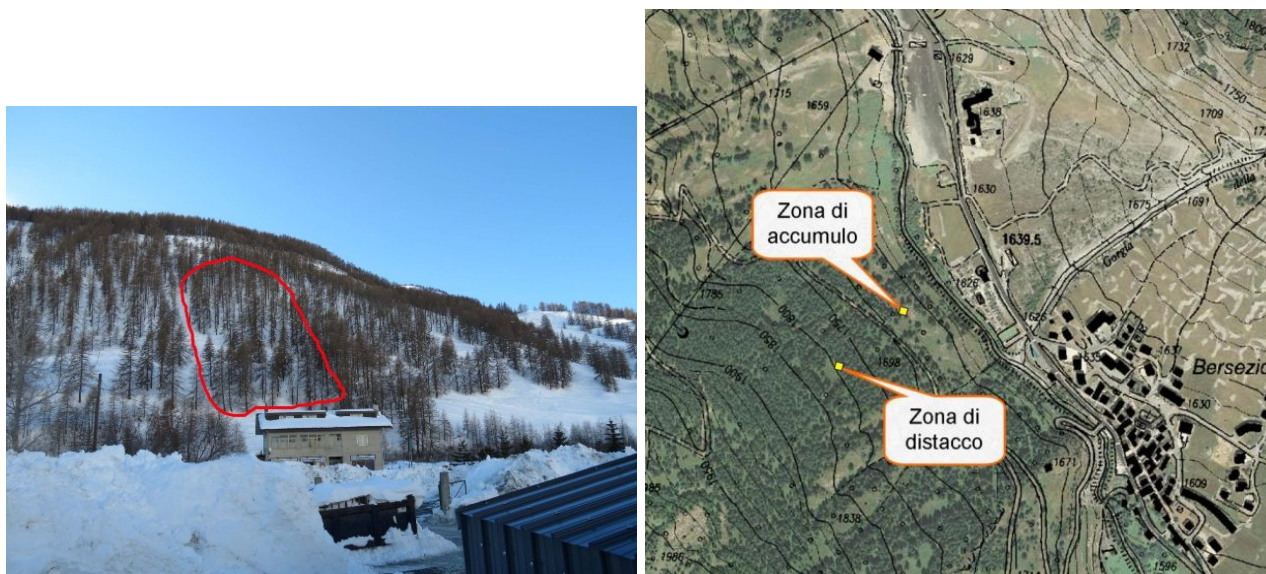
Figura 4.30: a sinistra la vista frontale della valanga; a destra l'estratto cartografico con evidenziate le zone di distacco e di accumulo.
