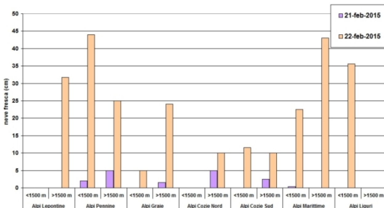
Figura 2.38: istogramma delle precipitazioni nevose per settore dalle stazioni di rilevamento manuale dal 21 al 22 febbraio 2015 . Le precipitazioni nevose sono misurate alle ore 8.00 locali e cumulate nelle 24 ore precedenti.
