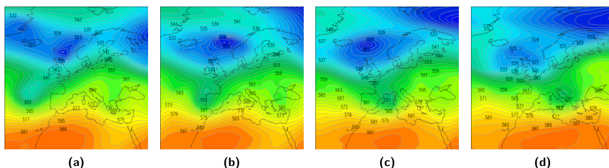
Figura 2.58: altezza di geopotenziale a 500 hPa alle ore 12 UTC del 25 (2.58a), 26 (2.58b), 27 (2.58c) e 28 (2.58d) aprile 2015.
