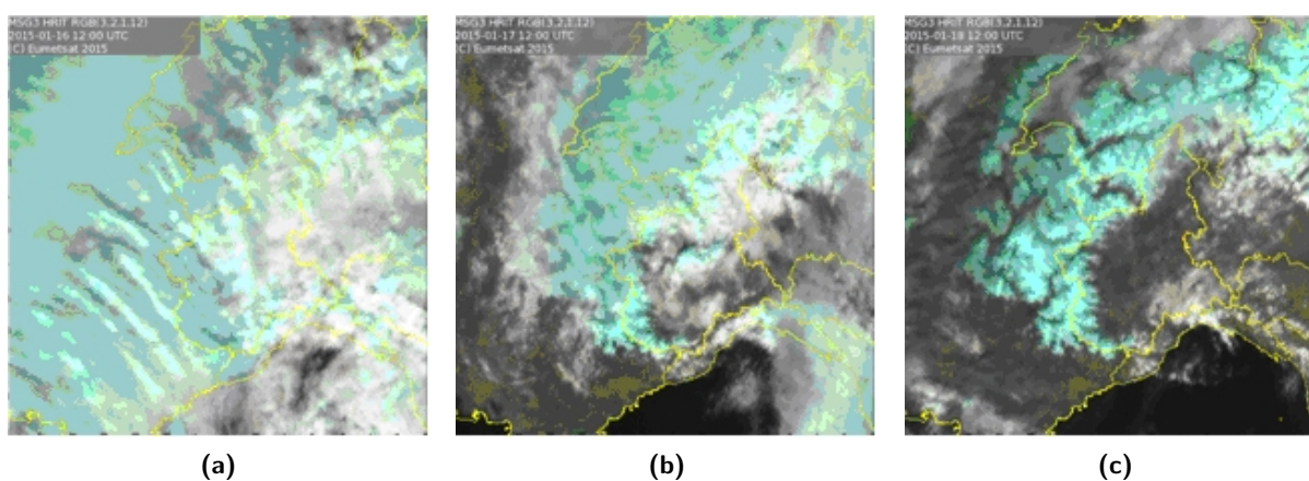
Figura 2.26: immagini da satellite dell'arco alpino occidentale dei giorni 16 (2.26a), 17 (2.26b) e 18 (2.26c) gennaio 2015 alle ore 12UTC.
