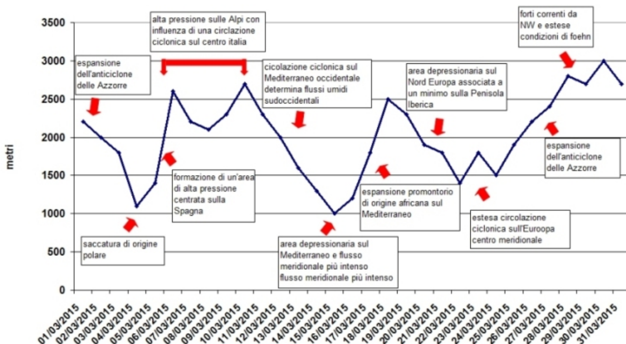
Figura 2.40: andamento dello zero termico nel mese di marzo 2015 (in blu).
