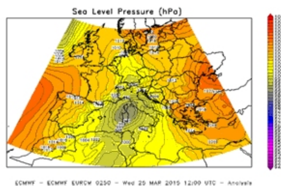
Figura 2.50: Analisi della pressione al livello del mare alle ore 12 UTC di mercoledì 25 marzo .
