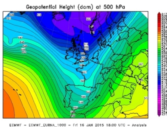
Figura 2.23: altezza di geopotenziale a 500 hPa alle ore 18 UTC del 16 gennaio 2015 . Elaborazione Arpa Piemonte su dati ECMWF.
