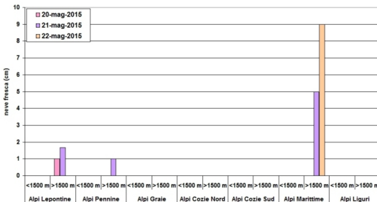
Figura 2.65: istogramma delle precipitazioni nevose per settore dalle stazioni di rilevamento manuale dal 20 al 22 maggio 2015 . Le precipitazioni nevose sono misurate alle ore 8.00 locali e cumulate nelle 24 ore precedenti.
