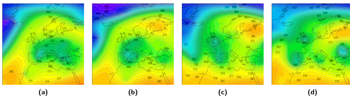
Figura 2.41: altezza di geopotenziale a 500hPa alle ore 12UTC del 14 (2.41a), 15 (2.41b), 16 (2.41c) e 17 (2.41d) marzo 2015 .
