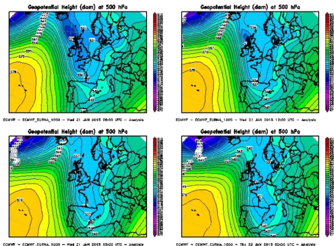
Figura 2.27: evoluzione dell'altezza di geopotenziale a 500 hPa tra le 06 UTC del 21 gennaio (in alto a sinistra) e le ore 00 UTC del 22 gennaio 2015 (in basso a destra), intervallata ogni 6 ore.
