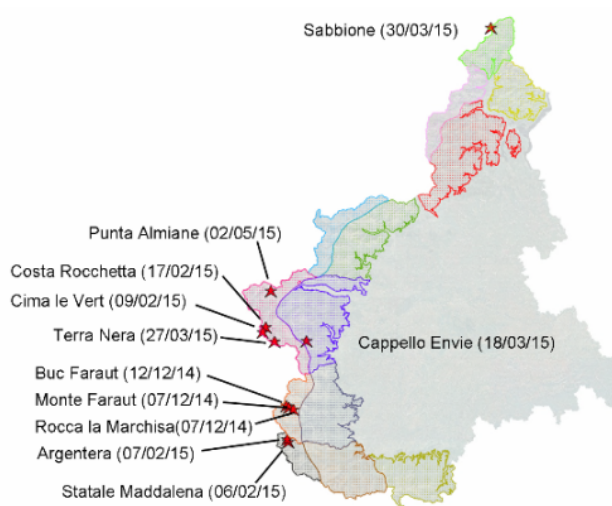
Figura 4.25: distribuzione degli incidenti da valanga sull'arco alpino piemontese nella stagione invernale 2014-15.
