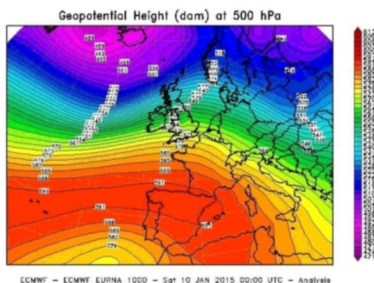
Figura 2.20: altezza di geopotenziale a 500 hPa alle ore 00 UTC del 10 gennaio 2015 . Elaborazione Arpa Piemonte su dati ECMWF.
