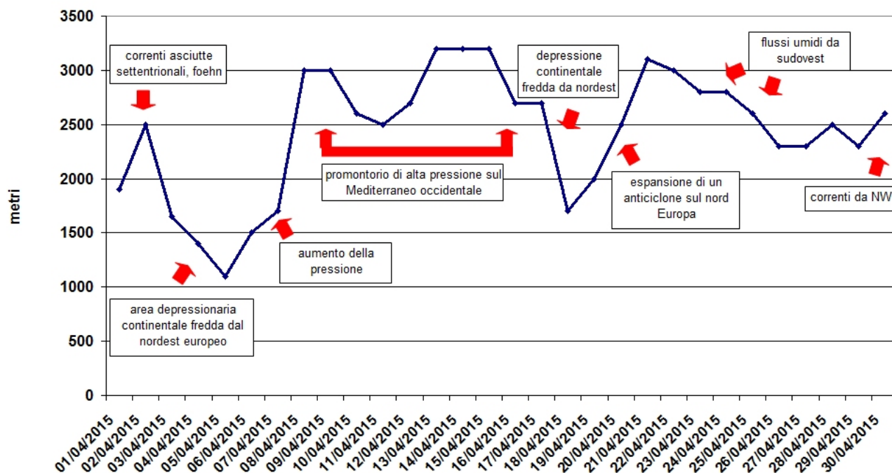
Figura 2.56: andamento dello zero termico nel mese di aprile 2015 (in blu).
