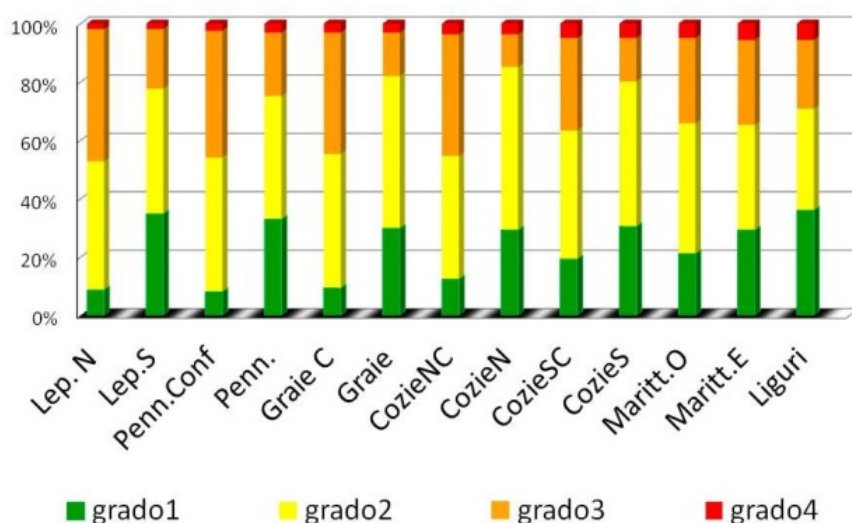
Figura 3.10: distribuzione percentuale dei gradi di pericolo suddivisa per settore nella stagione 2014-15.
