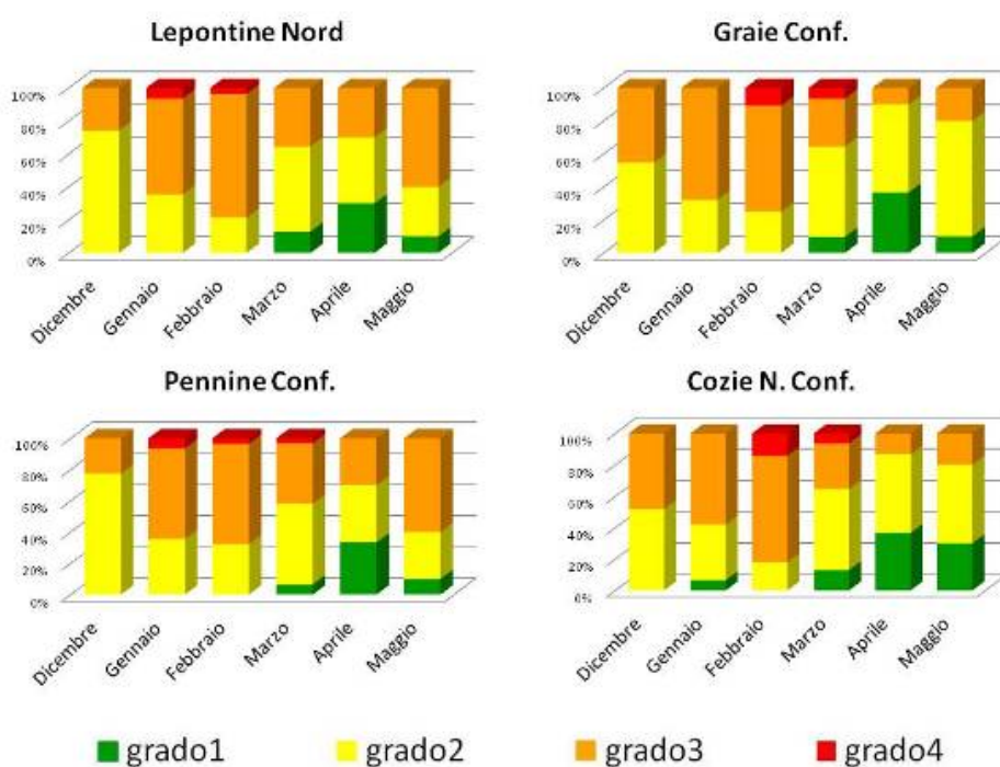
Figura 3.11: andamento dei gradi di pericolo nella fascia di confine dei settori settentrionali ed occidentali da dicembre 2014 a maggio 2015.
