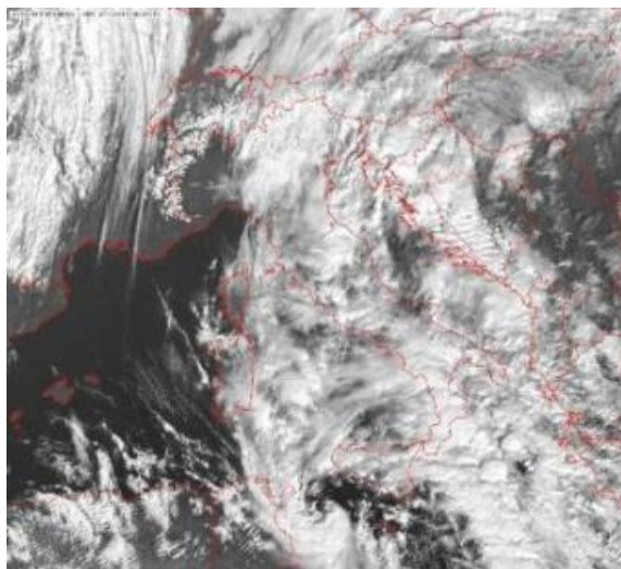
Figura 2.3: immagine satellitare nel canale del visibile del giorno 7 novembre 2014 alle ore 9 UTC.
