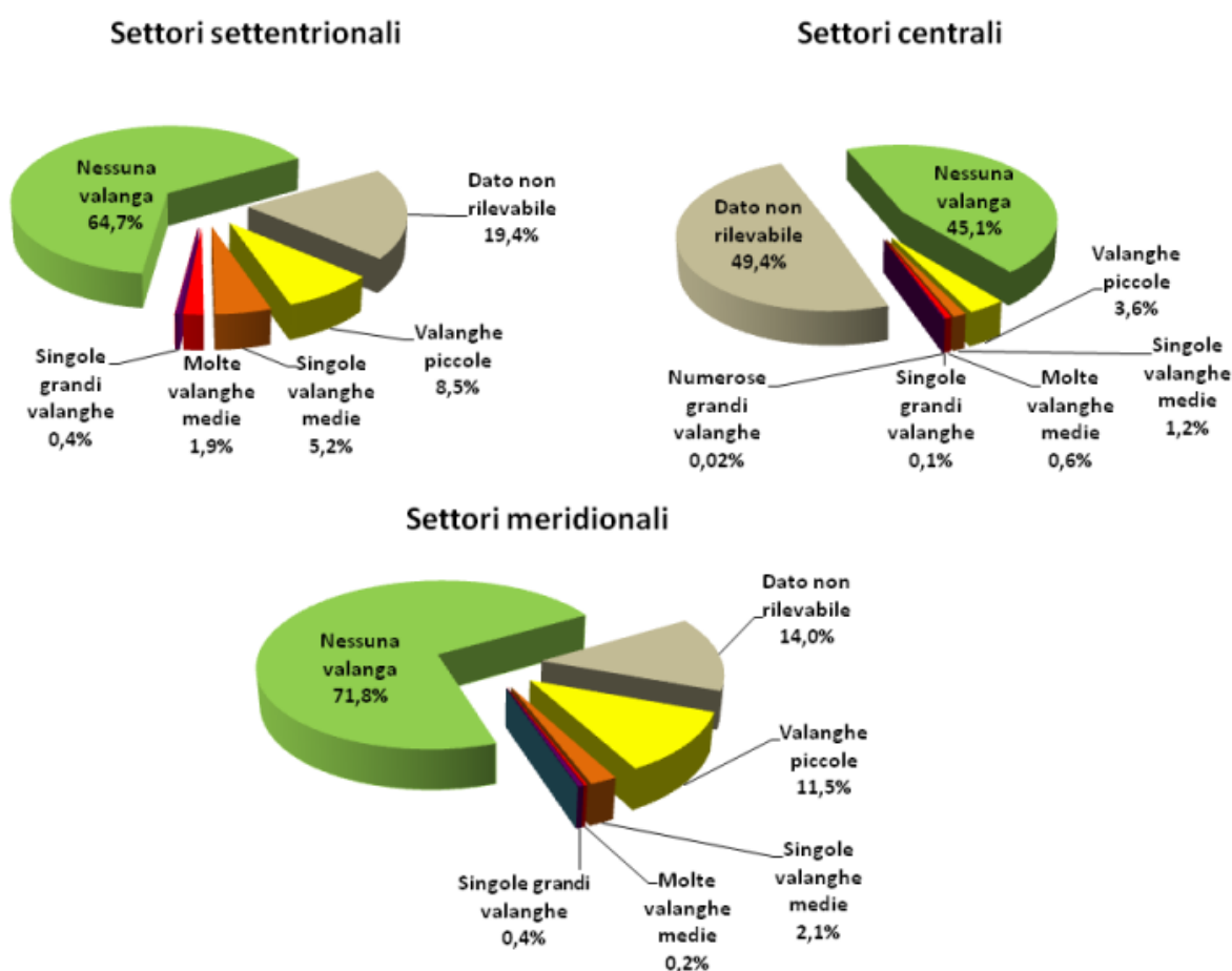
Figura 4.4: attività valanghiva spontanea segnalata nella stagione 2014-15 suddivisa per settori.
