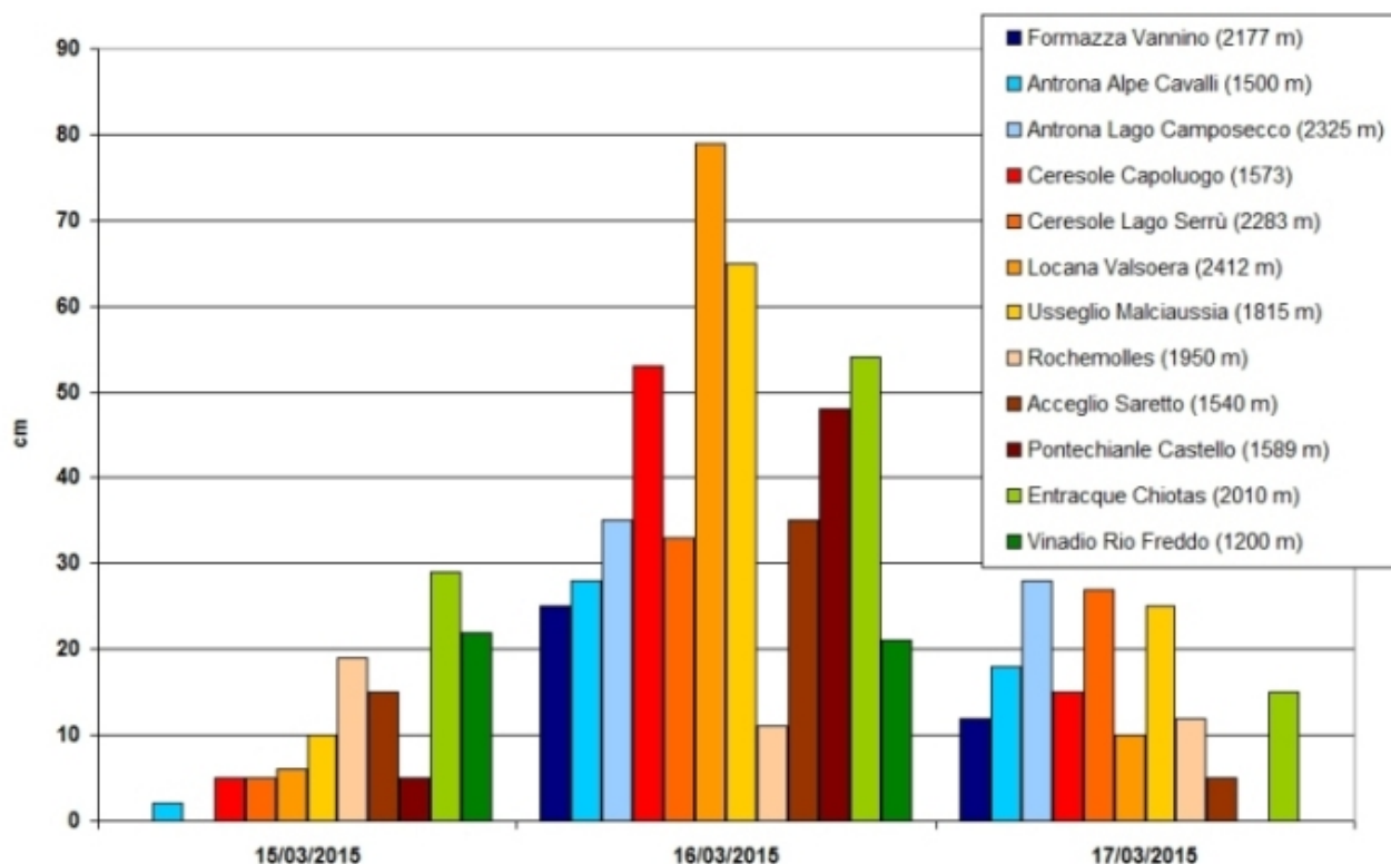
Figura 2.45: altezza della neve fresca giornaliera in alcune stazioni di rilevamento manuale dal 15 al 17 marzo 2015 . Con le gradazioni di blu sono indicate le località dei settori nord, con quelle di rosso/arancione/marrone quelle dei settori ovest, mentre con le gradazioni di verde quelle dei settori sud. Le precipitazioni nevose sono misurate alle ore 8.00 locali e cumulate nelle 24 ore precedenti.
