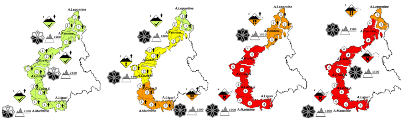
Figura 4.15: rapida evoluzione del grado di pericolo da sabato 14 a martedì 17 marzo.
