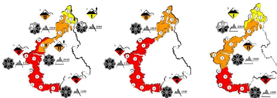
Figura 4.6: evoluzione del grado di pericolo riportato nel bollettino valanghe di venerdì 6 Febbraio .
