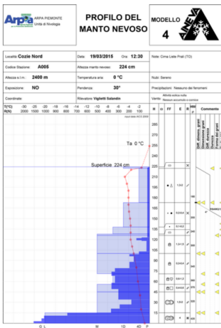
Figura 4.42: profilo nivologico effettuato il giorno dopo l'incidente alla stessa quota della zona di distacco.
