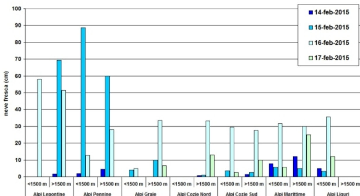
Figura 2.35: istogramma delle precipitazioni nevose per settore dalle stazioni di rilevamento manuale dal 14 al 17 febbraio 2015. Le precipitazioni nevose sono misurate alle ore 8.00 locali e cumulate nelle 24 ore precedenti.
