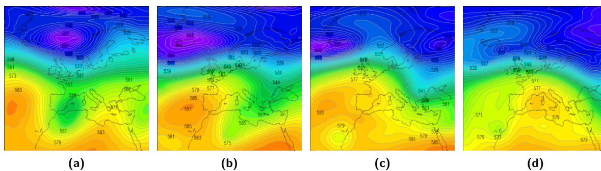
Figura 2.13: altezza di geopotenziale a 500hPa del 15(2.13a), 18 (2.13b), 21 (2.13c) e 23 (2.13d) dicembre 2014.
