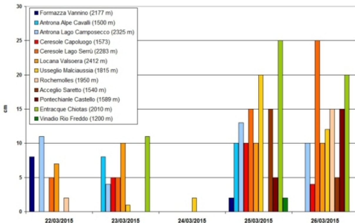
Figura 2.48: altezza della neve fresca giornaliera in alcune stazioni di rilevamento manuale dal 22 al 26 marzo 2015 . Con le gradazioni di blu sono indicate le località dei settori nord, con quelle di rosso/arancione/marrone quelle dei settori ovest, mentre con le gradazioni di verde quelle dei settori sud. Le precipitazioni nevose sono misurate alle ore 8.00 locali e cumulate nelle 24 ore precedenti.
