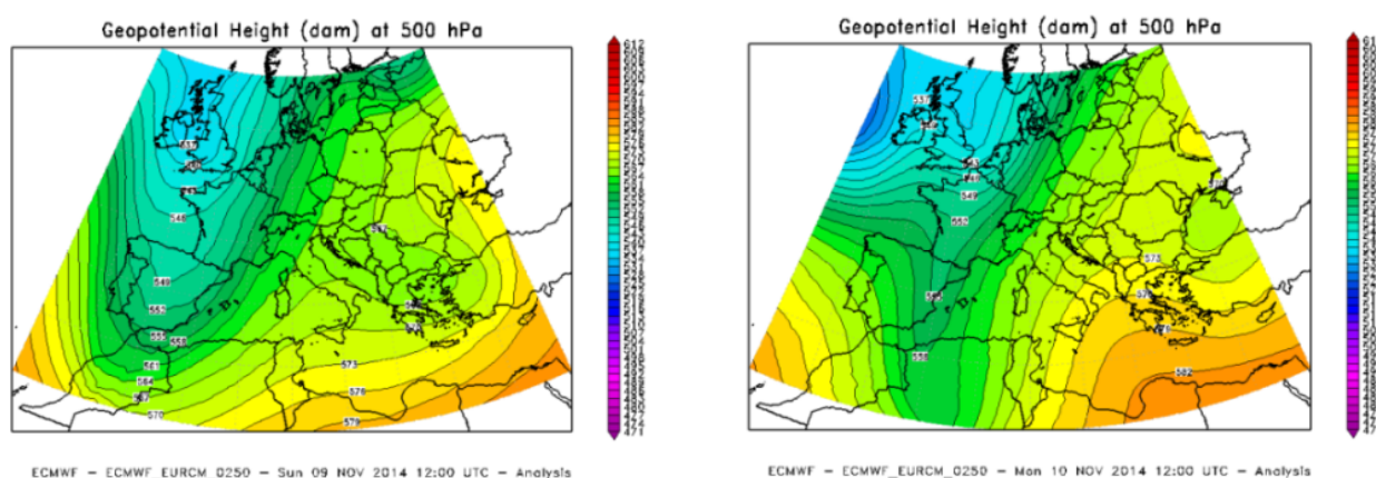
Figura 2.4: analisi dell'altezza di geopotenziale a 500 hPa alle ore 12 UTC del 9 novembre 2014 (a sinistra) e del 10 novembre 2014 (a destra) che evidenziano le configurazioni che hanno determinato maltempo sul Piemonte.
