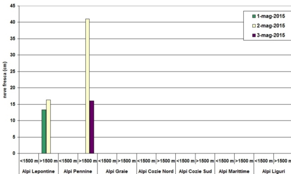
Figura 2.62: istogramma delle precipitazioni nevose per settore dalle stazioni di rilevamento manuale dall'1 al 3 maggio 2015. Le precipitazioni nevose sono misurate alle ore 8.00 locali e cumulate nelle 24 ore precedenti.
