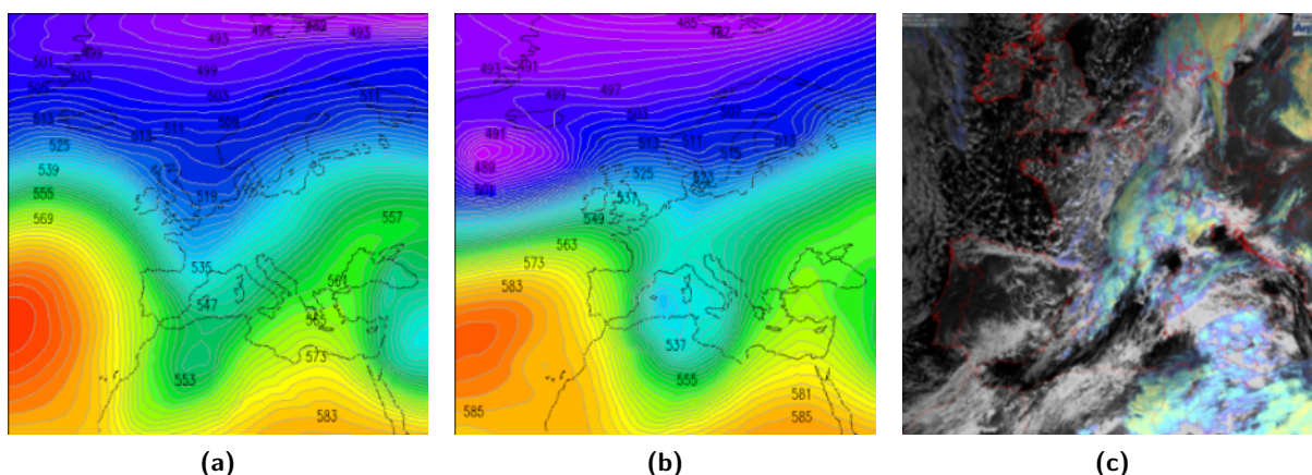
Figura 2.37: altezza di geopotenziale a 500hPa alle ore 12UTC del 21 (2.37a) e 22 (2.37b) febbraio 2015 , immagine da satellite Meteosat bi-spettrale del 21 febbraio alle ore 12 UTC (2.37c).
