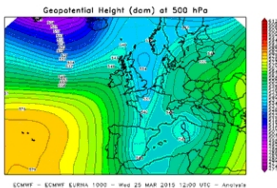
Figura 2.49: Analisi dell'altezza di geopotenziale a 500 hPa alle ore 12 UTC di mercoledì 25 marzo .
