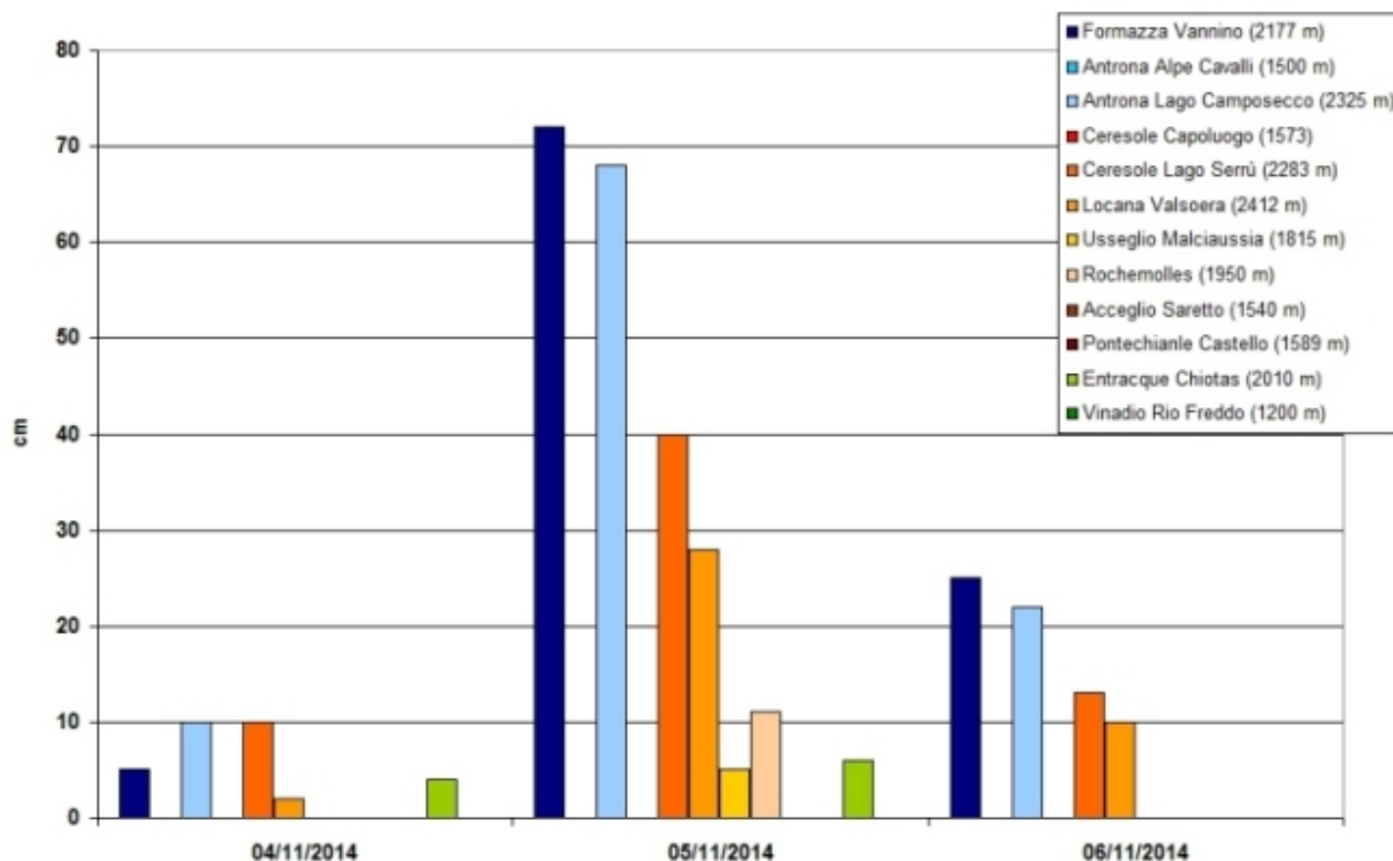
Figura 2.1: altezza della neve fresca giornaliera in alcune stazioni di rilevamento manuale durante l'evento del 4-6 novembre 2014 . Con le gradazioni di blu sono indicate le località dei settori nord, con quelle di rosso/arancione/marrone quelle dei settori ovest, mentre con le gradazioni di verde quelle dei settori sud. Le precipitazioni nevose sono misurate alle ore 8.00 locali e cumulate nelle 24 ore precedenti.
