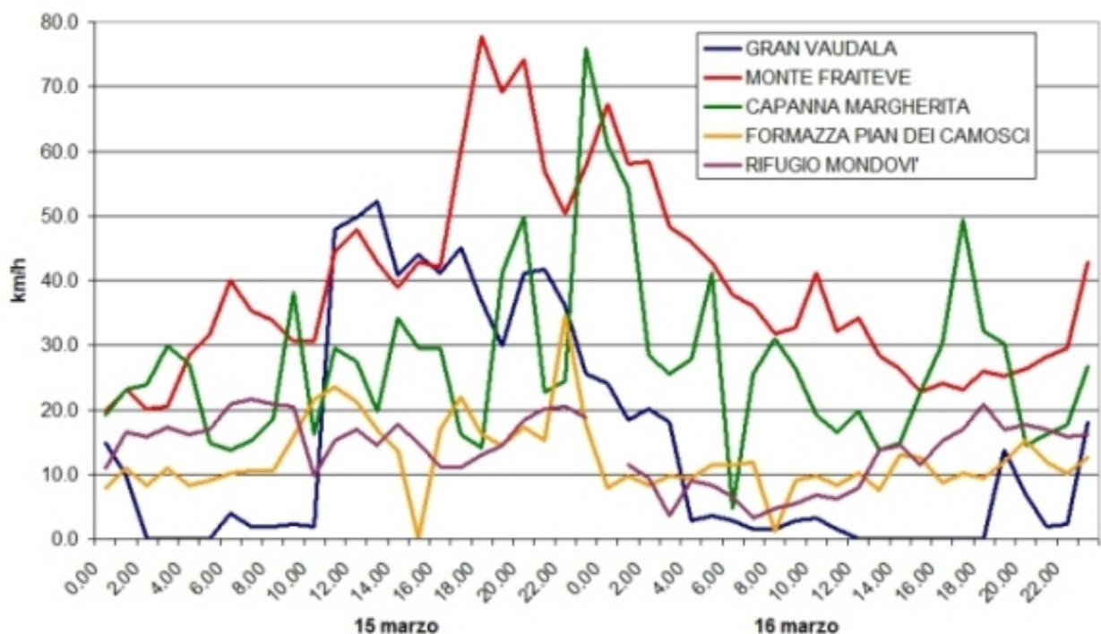
Figura 2.46: Andamento della massima raffica oraria dei giorni 15 e 16 marzo per alcune stazioni di montagna della rete di Arpa Piemonte.
