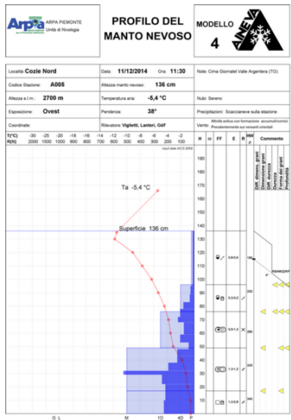
Figura 4.55: profilo del manto nevoso effettuato 3 giorni dopo il distacco della valanga.
