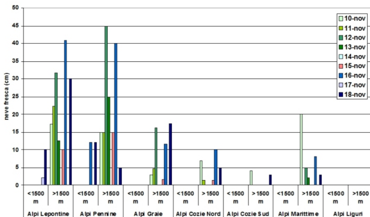
Figura 2.6: istogramma delle precipitazioni nevose per settore nei giorni dal 10 al 18 novembre 2014 delle stazioni manuali, si osservi come le precipitazioni nevose abbiano interessato soprattutto il settore nord-occidentale del Piemonte. Le precipitazioni nevose sono misurate alle ore 8.00 locali e cumulate nelle 24 ore precedenti.
