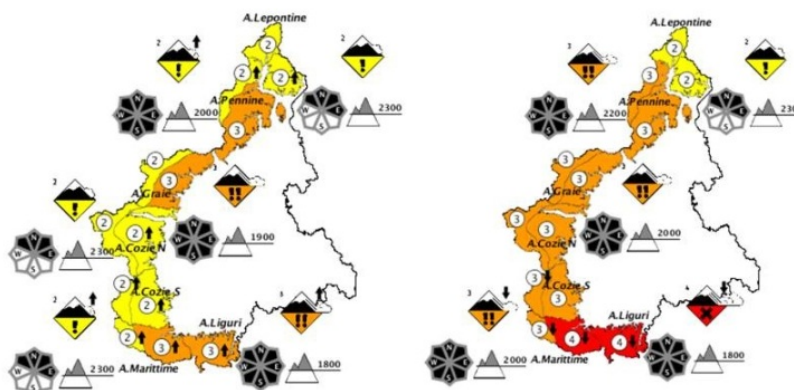
Figura 4.16: grado di pericolo emesso per le giornate del 25 e 26 marzo.
