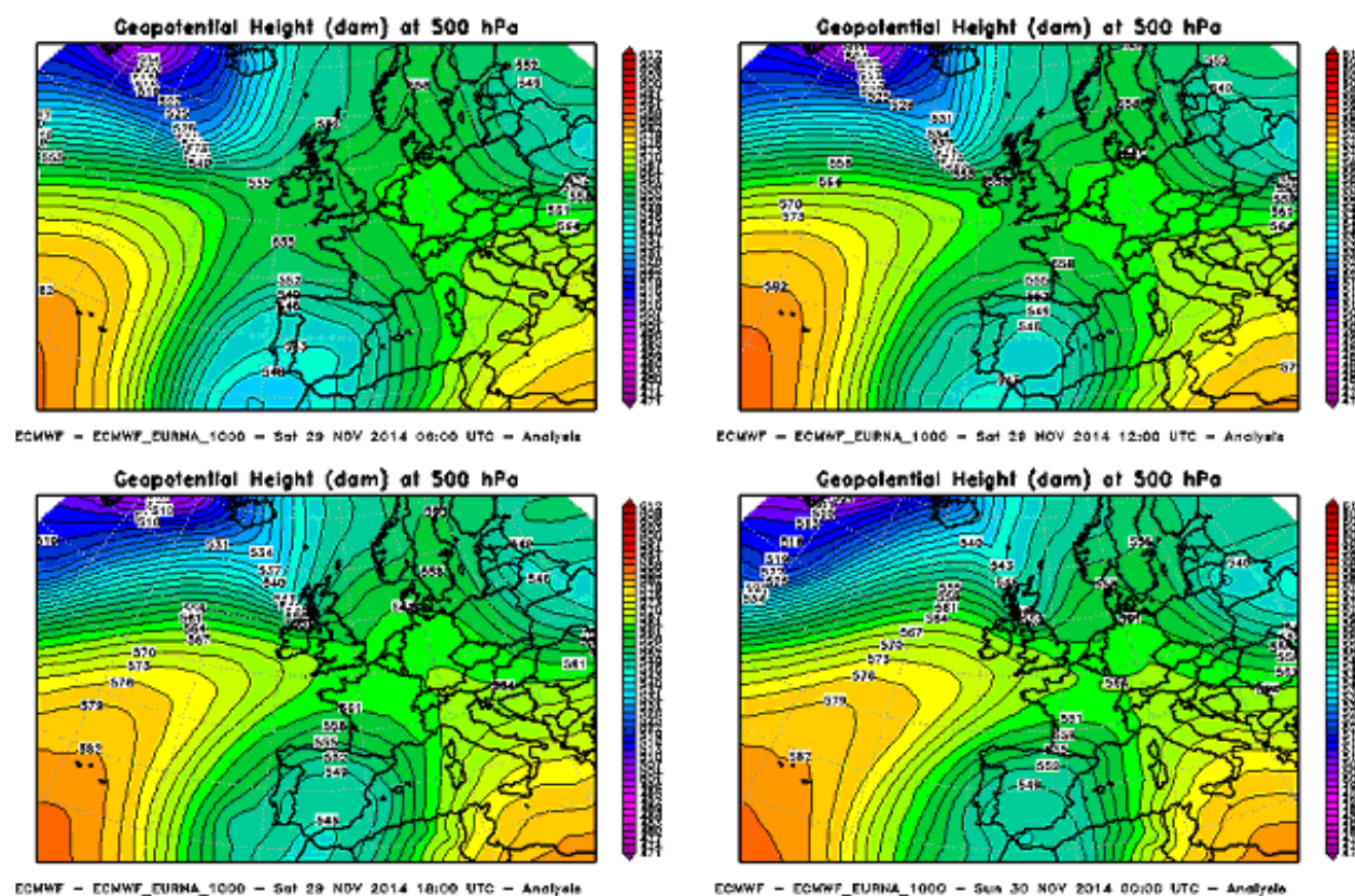
Figura 2.7: analisi dell'altezza di geopotenziale a 500 hPa alle ore 00 UTC del 29 novembre 2014 (in alto a sinistra), alle 12 UTC del 29 novembre 2014 (in alto a destra), alle ore 18 UTC del 29 novembre 2014 (in basso a sinistra) e alle 00 UTC del 30 novembre 2014 (in basso a destra).
