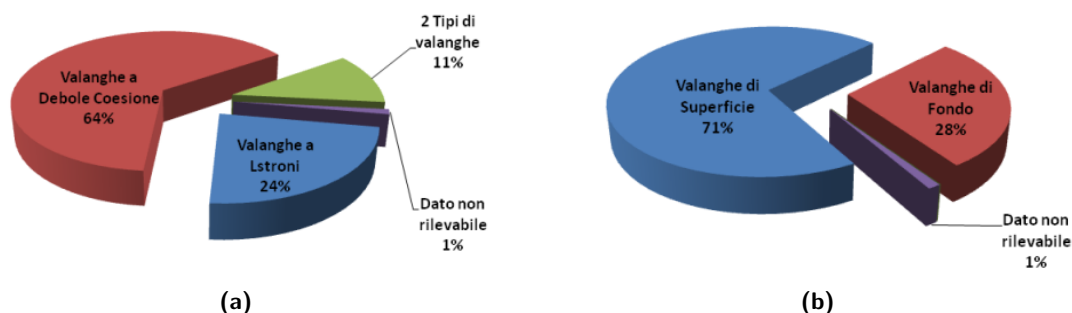
Figura 4.2: 4.2a, 4.2b tipologie di valanghe osservate nella stagione 2014-15.
