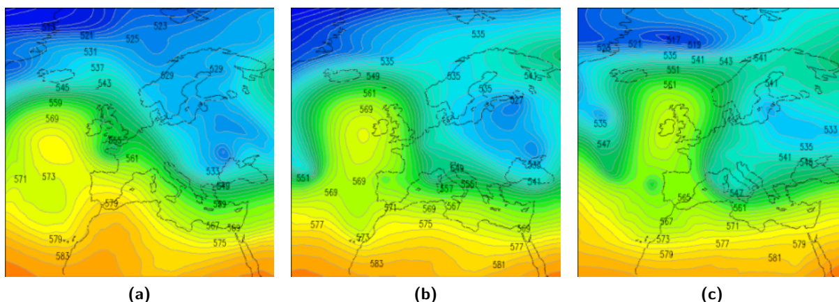
Figura 2.54: altezza di geopotenziale a 500hPa alle ore 12UTC del 3 (2.54a) , 4 (2.54b) e 5 (2.54c) aprile 2015 .
