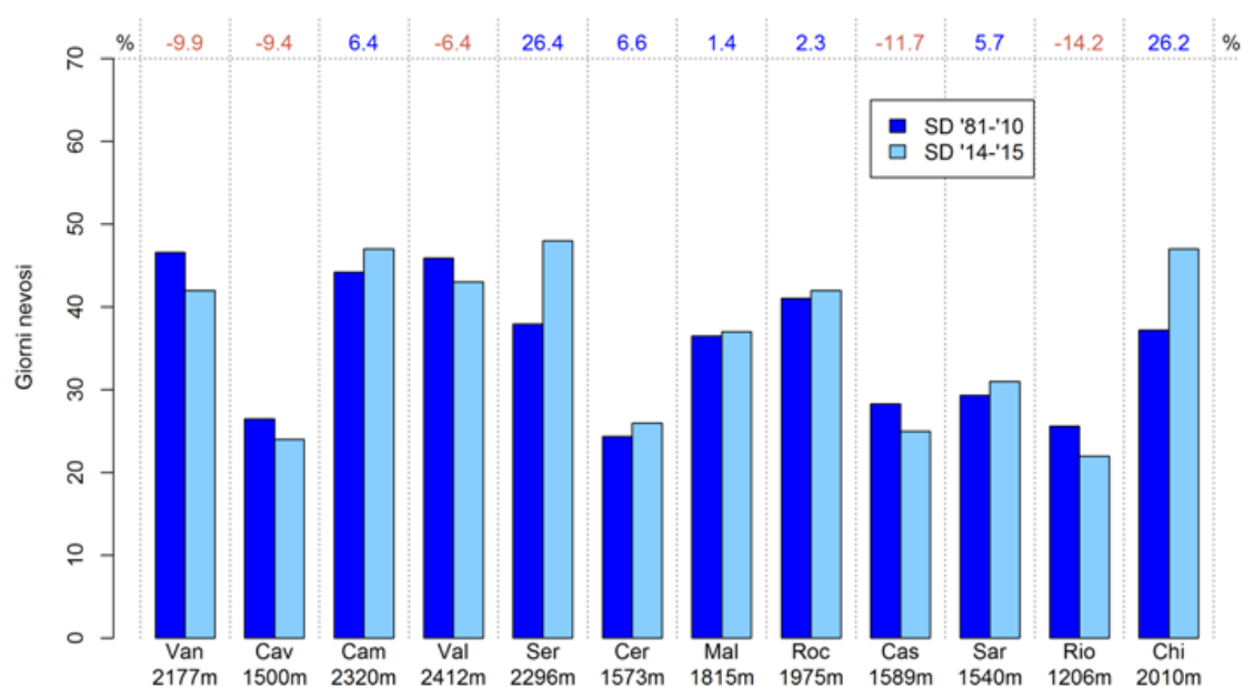
Figura 1.3: giorni Nevosi (SD) da novembre a maggio stagione 2014-2015 (in azzurro) a confronto con la media trentennale '81-'10 (in blu).
