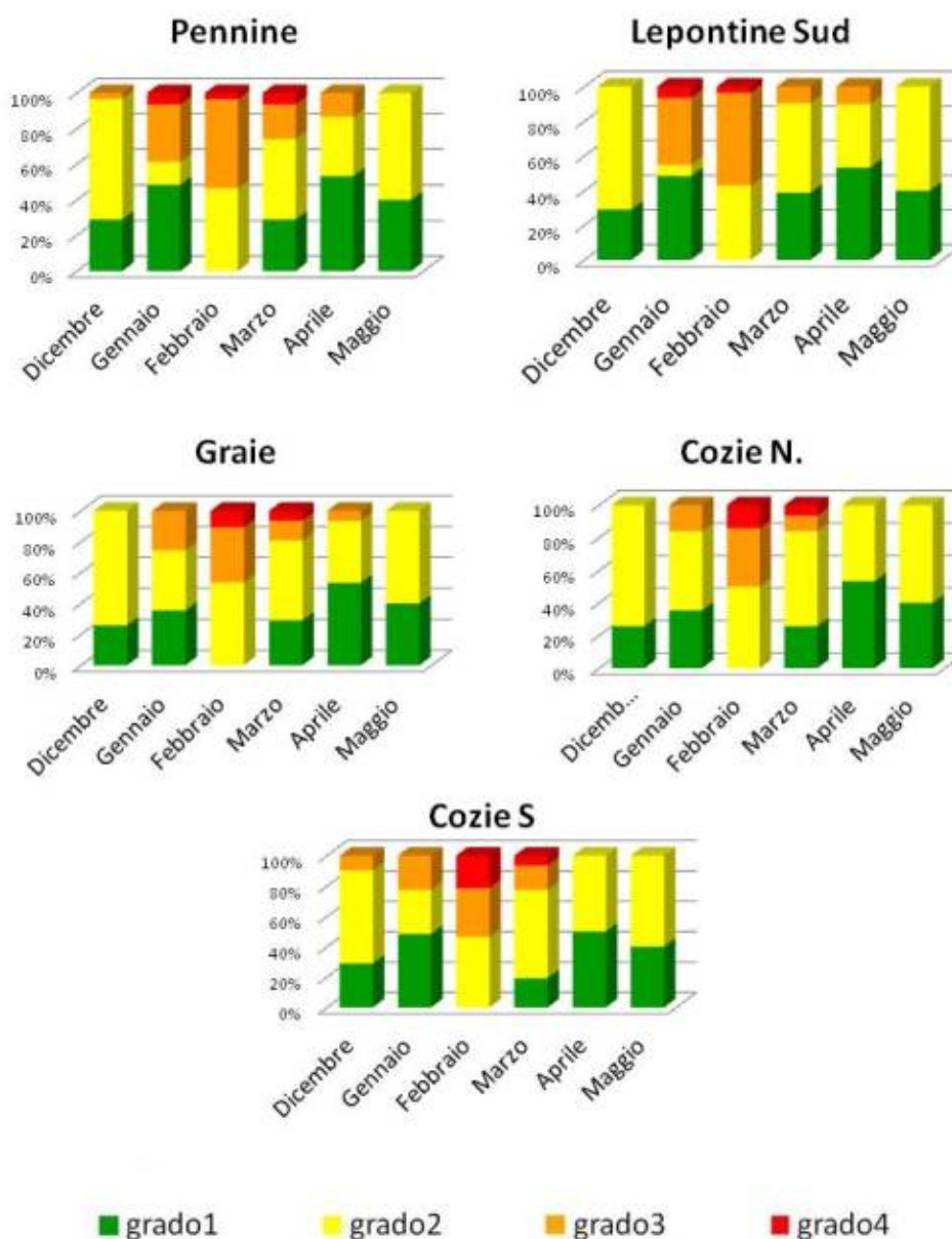
Figura 3.12: andamento dei gradi di pericolo nella fascia pedemontana dei settori settentrionali ed occidentali da dicembre 2014 a maggio 2015.
