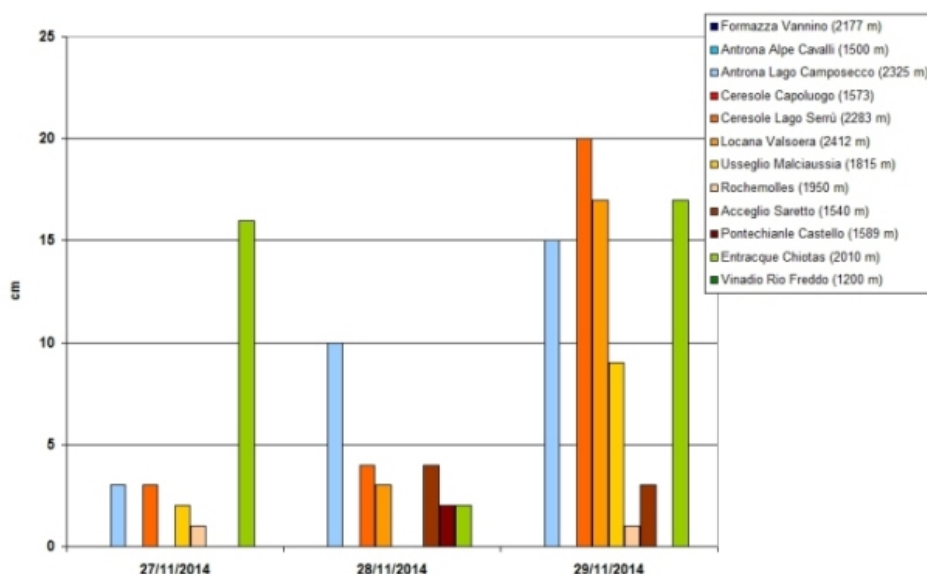
Figura 2.8: altezza della neve fresca giornaliera in alcune stazioni di rilevamento manuale durante l'evento del 27-29 novembre 2014 . Con le gradazioni di blu sono indicate le località dei settori nord, con quelle di rosso/arancione/marrone quelle dei settori ovest, mentre con le gradazioni di verde quelle dei settori sud. Le precipitazioni nevose sono misurate alle ore 8.00 locali e cumulate nelle 24 ore precedenti.
