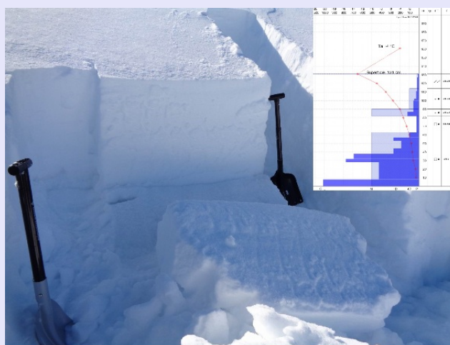
Figura 2.39: Il test di stabilità della colonna estesa - ECT effettuato lo stesso giorno in val Soana ha evidenziato la debolezza all'interfaccia con lo strato di cristalli sfaccettati. La struttura del manto risultava molto simile a quella del profilo sopra descritto.
