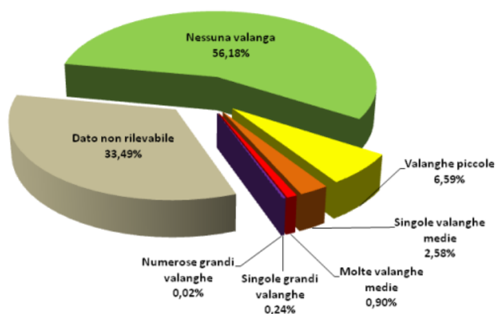
Figura 4.1: attività valanghiva spontanea segnalata nella stagione 2014-15.
