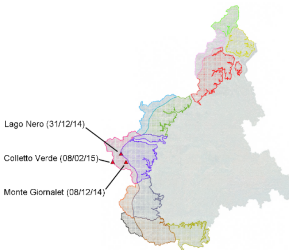
Figura 4.52: localizzazione delle valanghe provocate, i contorni colorati rappresentano i confini dei settori alpini piemontesi riportati nei Bollettini Valanghe.
