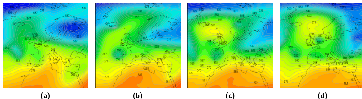
Figura 2.57: altezza di geopotenziale a 500hPa alle ore 12UTC del 16 (2.57a), 17 (2.57b), 18 (2.57c) e 19 (2.57d) aprile 2015.
