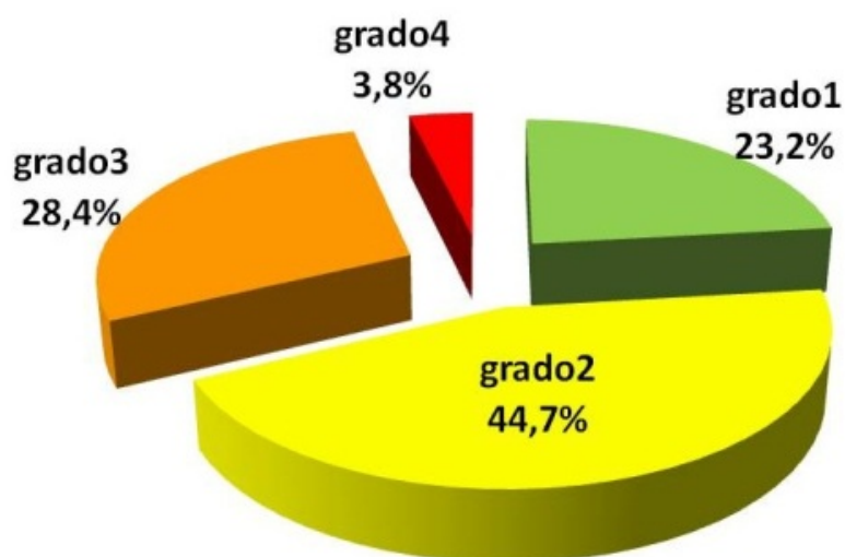
Figura 3.9: frequenza di utilizzo dei gradi di pericolo sull'arco alpino piemontese nella stagione 2014-15.
