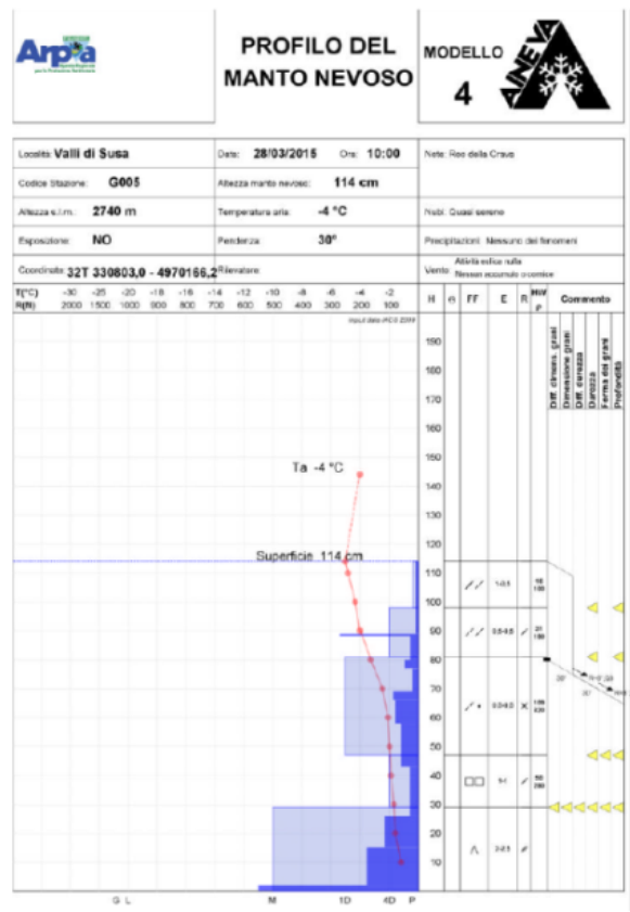
Figura 4.46: profilo nivologico effettuato il giorno dopo l'incidente nella zona di distacco della seconda valanga.
