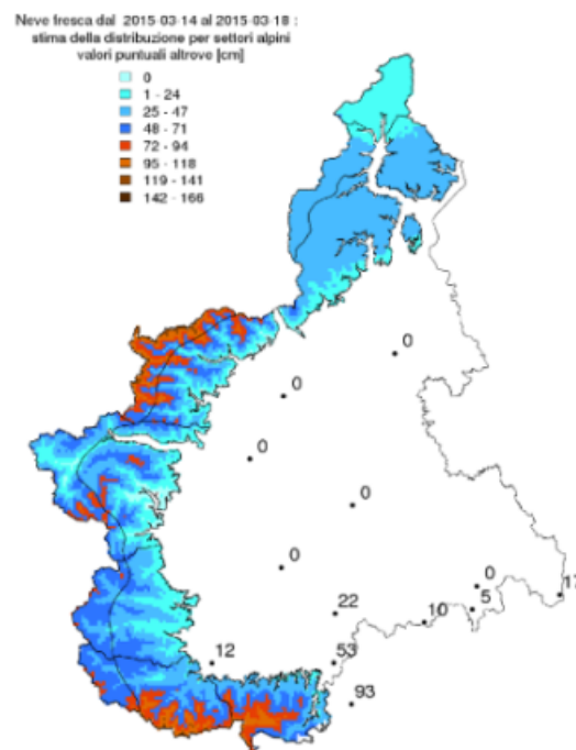
Figura 2.43: mappa della stima della distribuzione della neve fresca cumulata dal 14 al 18 marzo 2015 sui settori alpini piemontesi del Bollettino Valanghe.
