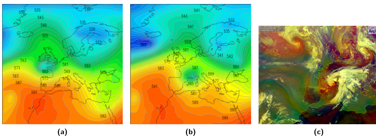
Figura 2.63: altezza di geopotenziale a 500hPa alle ore 12UTC del 14 (2.63a) e 15 maggio (2.63b) e immagine da satellite bi spettrale del 15 maggio alle ore 12 UTC (2.63c).
