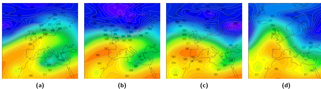
Figura 2.19: altezza di geopotenziale a 500hPa alle 12UTC dell' 1 (2.19a), del 2 (2.19b), del 3 (2.19c) e del 4 (2.19d) gennaio 2015.
