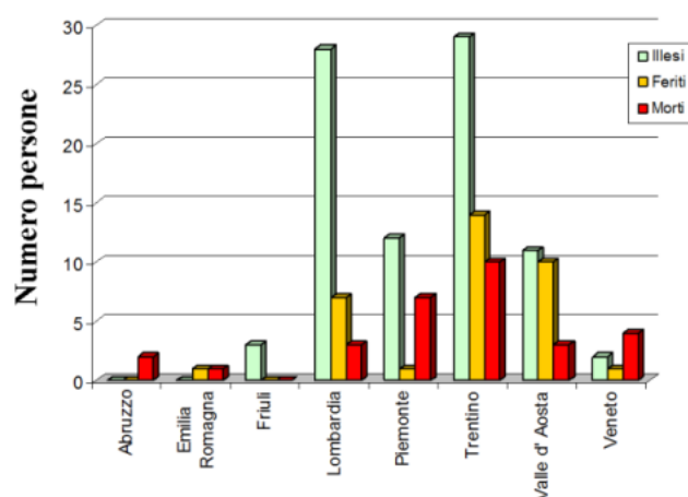
Figura 4.26: distribuzione degli incidenti da valanga sull'arco alpino italiano nella stagione invernale 2014-15.
