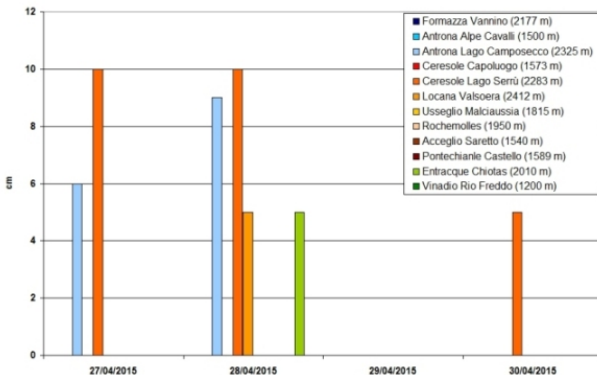
Figura 2.59: altezza della neve fresca giornaliera in alcune stazioni di rilevamento manuale dal 27 al 30 aprile 2015. Con le gradazioni di blu sono indicate le località dei settori nord, con quelle di rosso/arancione/marrone quelle dei settori ovest, mentre con le gradazioni di verde quelle dei settori sud. Le precipitazioni nevose sono misurate dalle ore 8.00 locali e cumulate nelle 24 ore precedenti.
