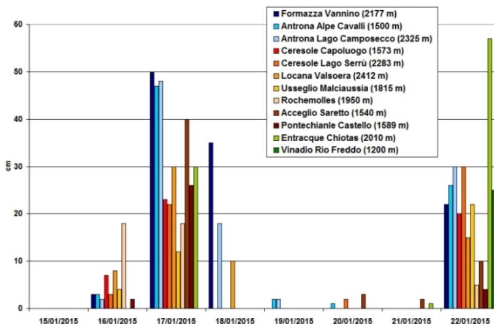
Figura 2.25: altezza della neve fresca giornaliera in alcune stazioni di rilevamento manuale dal 15 al 22 gennaio 2015 . Con le gradazioni di blu sono indicate le località dei settori nord, con quelle di rosso/arancione/marrone quelle dei settori ovest, mentre con le gradazioni di verde quelle dei settori sud. Le precipitazioni nevose sono misurate alle ore 8.00 locali e cumulate nelle 24 ore precedenti.
