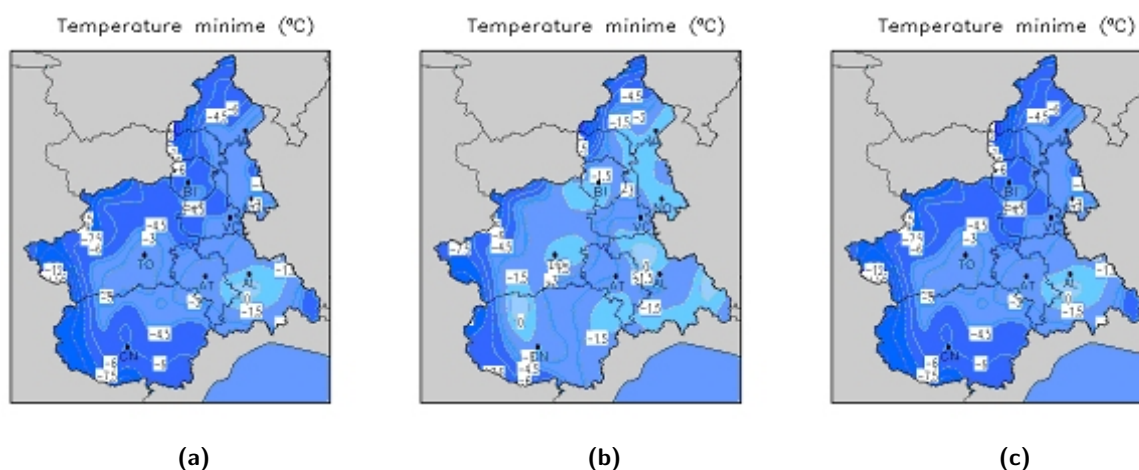
Figura 2.16: temperature minime il 26 (2.16a), 27 (2.16b) e 28 (2.16c) dicembre misurate dalle rete al suolo di Arpa Piemonte.
