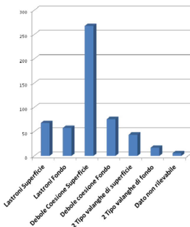
Figura 4.3: tipologia di valanghe osservate con la compilazione del Mod.1 nella stagione 2014-15.
