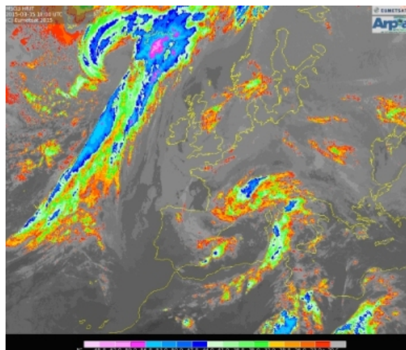
Figura 2.42: immagine da satellite nel canale dell'IR alle ore 18 UTC di domenica 15 marzo .
