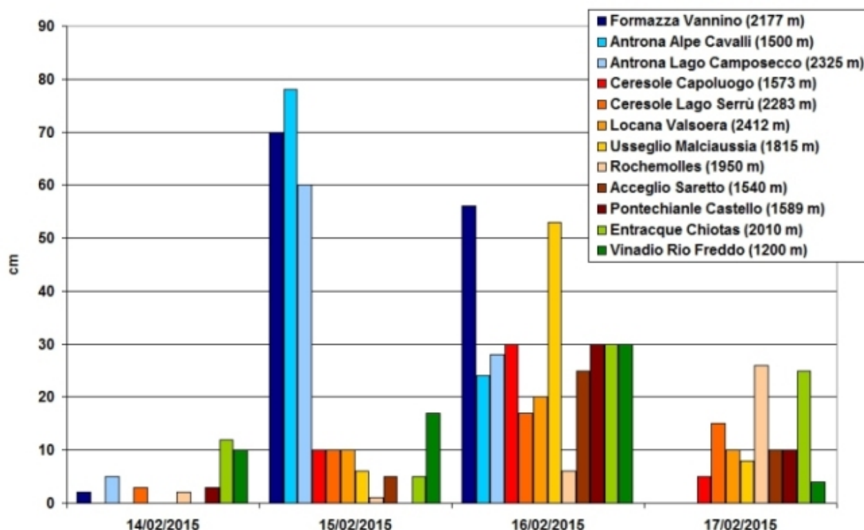
Figura 2.36: altezza della neve fresca giornaliera in alcune stazioni di rilevamento manuale dal 14 al 17 febbraio 2015. Con le gradazioni di blu sono indicate le località dei settori nord, con quelle di rosso/arancione/marrone quelle dei settori ovest, mentre con le gradazioni di verde quelle dei settori sud. Le precipitazioni nevose sono misurate alle ore 8.00 locali e cumulate nelle 24 ore precedenti.
