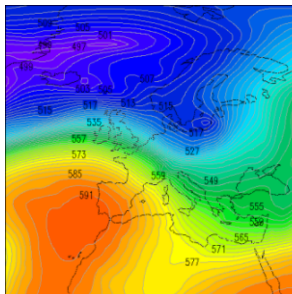
Figura 2.53: analisi dell'altezza di geopotenziale a 500 hPa del 30 marzo alle ore 12 UTC..
