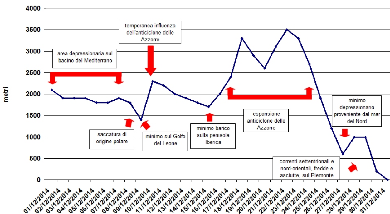
Figura 2.10: andamento dello zero termico nel mese di dicembre 2014 (in blu).
