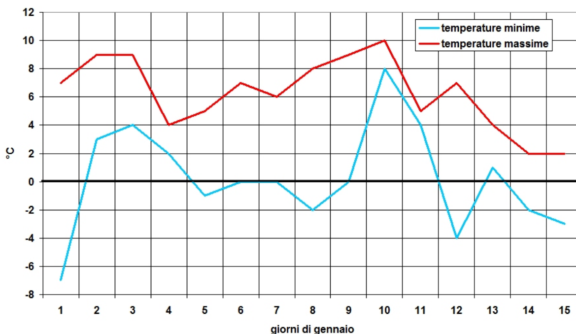
Figura 2.18: andamento medio delle temperature a 2000 m di quota registrate dalle stazioni della rete di Arpa Piemonte nei primi 15 giorni di gennaio .
