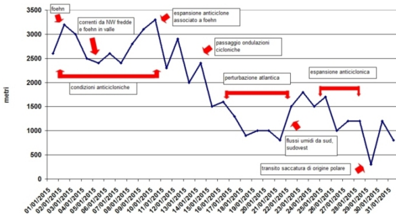
Figura 2.22: andamento dello zero termico nel mese di gennaio 2015 (in blu).
