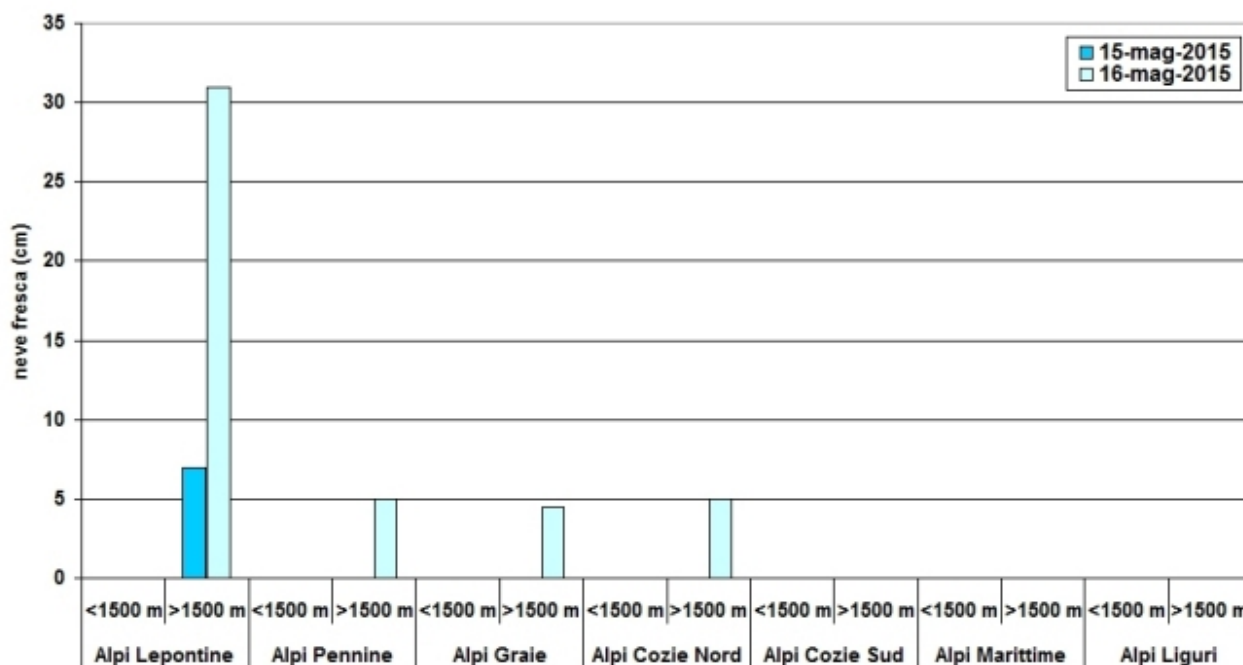
Figura 2.64: istogramma delle precipitazioni nevose per settore dalle stazioni di rilevamento manuale dal 15 al 16 maggio 2015 . Le precipitazioni nevose sono misurate alle ore 8.00 locali e cumulate nelle 24 ore precedenti.
