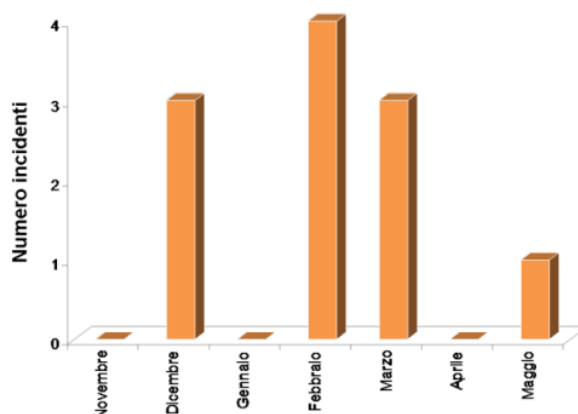
Figura 4.24: distribuzione mensile degli incidenti da valanga nella stagione invernale 2014-15.
