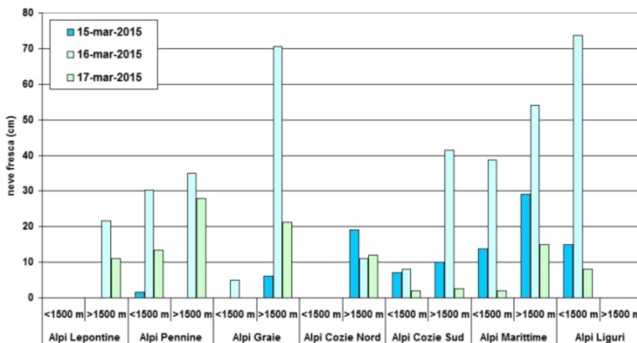
Figura 2.44: istogramma delle precipitazioni nevose per settore dalle stazioni di rilevamento manuale dal 15 al 17 marzo 2015 . Le precipitazioni nevose sono misurate alle ore 8.00 locali e cumulate nelle 24 ore precedenti.
