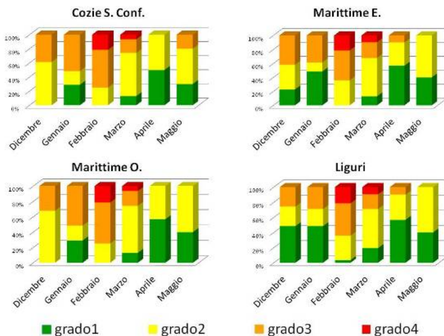
Figura 3.13: andamento dei gradi di pericolo nella settori meridionali da dicembre 2014 a maggio 2015.
