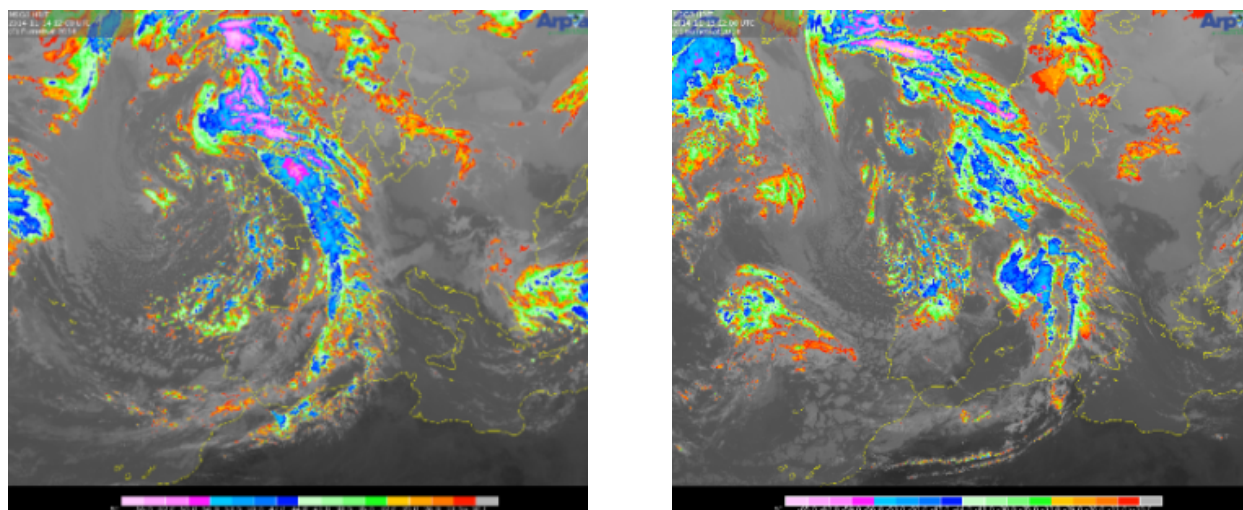
Figura 2.5: immagine satellitare nel canale del visibile dell'IR il 14 novembre (a sinistra) e il 15 novembre (a destra) alle ore 12UTC.
