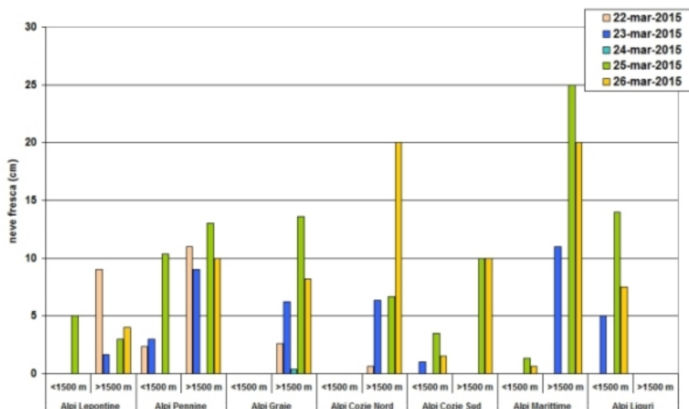
Figura 2.51: istogramma delle precipitazioni nevose per settore dalle stazioni di rilevamento manuale dal 22 al 26 marzo 2015 . Le precipitazioni nevose sono misurate alle ore 8.00 locali e cumulate nelle 24 ore precedenti.
