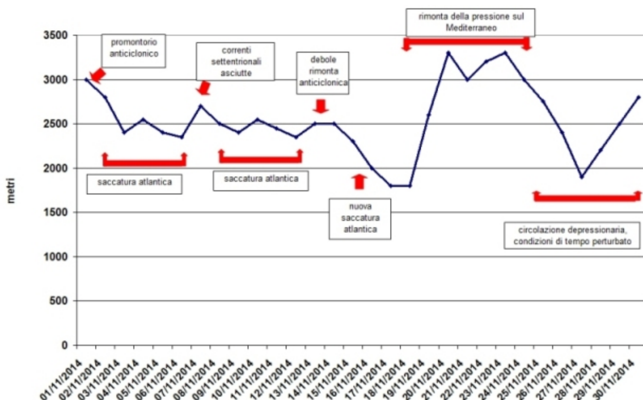
Figura 2.2: andamento dello zero termico nel mese di novembre 2014 (in blu).
