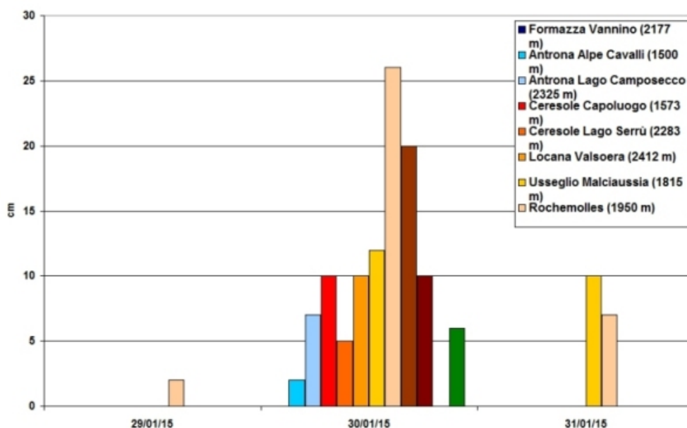
Figura 2.28: altezza della neve fresca giornaliera in alcune stazioni di rilevamento manuale dal 29 al 31 gennaio 2015 . Con le gradazioni di blu sono indicate le località dei settori nord, con quelle di rosso/arancione/marrone quelle dei settori ovest, mentre con le gradazioni di verde quelle dei settori sud. Le precipitazioni nevose sono misurate alle ore 8.00 locali e cumulate nelle 24 ore precedenti.
