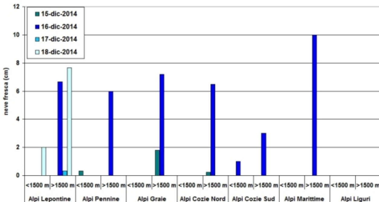
Figura 2.14: istogramma delle precipitazioni nevose per settore nei giorni dal 15 al 18 dicembre 2014 delle stazioni manuali, si osservi come le precipitazioni nevose abbiano interessato il settore nord-occidentale del Piemonte. Le precipitazioni nevose sono misurate alle ore 8.00 locali e cumulate nelle 24 ore precedenti.
