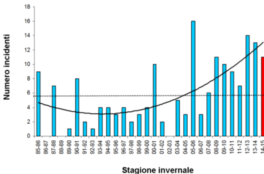
Figura 4.23: frequenza degli incidenti da valanga negli ultimi 30 anni. La linea tratteggiata e la linea intera descrivono rispettivamente la media (5.7 incidenti/anno) e la tendenza polinomiale.
