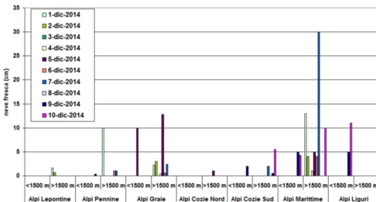
Figura 2.12: istogramma delle precipitazioni nevose per settore nei giorni dall'1 al 10 dicembre 2014 delle stazioni manuali, si osservi come le precipitazioni nevose abbiano interessato il settore nord-occidentale del Piemonte. Le precipitazioni nevose sono misurate alle ore 8.00 locali e cumulate nelle 24 ore precedenti.
