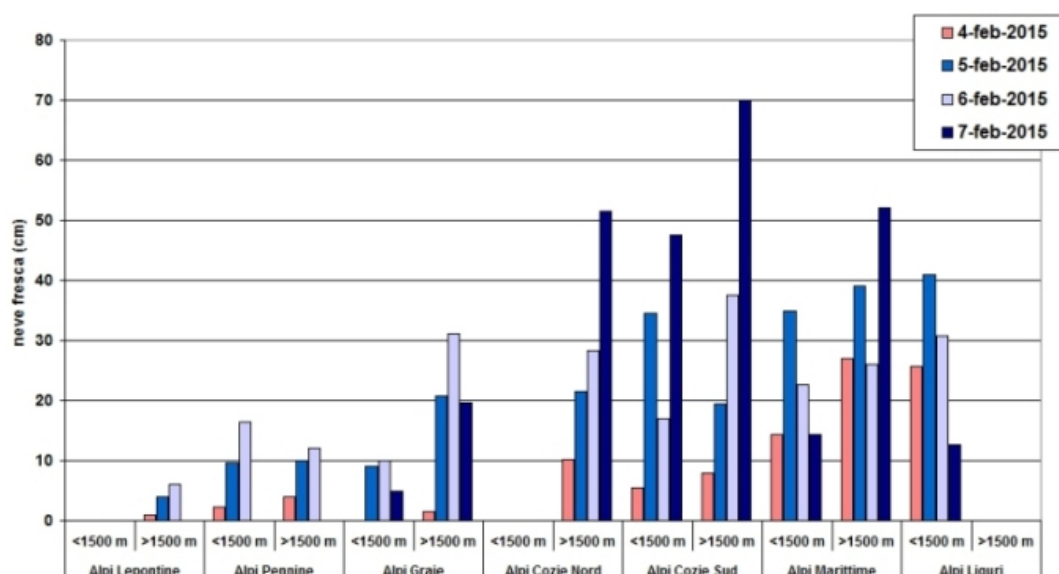
Figura 2.31: istogramma delle precipitazioni nevose per settore dalle stazioni di rilevamento manuale dal 4 al 7 febbraio 2015 . Le precipitazioni nevose sono misurate alle ore 8.00 locali e cumulate nelle 24 ore precedenti.
