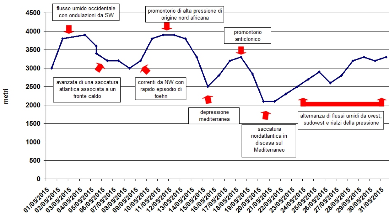
Figura 2.61: andamento dello zero termico nel mese di maggio 2015 (in blu).
