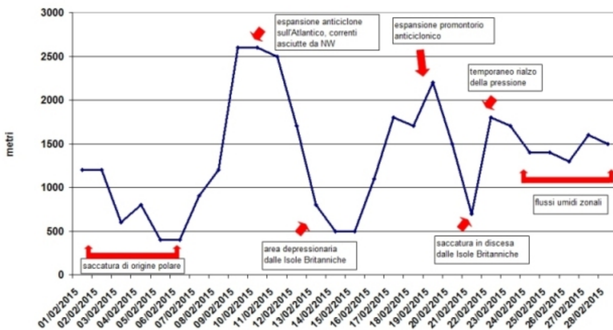
Figura 2.30: andamento dello zero termico nel mese di febbraio 2015 (in blu).
