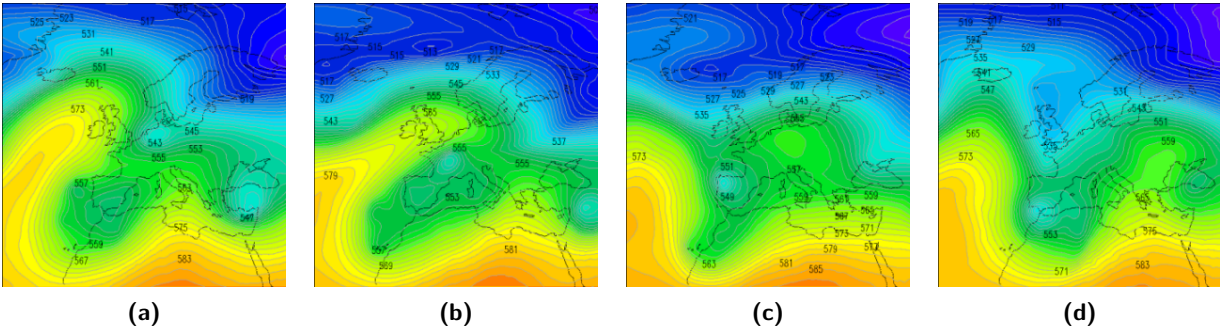
Figura 2.47: altezza di geopotenziale a 500hPa alle ore 12UTC del 21 (2.47a), 22 (2.47b), 23 (2.47c) e 24 (2.47d) marzo 2015 .
