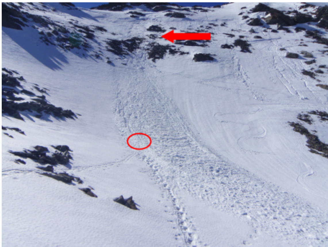
Figura 4.50: valanga di Punta Almiane. La freccia rossa indica il punto del traverso da cui si è propagata la frattura a seguito del passaggio di uno sciatore. Il cerchio indica la posizione in cui è stato trasportato lo sciatore travolto.
