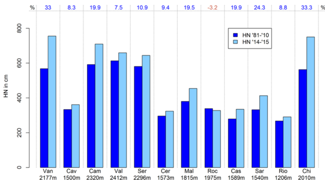
Figura 1.2: neve fresca cumulata da novembre a maggio nella stagione 2014-2015 (in azzurro) a confronto con la media trentennale '81-'10 (in blu).
