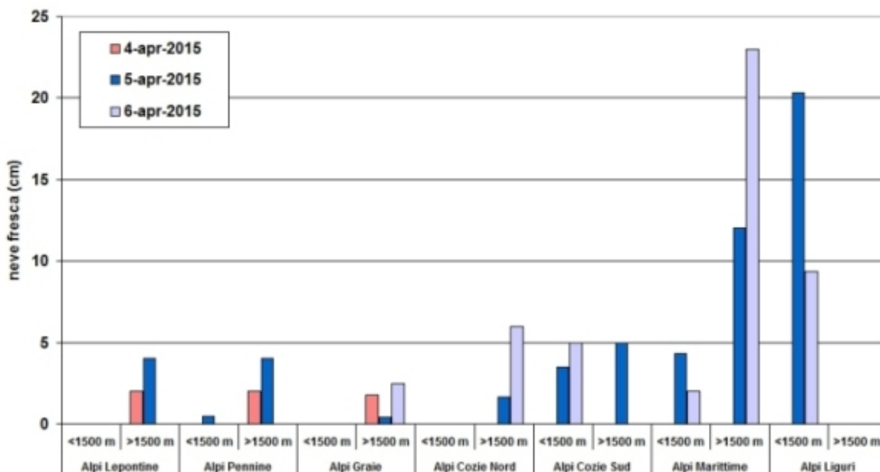
Figura 2.55: istogramma delle precipitazioni nevose per settore dalle stazioni di rilevamento manuale dal 4 al 6 aprile 2015 . Le precipitazioni nevose sono misurate alle ore 8.00 locali e cumulate nelle 24 ore precedenti.
