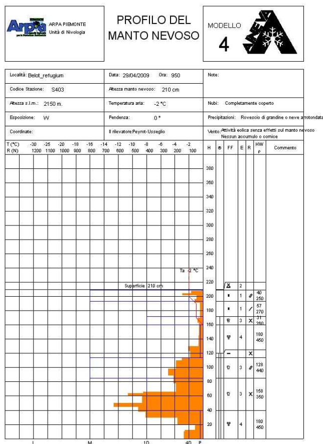
Fig. 5: Stratigrafia del manto nevoso effettuata in Valle Chisone presso il Rifugio Belot (2150 m) nel comune di Pragelato il 29/04/2009
