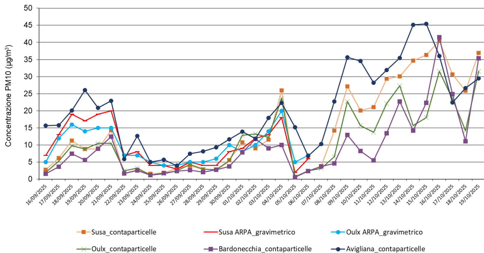
Figura 2 – PM10, valori medi giornalieri – confronto dati Sitaf/dati Arpa
