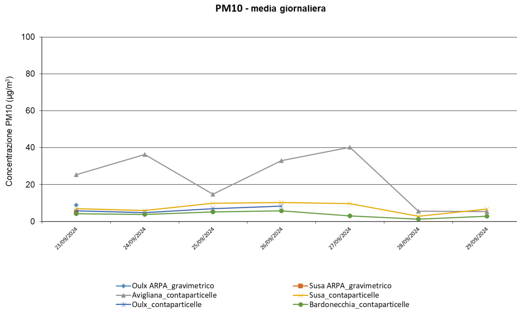
Figura 3 – PM10, valori medi giornalieri – confronto dati Sitaf/dati Arpa
