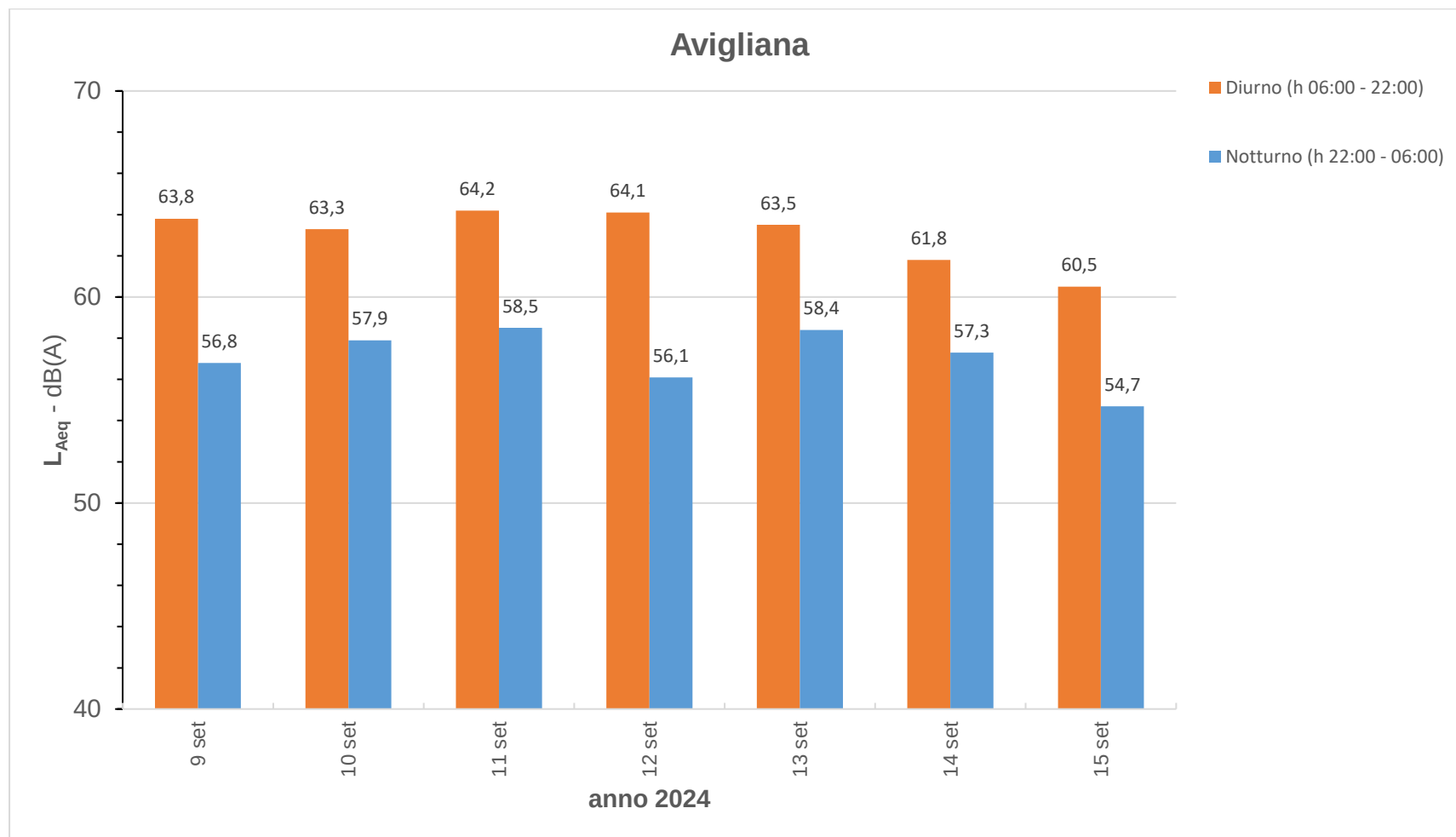
Figura 12 –Andamento dei livelli di rumore su base giornaliera nella postazione di Avigliana
