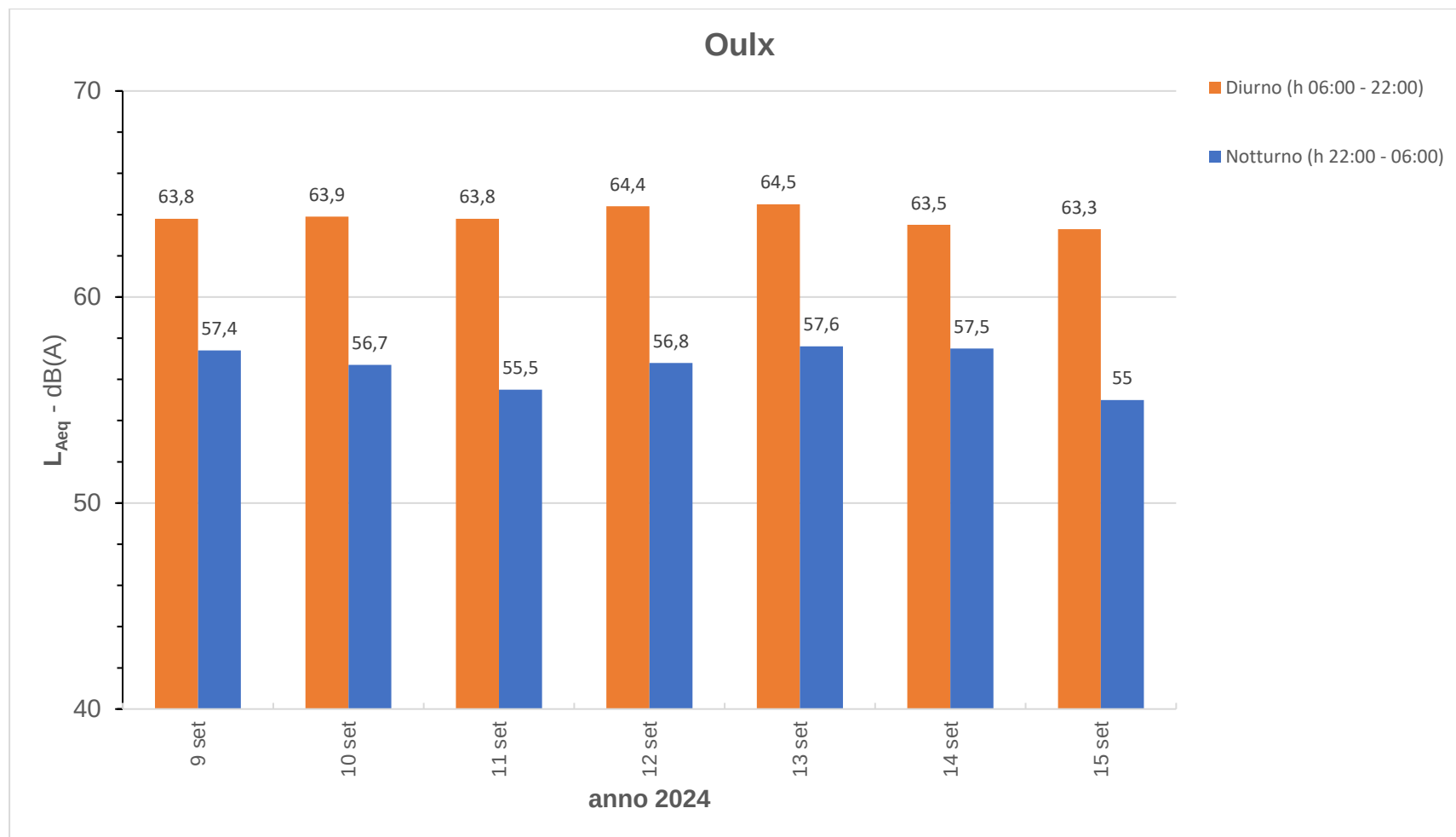
Figura 6 –Andamento dei livelli di rumore su base giornaliera nella postazione di Oulx
