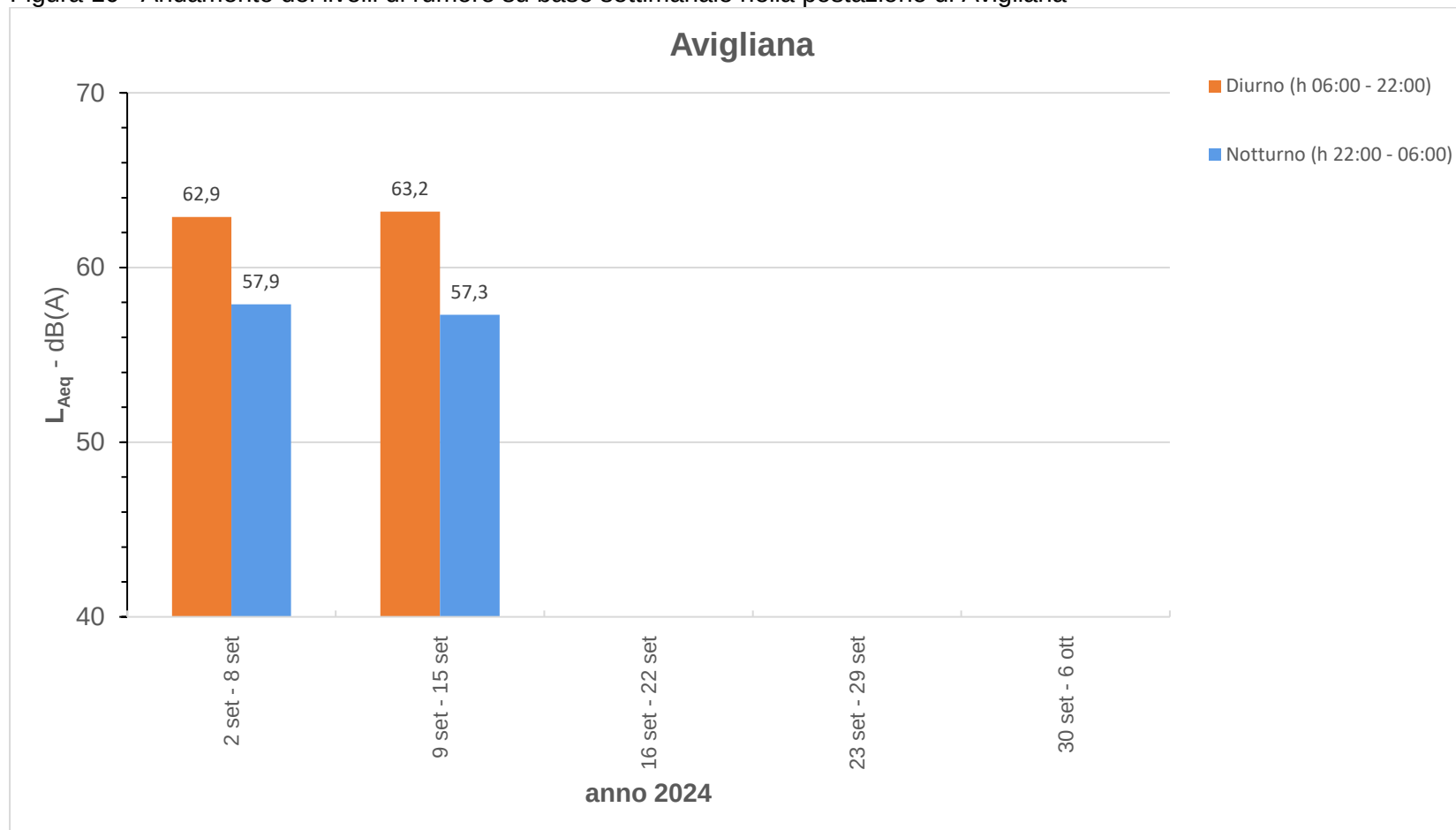
Figura 10 –Andamento dei livelli di rumore su base settimanale nella postazione di Avigliana
