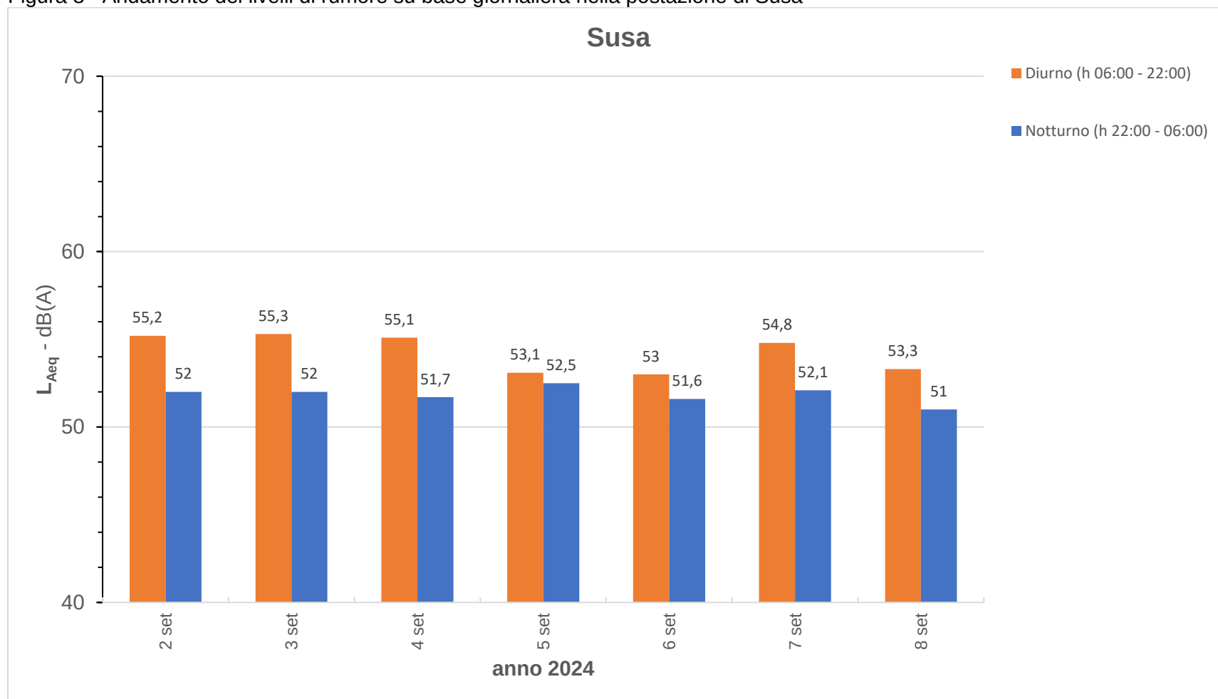
Figura 8 –Andamento dei livelli di rumore su base giornaliera nella postazione di Susa
