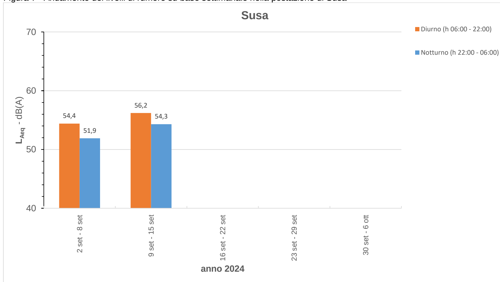
Figura 7 –Andamento dei livelli di rumore su base settimanale nella postazione di Susa
