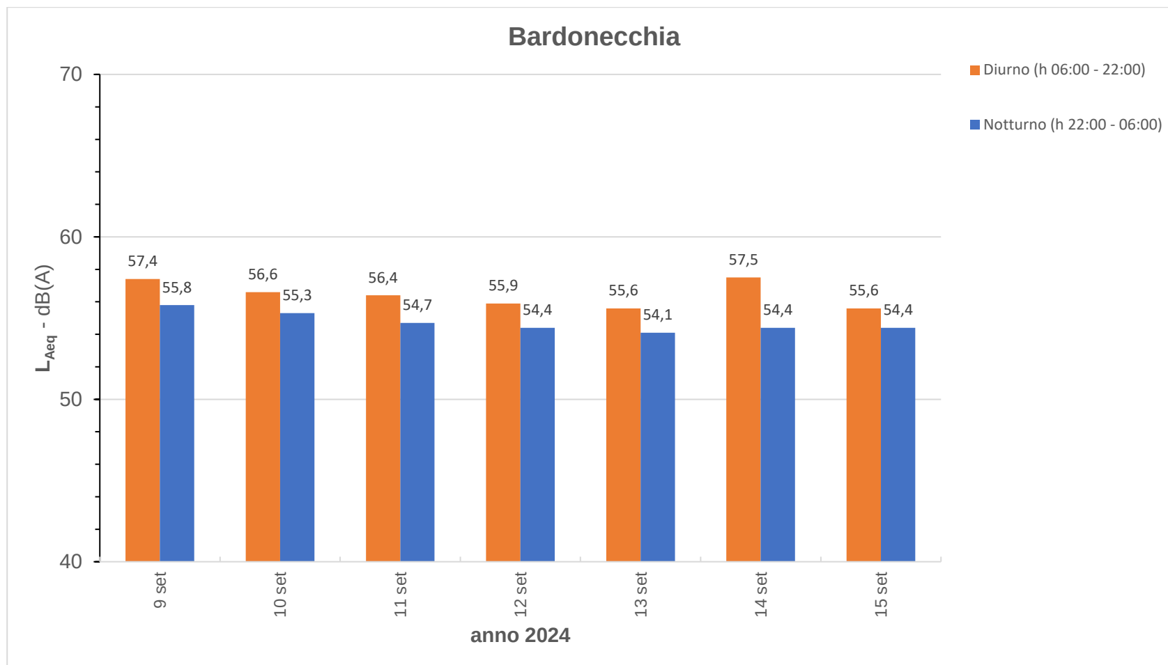
Figura 3 –Andamento dei livelli di rumore su base giornaliera nella postazione di Bardonecchia
