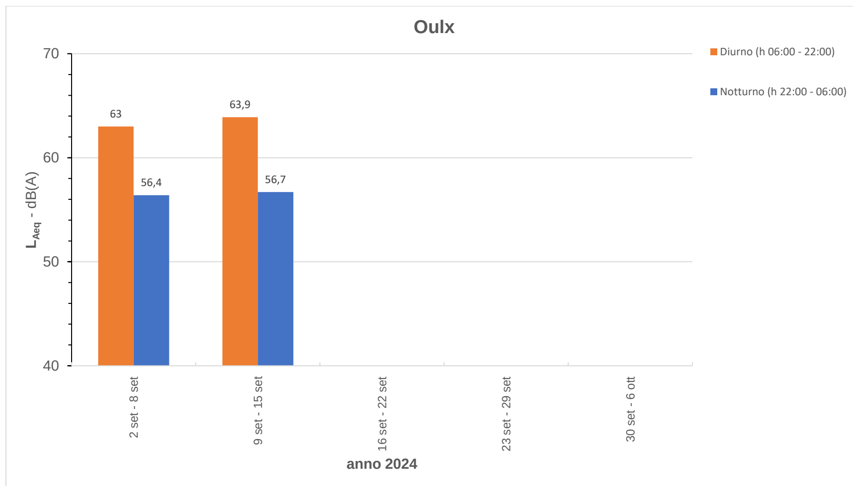
Figura 4 –Andamento dei livelli di rumore su base settimanale nella postazione di Oulx
