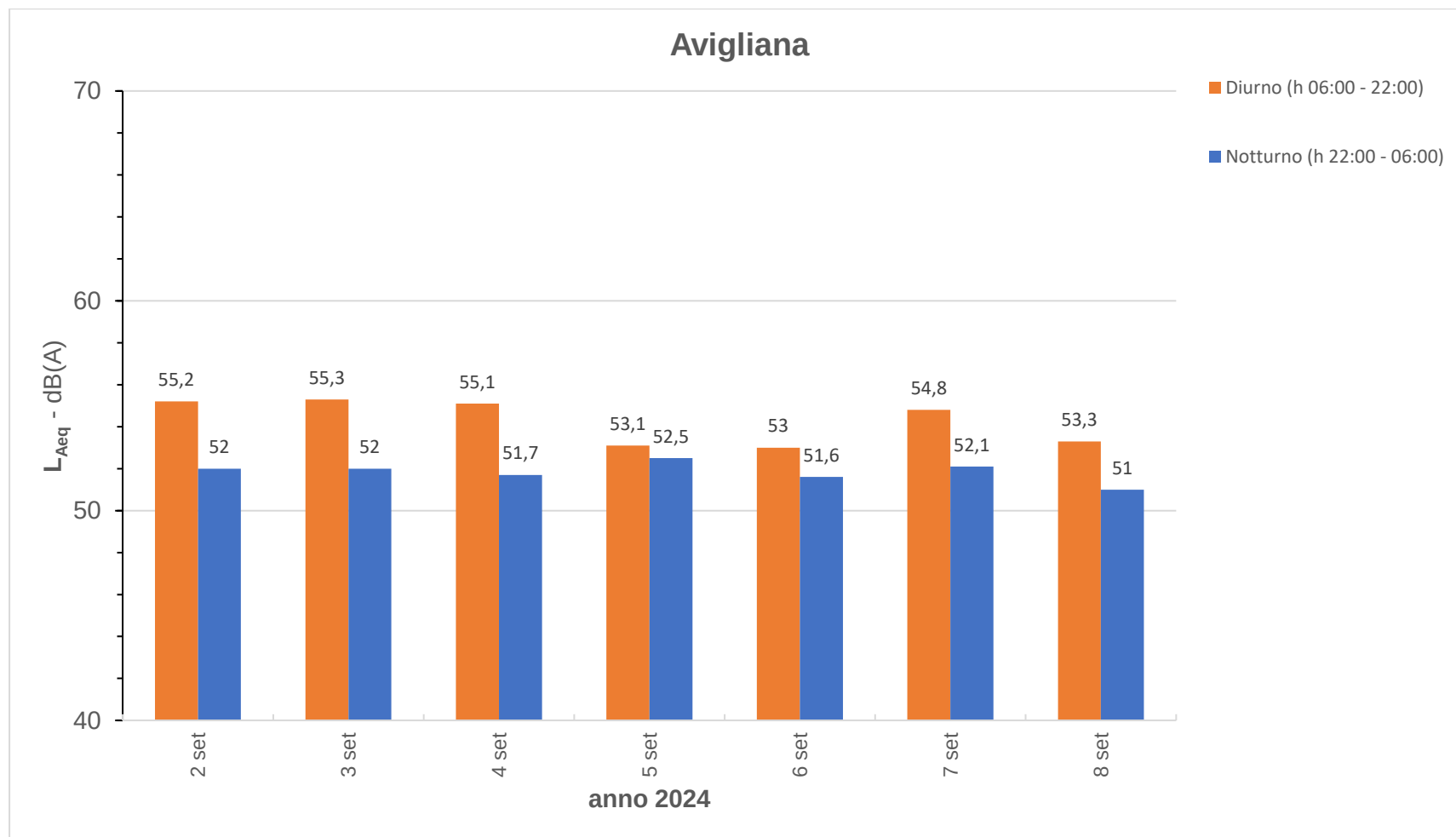
Figura 11 –Andamento dei livelli di rumore su base giornaliera nella postazione di Avigliana
