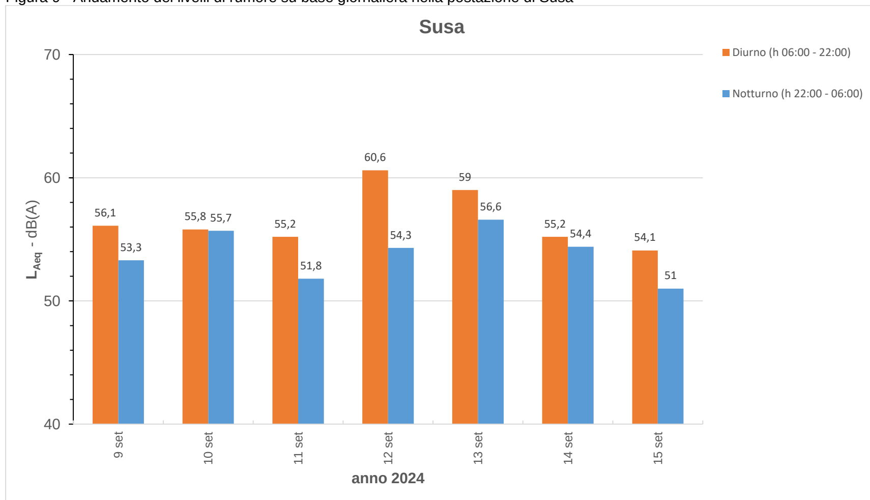
Figura 9 –Andamento dei livelli di rumore su base giornaliera nella postazione di Susa
