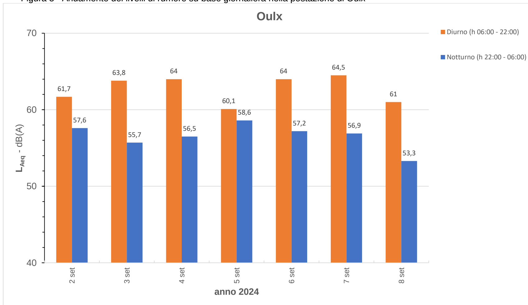
Figura 5 –Andamento dei livelli di rumore su base giornaliera nella postazione di Oulx
