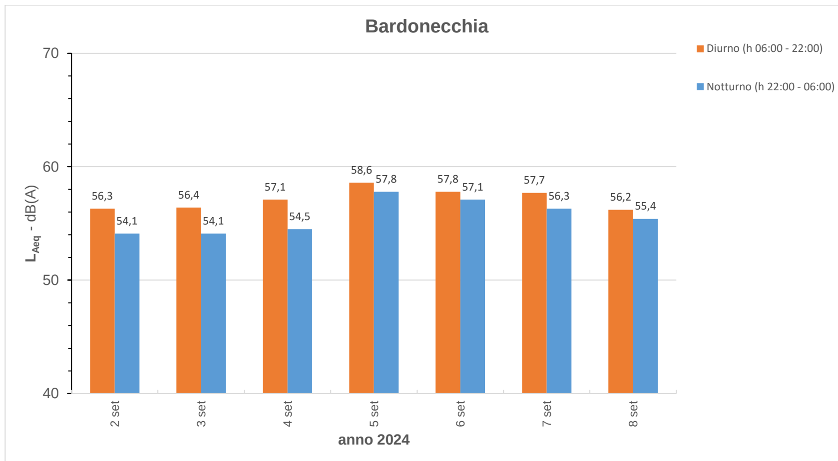
Figura 2 –Andamento dei livelli di rumore su base giornaliera nella postazione di Bardonecchia
