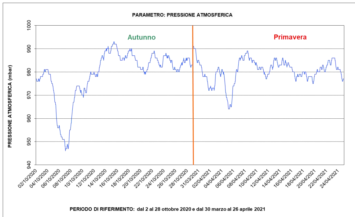
Figura 24: Pressione Atmosferica
