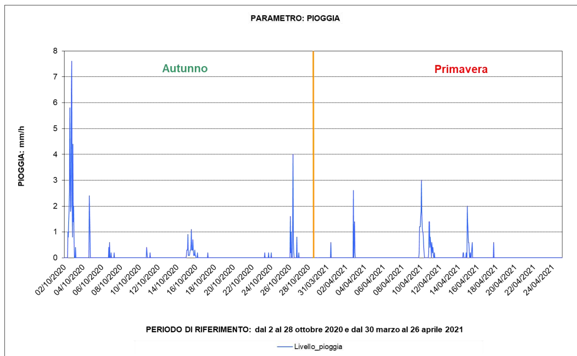
Figura 27: pioggia
