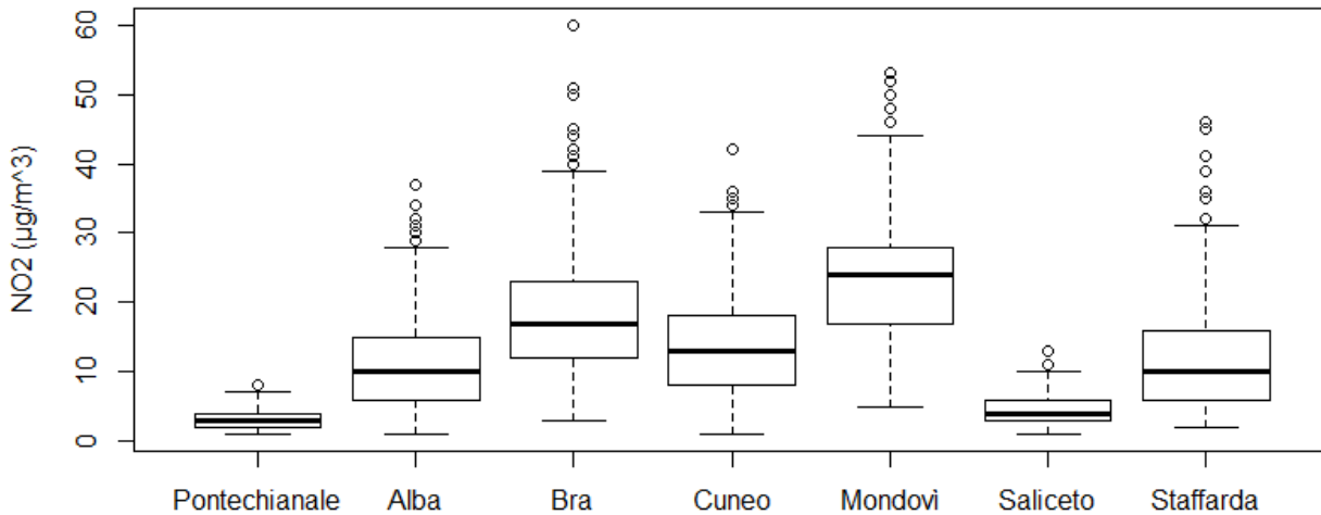
Figura 2) NO 2 : confronto tra le distribuzioni delle concentrazioni orarie rilevate con il laboratorio mobile a Pontechianale e presso le centraline della provincia (periodo 21 maggio ÷ 27 giugno '19)
