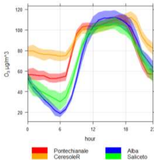
Figura 8) O 3 : giorno medio della campagna di Pontechianale confrontato con quello delle centraline fisse di Ceresole Reale, Alba e Saliceto (periodo: 21 maggio ÷ 27 giugno '19).
