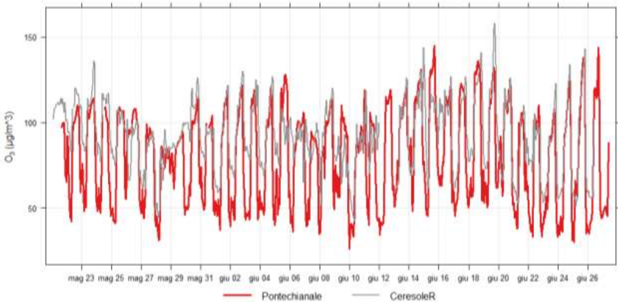
Figura 7) O 3 : concentrazioni orarie rilevate nei siti di Pontechianale e Ceresole Reale.
