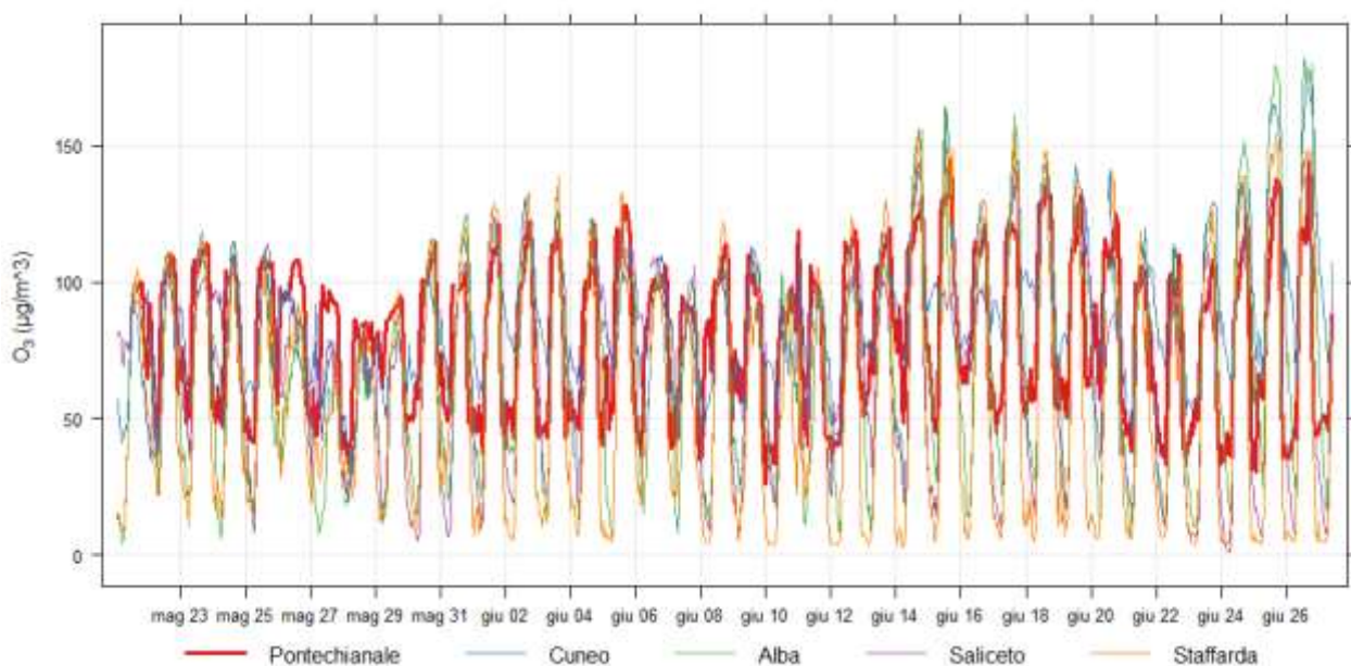
Figura 6) O 3 : concentrazioni orarie rilevate dal laboratorio mobile nel sito di Pontechianale e presso le centraline della provincia di Cuneo.
