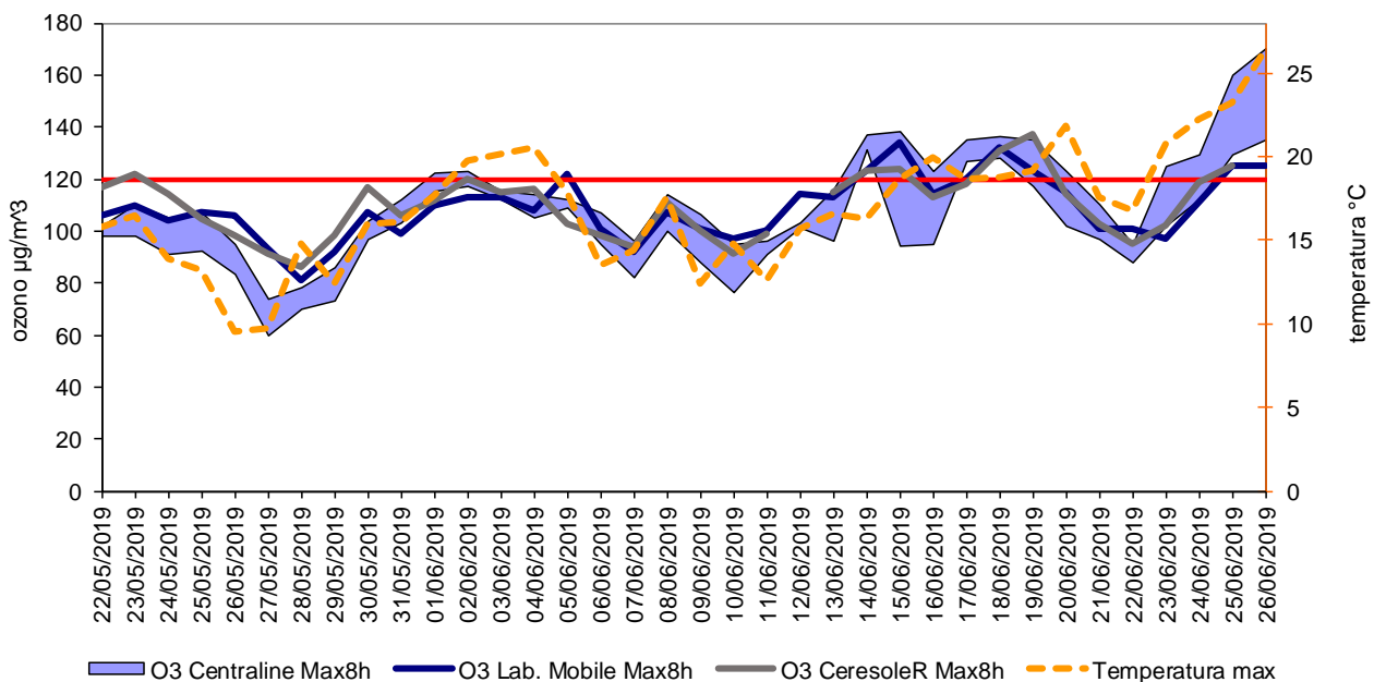
Figura 10) O 3 : massime giornaliere delle concentrazioni medie su 8 ore registrate con il laboratorio mobile a Pontechianale e presso le centraline fisse della provincia di Cuneo. Temperatura massima giornaliera misurata dal laboratorio mobile.
