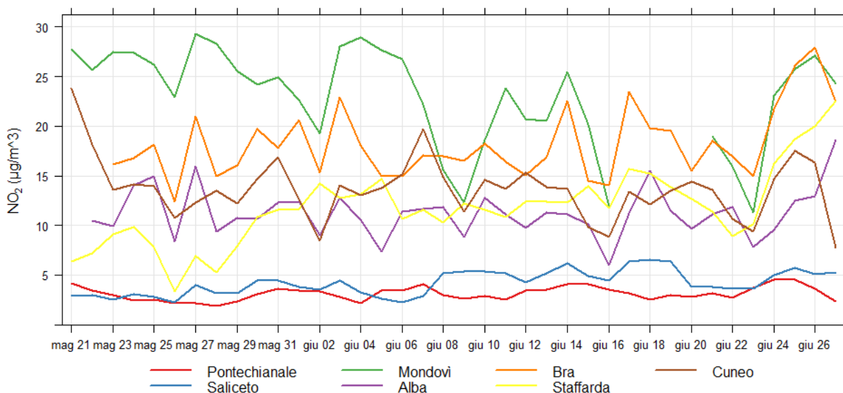
Figura 1) NO 2 : concentrazioni medie giornaliere rilevate dal laboratorio mobile nel sito di Pontechianale e presso le centraline della provincia di Cuneo.
