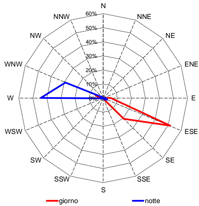
Figura 14) Rosa dei venti a Pontechianale – località Maddalena (periodo: 21 maggio ÷ 27 giugno '19).
