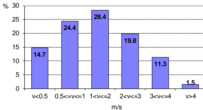
Figura 13) Frequenze di accadimento delle classi di velocità del vento a Pontechianale – località Maddalena (periodo: 21 maggio ÷ 27 giugno '19).
