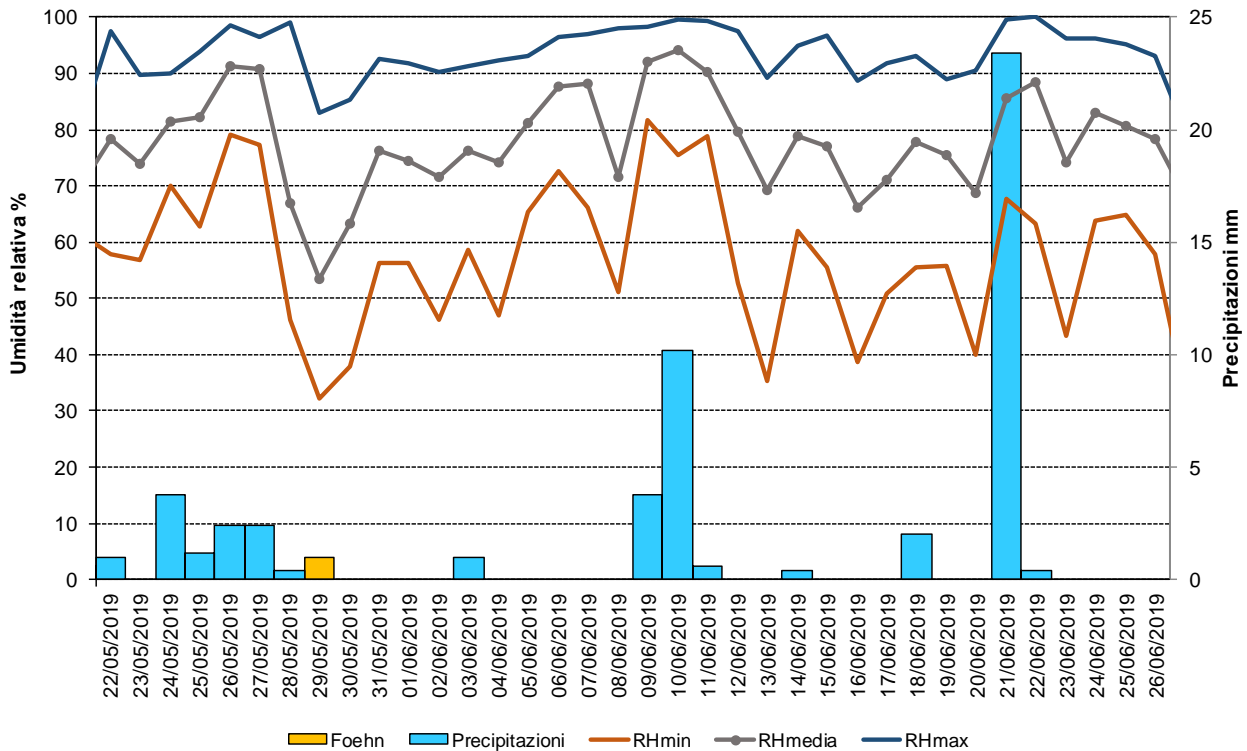
Figura 12) Umidità relativa dell'aria: medie, minime e massime giornaliere registrate con il laboratorio mobile a Pontechianale; precipitazione cumulata giornaliera misurata dalla stazione meteo Pontechianale-Castello; giorni di Foehn sul territorio regionale.
