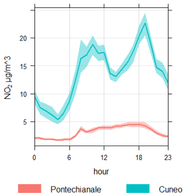
Figura 3) NO 2 : giorno medio della campagna di monitoraggio di Pontechianale confrontato con quello della centralina fissa di Cuneo (periodo 21 maggio ÷ 27 giugno '19).
