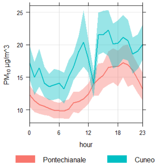
Figura 5) PM 10 : confronto dei giorni medi del sito di Pontechianale e della stazione di Cuneo-Alpini.
