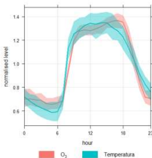
Figura 9) Confronto tra i giorni medi dell'O 3 e della temperatura misurati a Pontechianale su scala normalizzata (periodo: 21 maggio ÷ 27 giugno '19).
