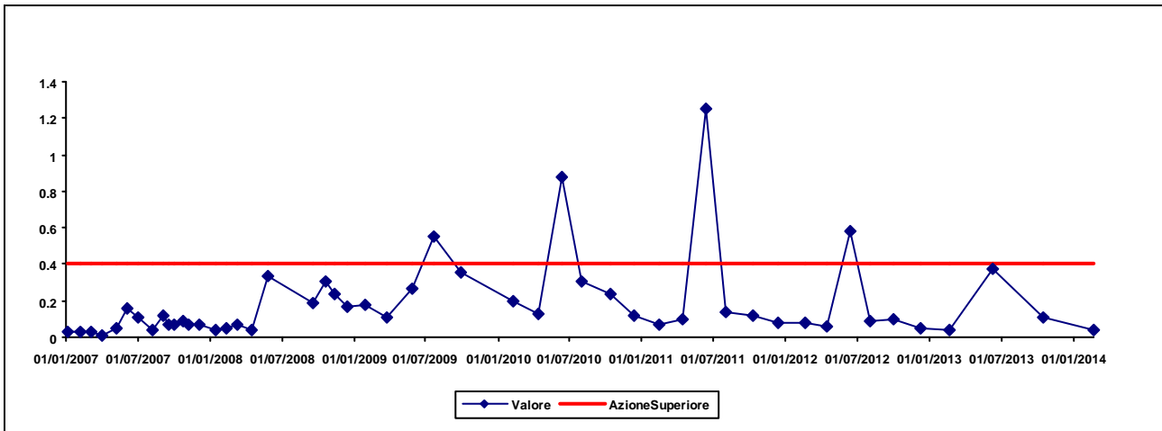
Figura 5.6 Andamento della concentrazione di Sr-90 nell'acqua di falda superficiale prelevata nel punto SPB (Bq/l).
