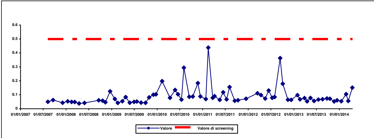
Figura 5.5 Andamento della concentrazione Beta totale nell'acqua di falda superficiale prelevata nel punto S4.1/7 (Bq/l).
