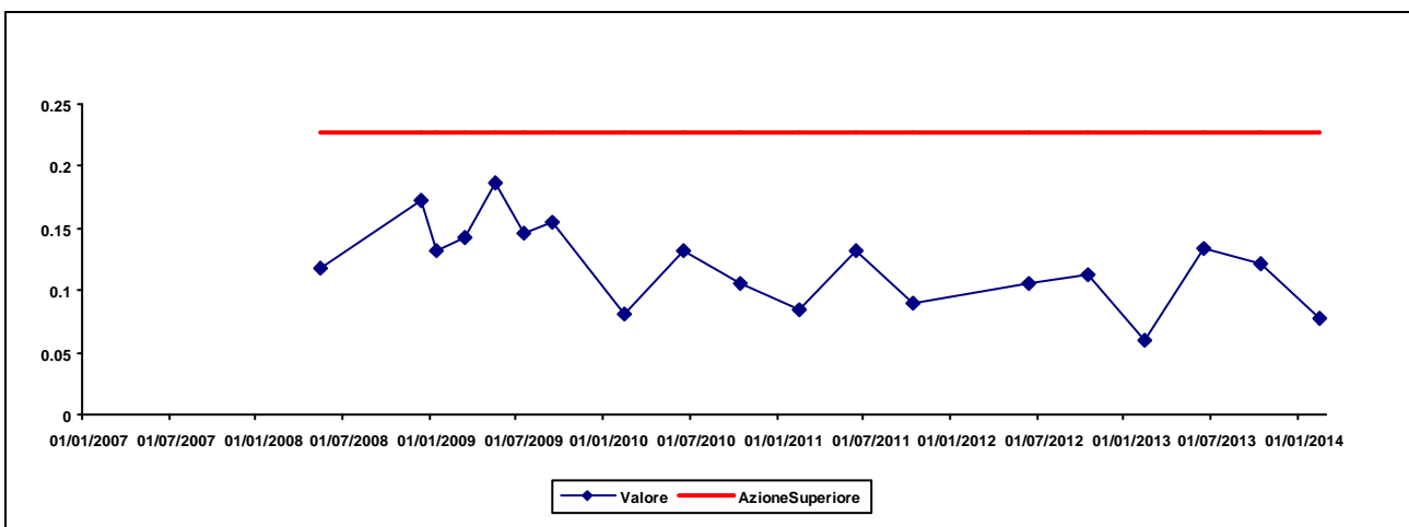
Figura 5.9 Andamento della concentrazione di Sr-90 nell'acqua di falda superficiale prelevata nel punto A5 (Bq/l).
