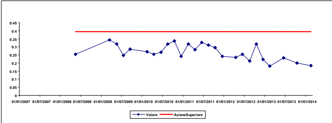
Figura 5.11 Andamento della concentrazione di Sr-90 nell'acqua di falda superficiale prelevata nel punto RP4/7 (Bq/l).
