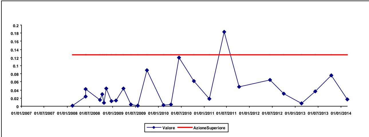
Figura 5.8 Andamento della concentrazione di Cs-137 nell'acqua di falda superficiale prelevata nel punto E5/6 (Bq/l)
