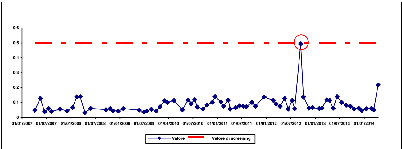
Figura 5.2 Andamento della concentrazione Beta totale nell'acqua potabile prelevata nel punto SQ05 (Bq/l).
