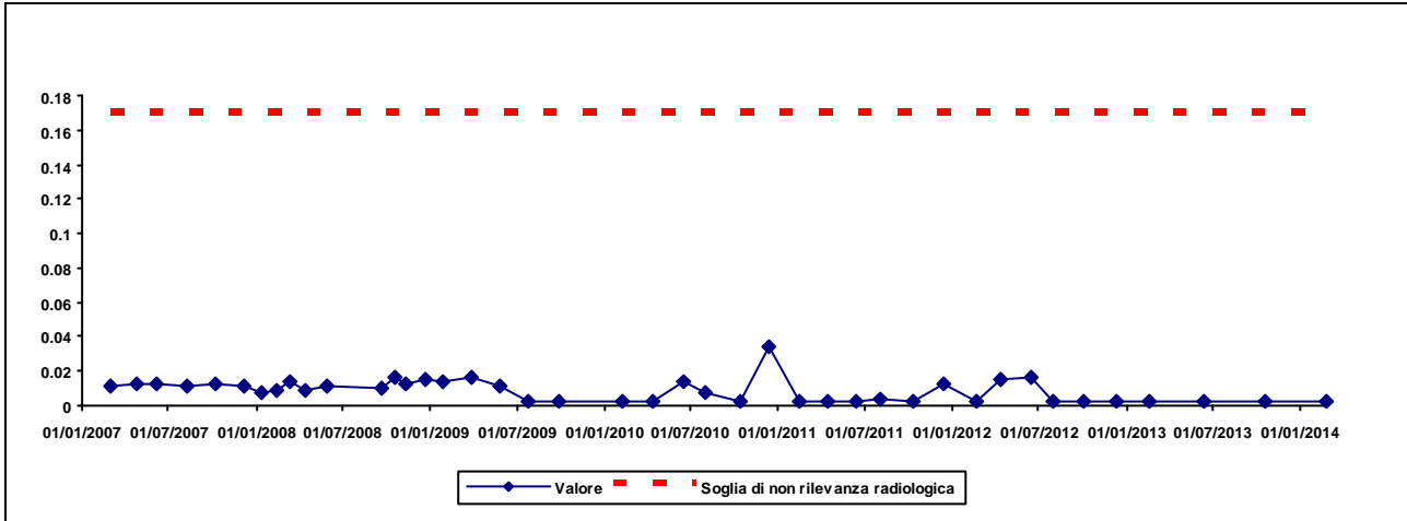
Figura 5.3 Andamento della concentrazione di Sr-90 nell'acqua di falda superficiale prelevata nel punto SP01 (Bq/l).
