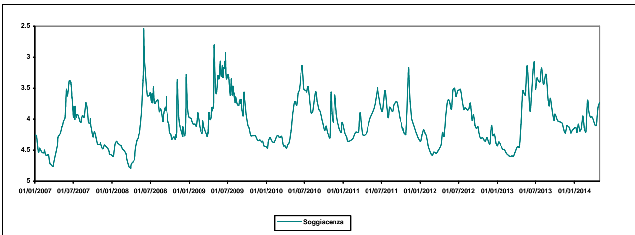
Figura 5.7 Andamento della soggiacenza della falda superficiale nel punto SPB (m.p.c.).
