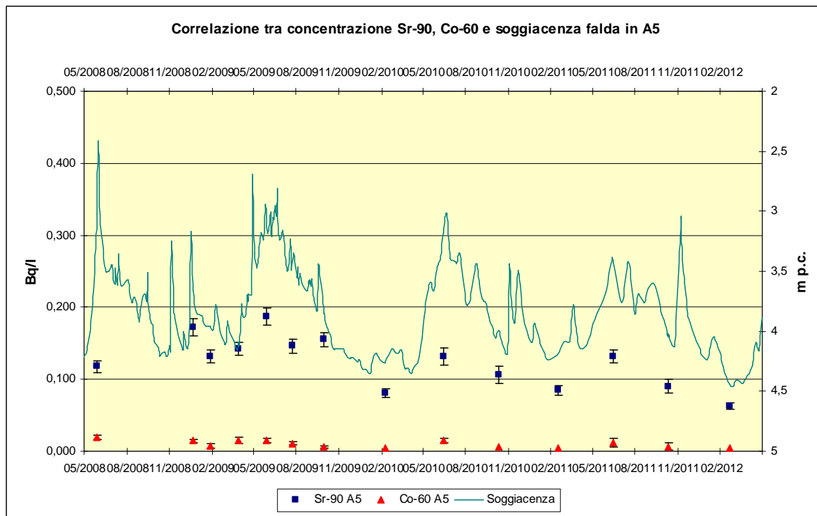
Grafico 5.3 Correlazione tra concentrazione di Sr-90, Co-60 e soggiacenza della falda nel pozzo A5.
