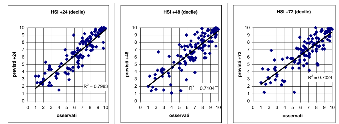
Figura 3.17- Correlazione tra HSI previsto ed osservato. L'HSI viene utilizzato per il calcolo dei livelli di attenzione e che considera la temperatura massima e minima, la copertura nuvolosa e la climatologia.
