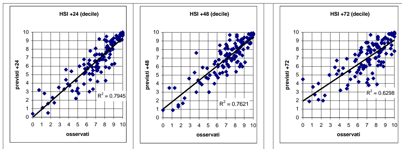
Figura 3.12- Correlazione tra HSI previsto ed osservato. L'HSI viene utilizzato per il calcolo dei livelli di attenzione e che considera la temperatura massima e minima, la copertura nuvolosa e la climatologia.
