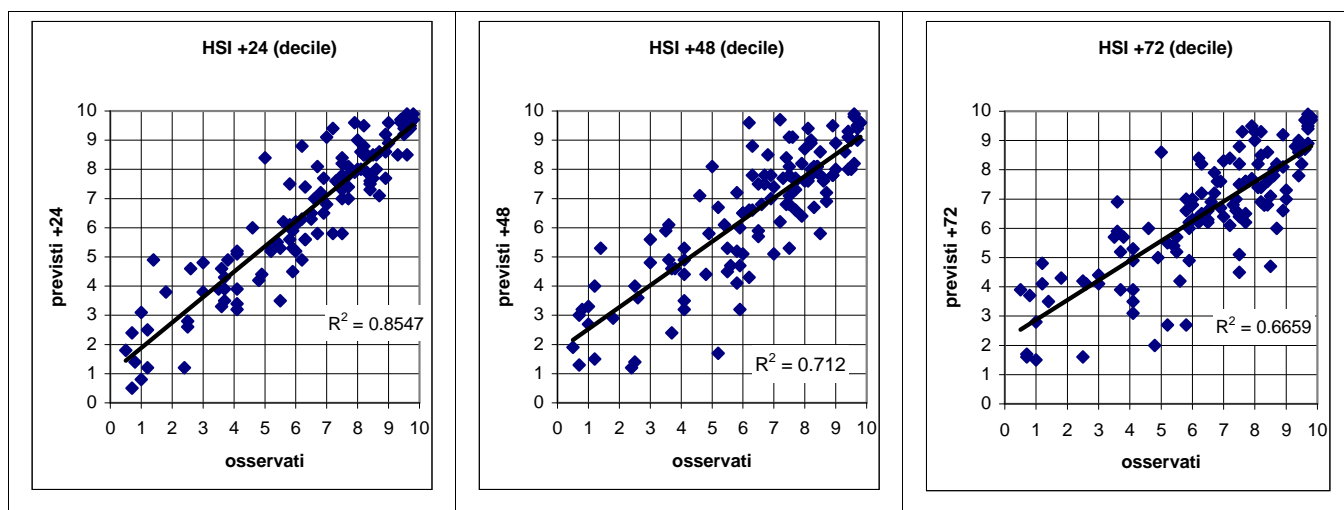
Figura 3.27- Correlazione tra HSI previsto ed osservato. L'HSI viene utilizzato per il calcolo dei livelli di attenzione e che considera la temperatura massima e minima, la copertura nuvolosa e la climatologia.
