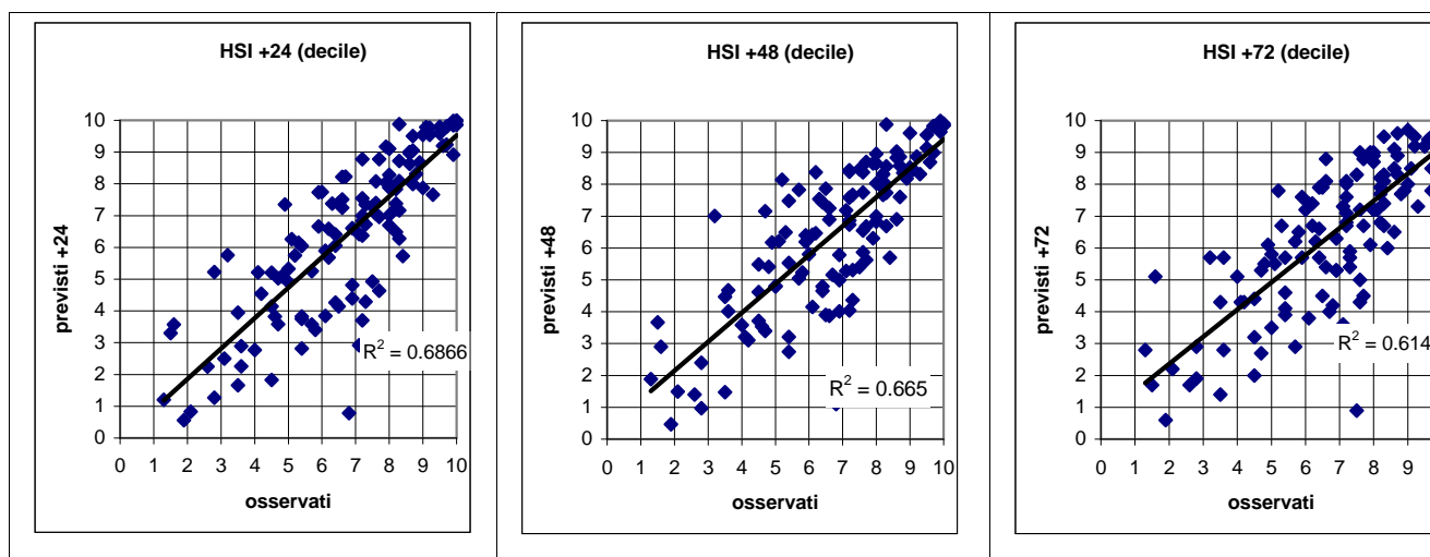
Figura 3.32- Correlazione tra HSI previsto ed osservato. L'HSI viene utilizzato per il calcolo dei livelli di attenzione e che considera la temperatura massima e minima, la copertura nuvolosa e la climatologia.
